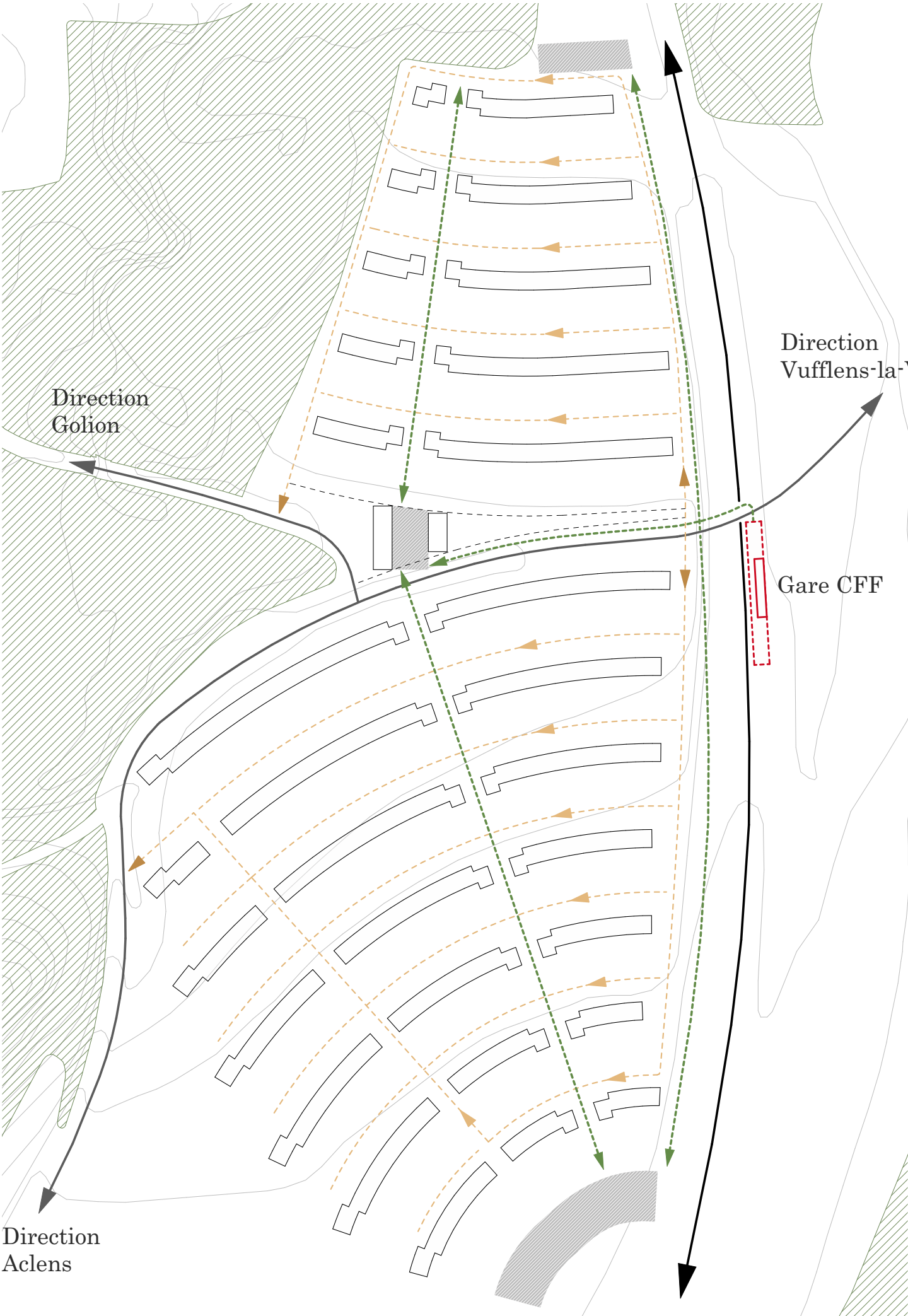
Schéma axes principaux, éléments caractéristiques 1:2'000
