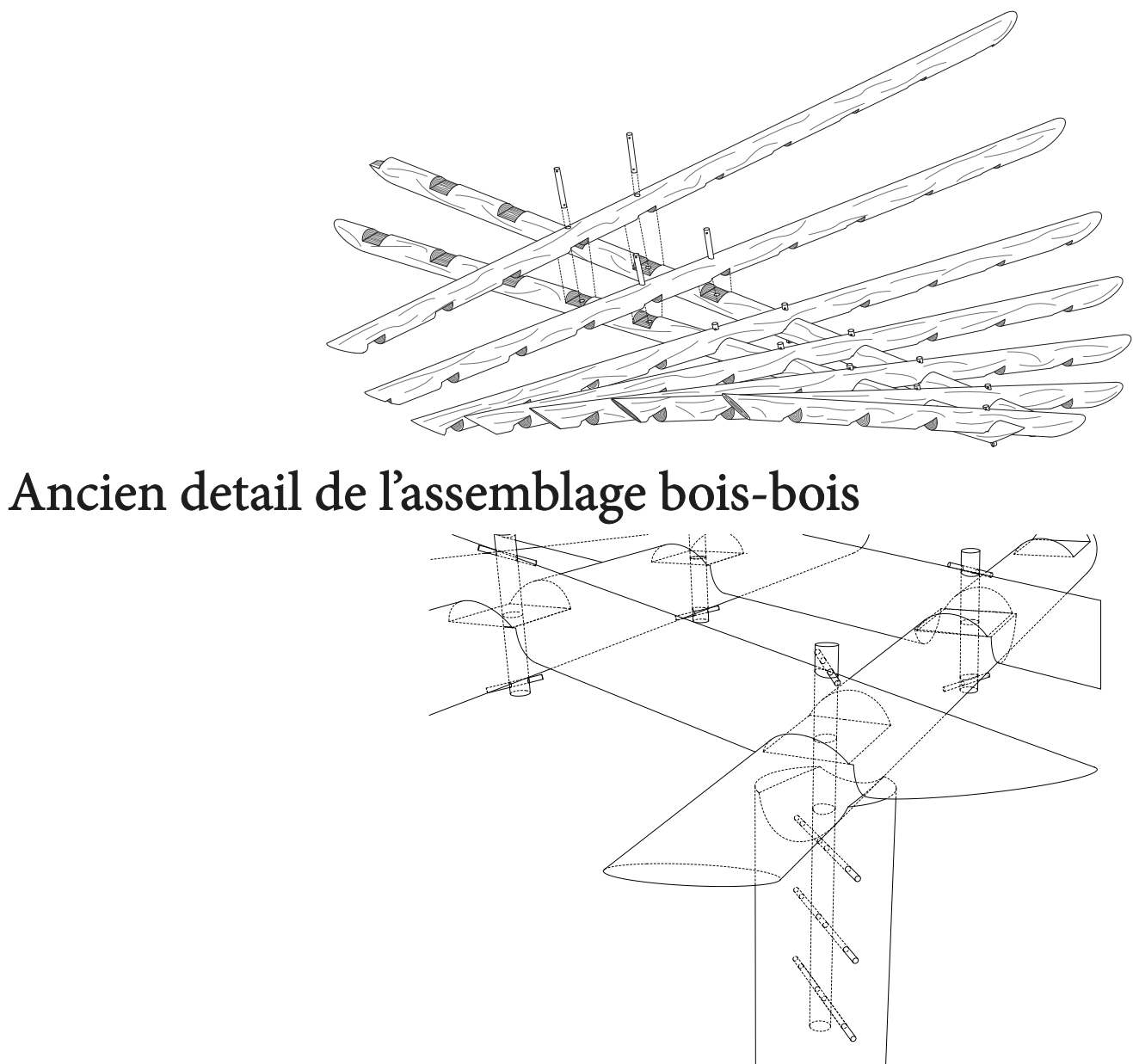
Ancien detail de l'assemblage bois-bois avec le pilier
