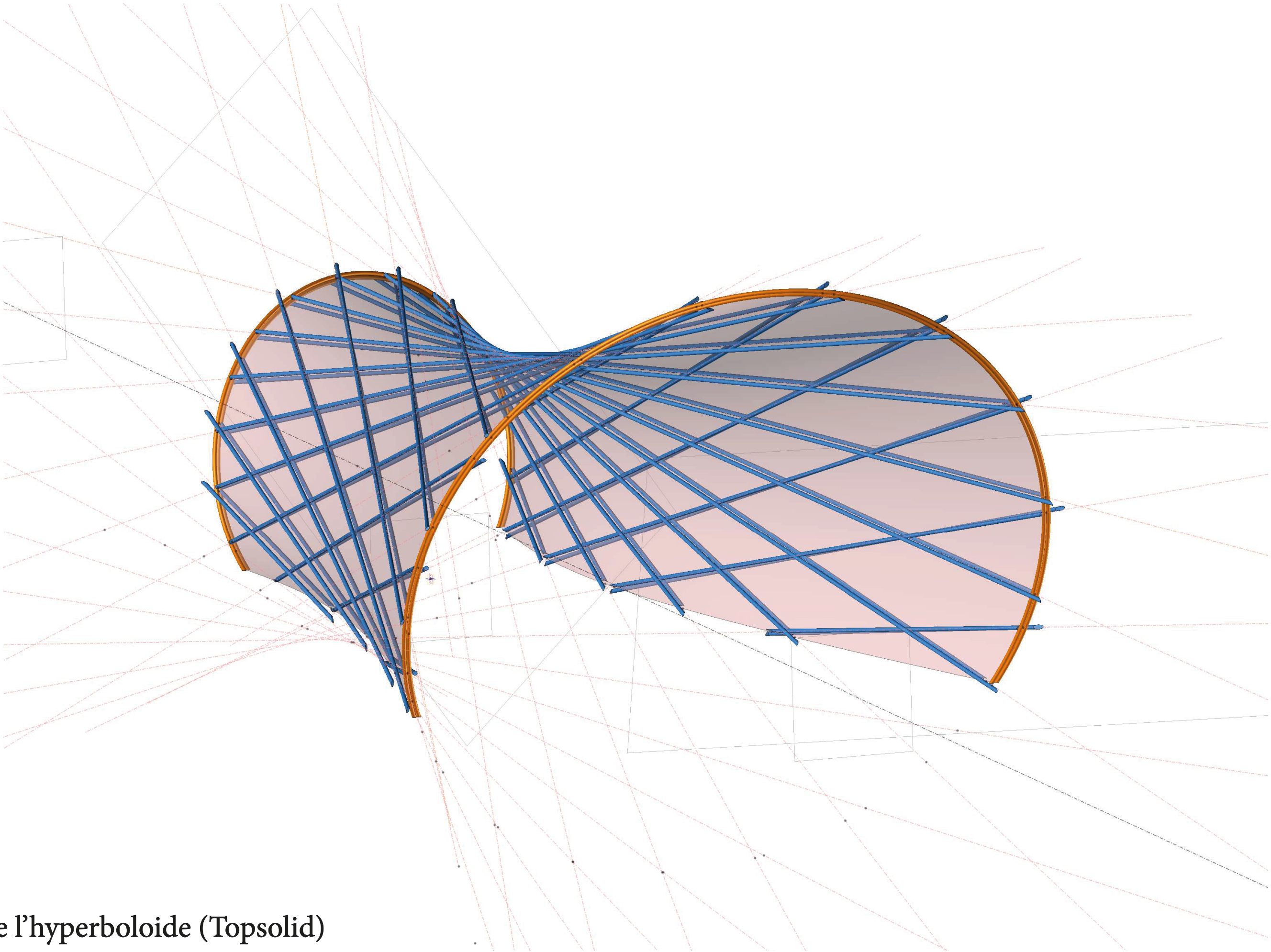
Recherche de l'hyperboloïde (Topsolid)
