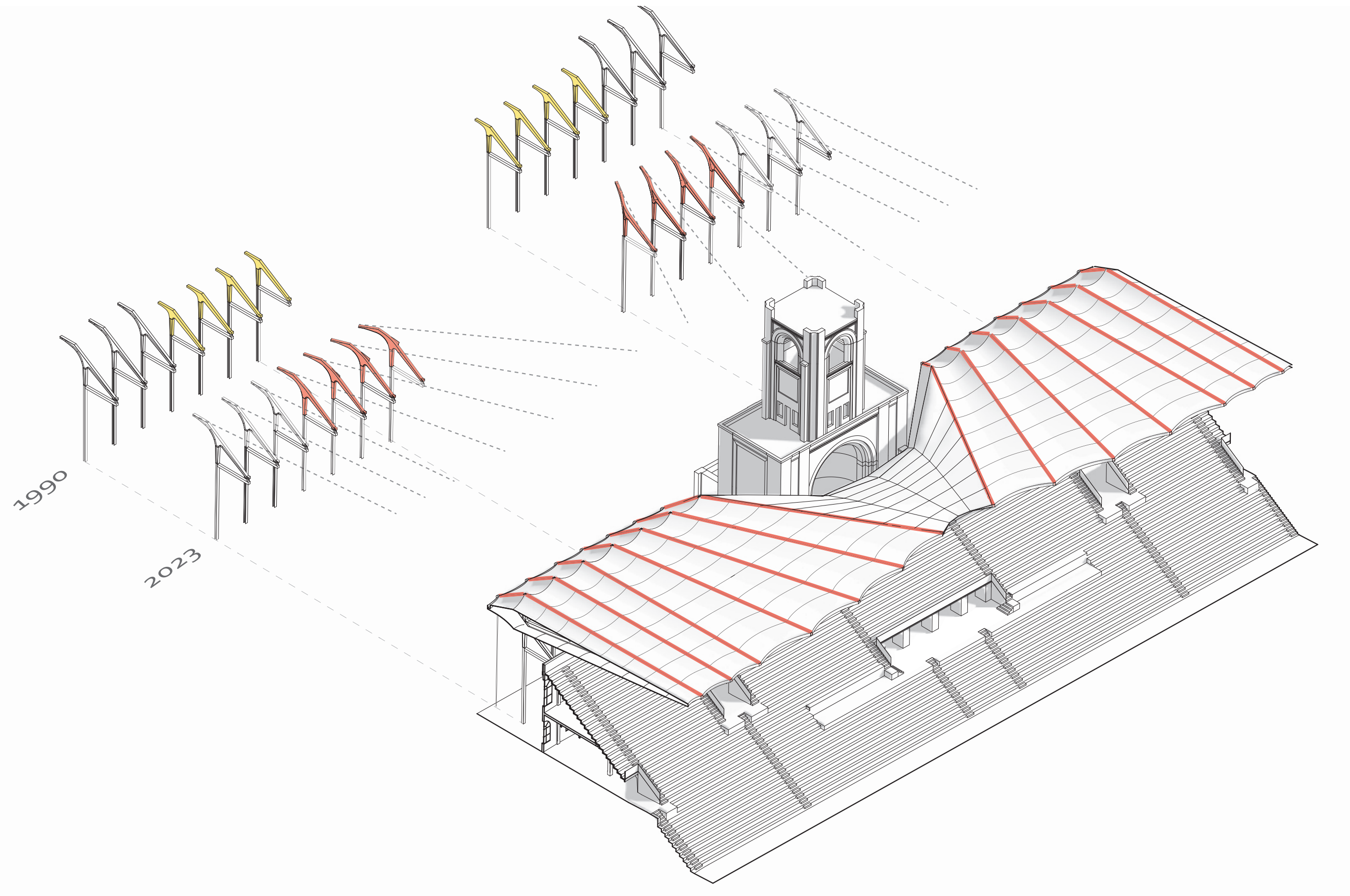
Influence de la tour sur la structure
