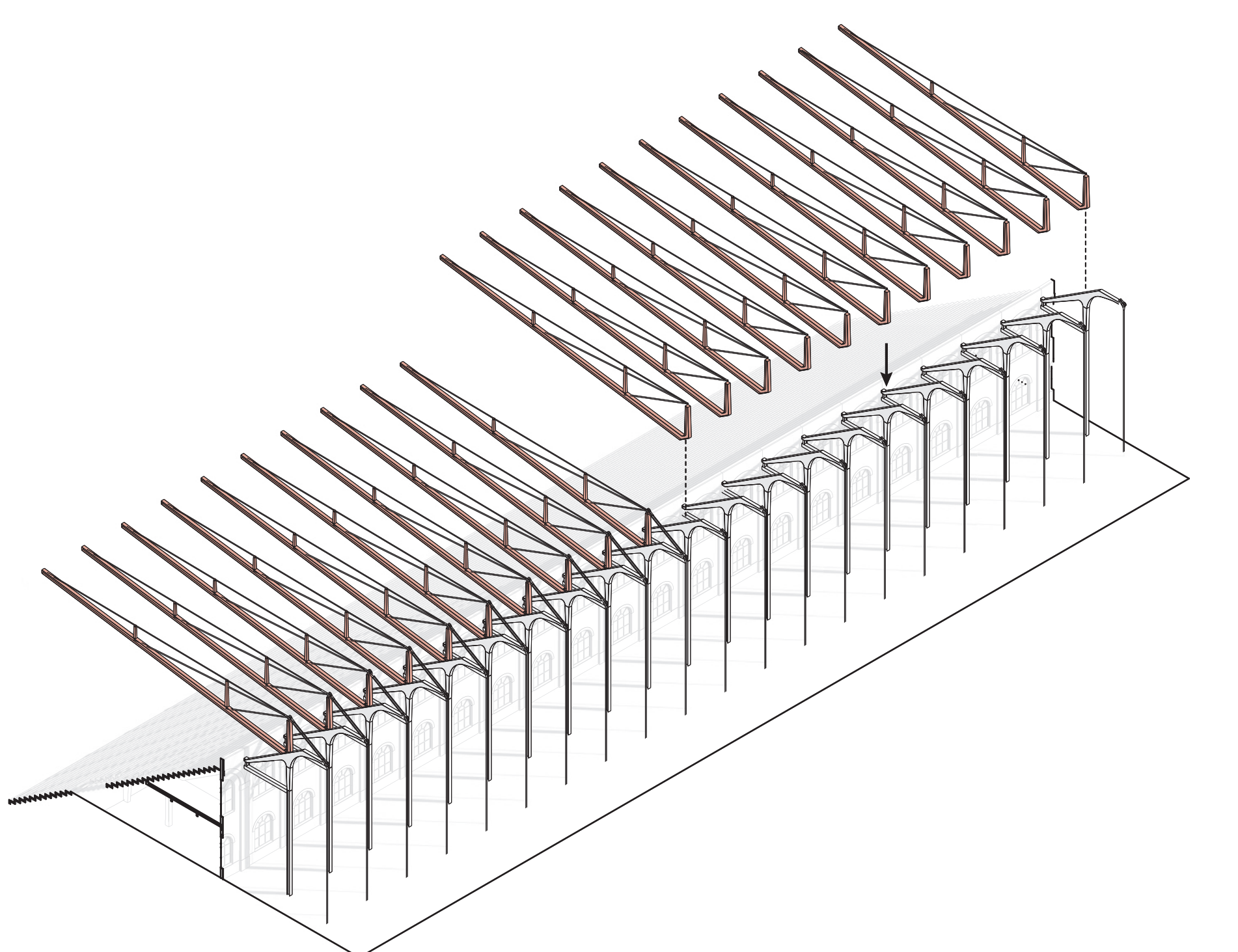
Influence de la tour sur la structure
