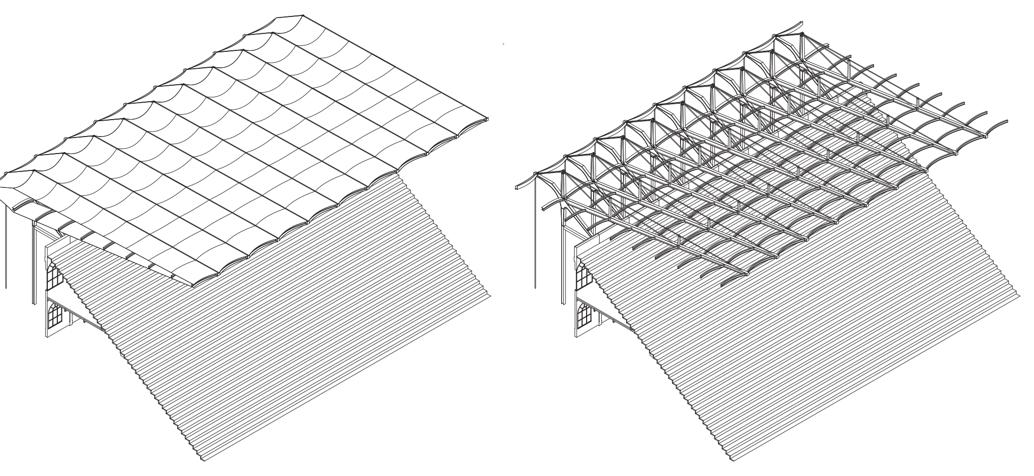
Composition de la toiture
