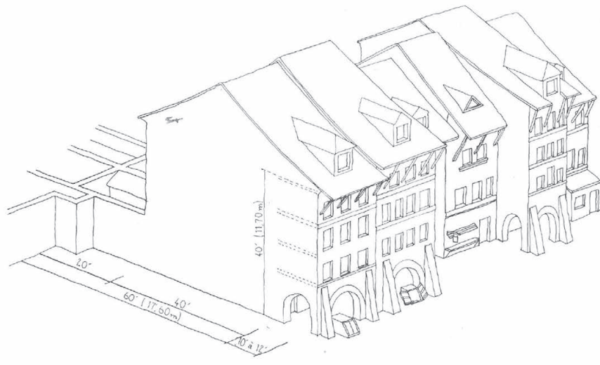
Les arcades comme gain d'espace.
