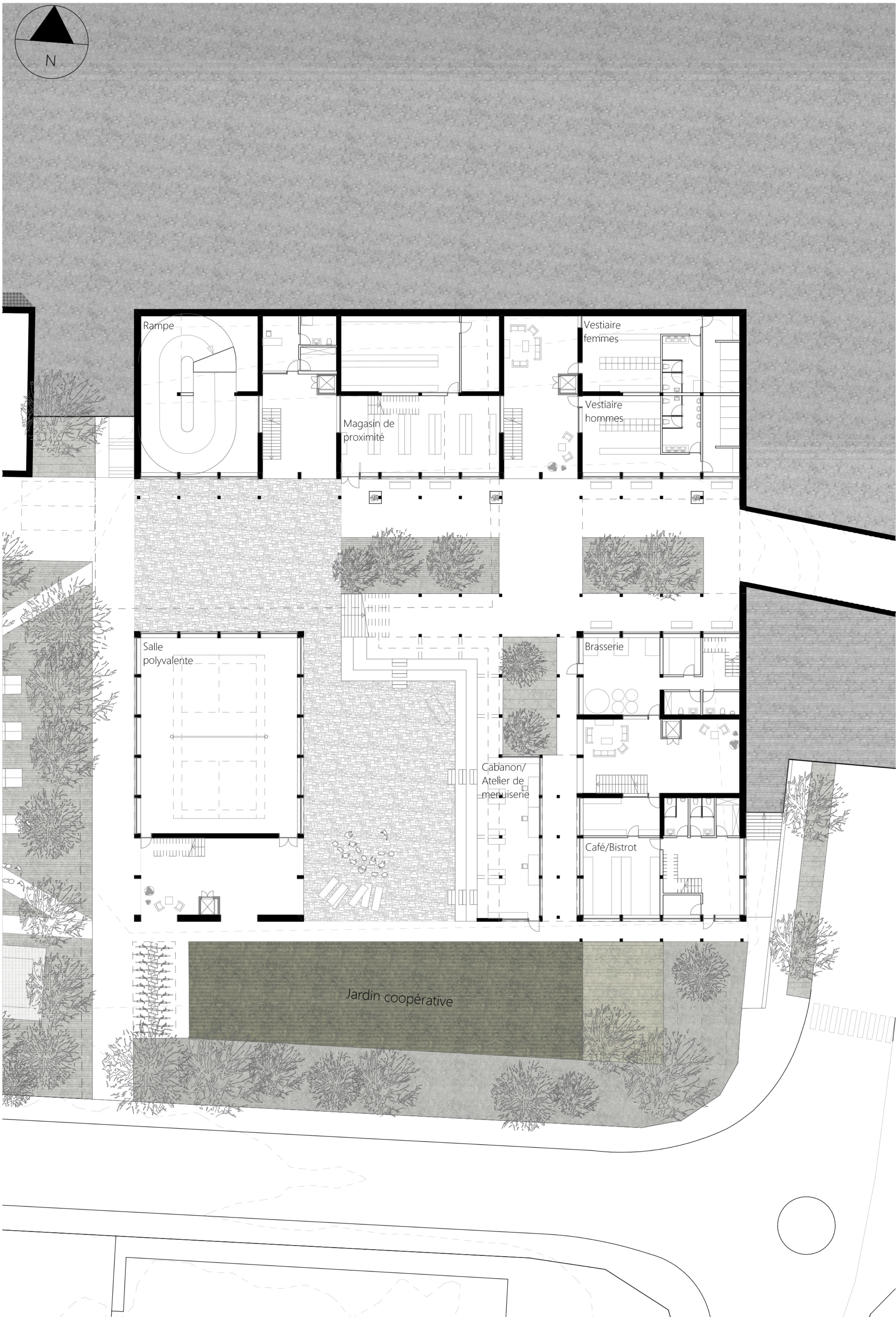
Rez-de-chaussée inférieur / 1:200
