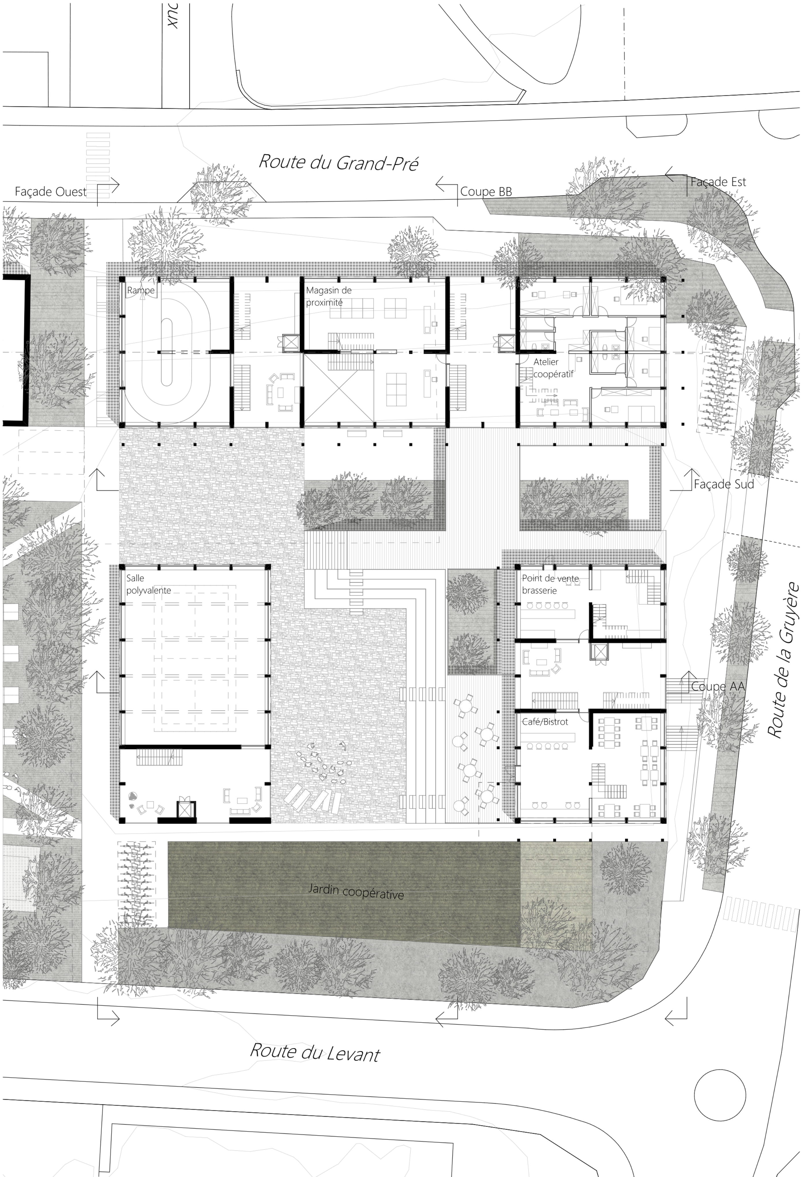
Rez-de-chaussée supérieur / 1:200
