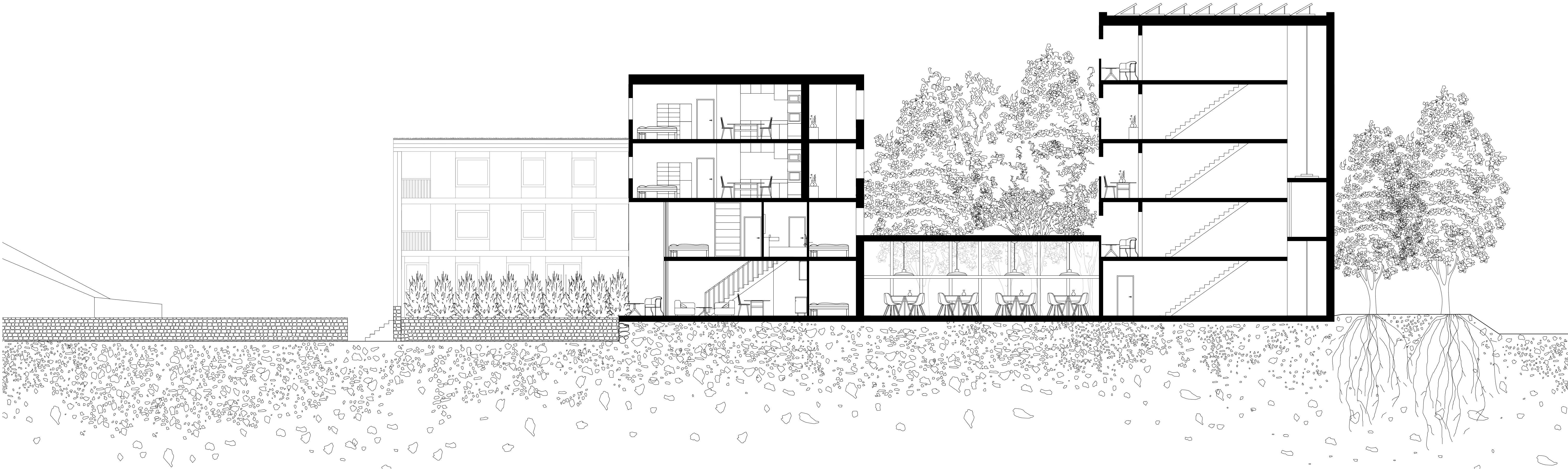
Coupe ouest 1:100
