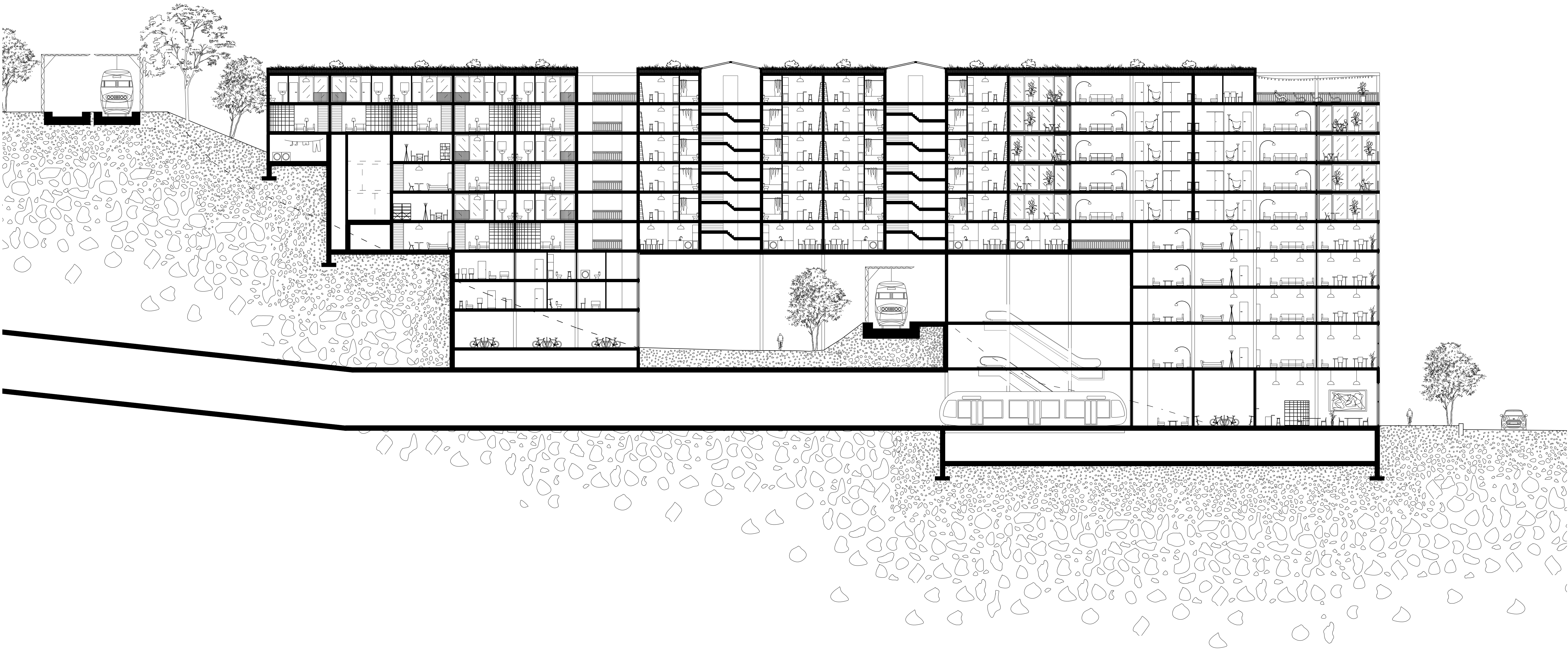
Coupe transversale ouest 1:200
