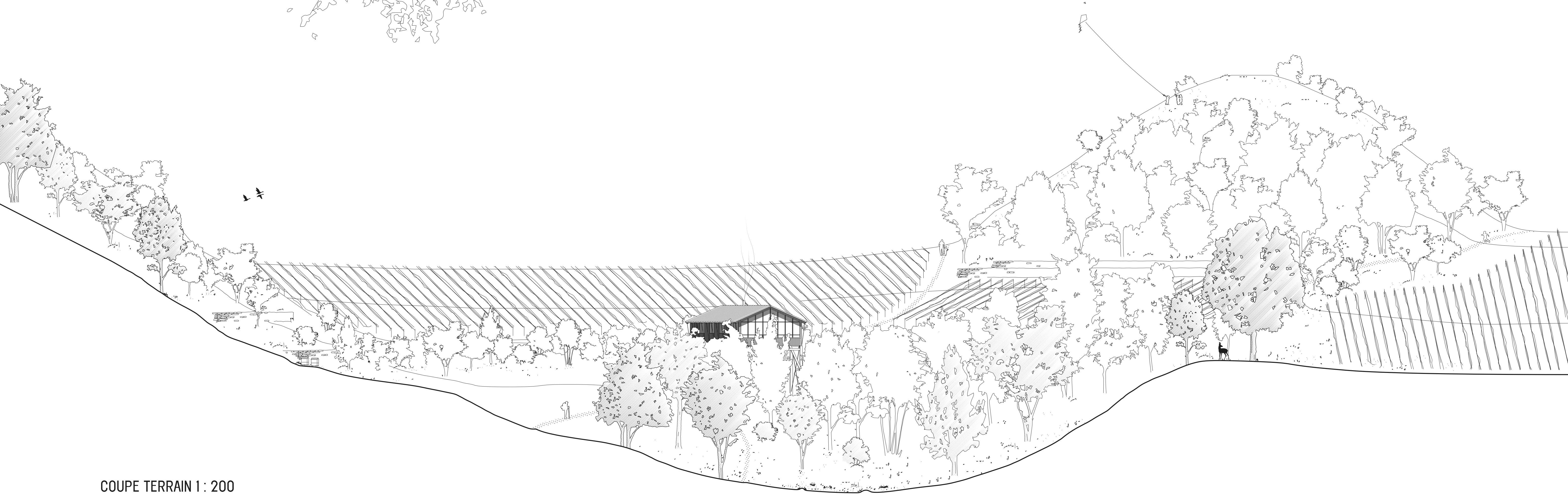
COUPE TERRAIN 1 : 200
