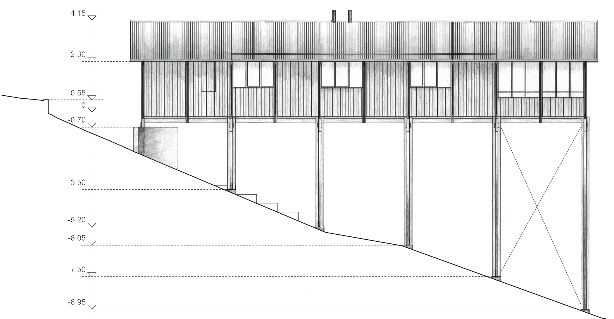
FACADE OUEST 1 : 100
