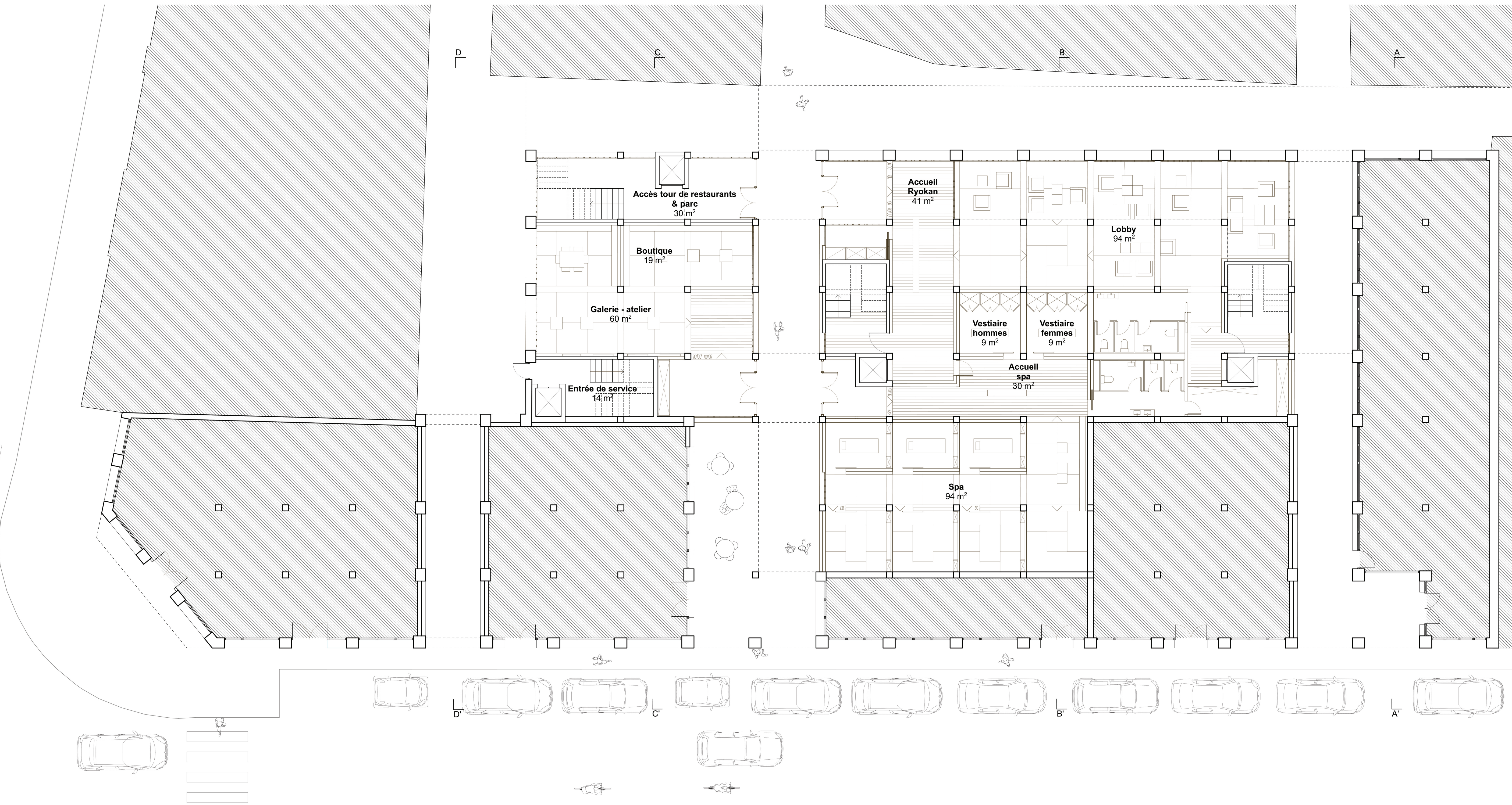
🕒 Rez-de-Chaussée, Ruelle Japonaise 1/100e
