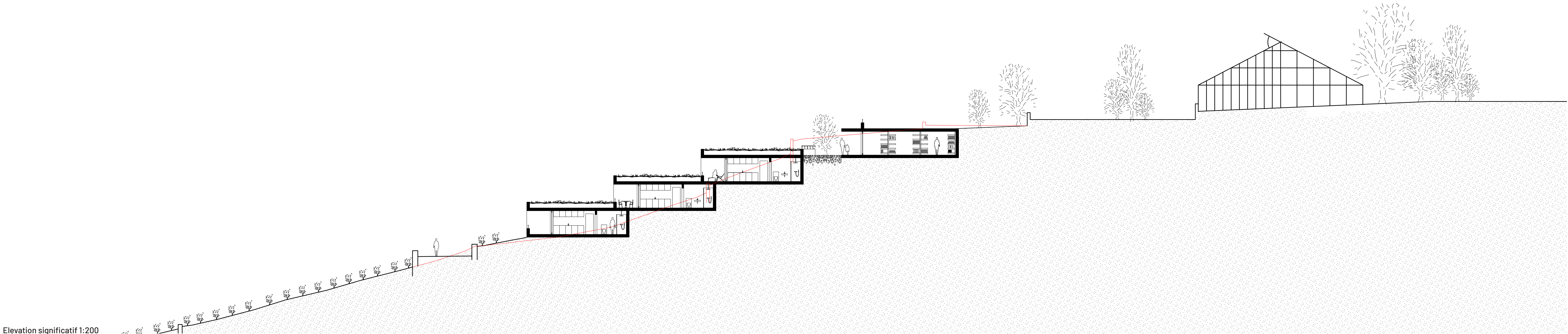
Elevation significatif 1:200
