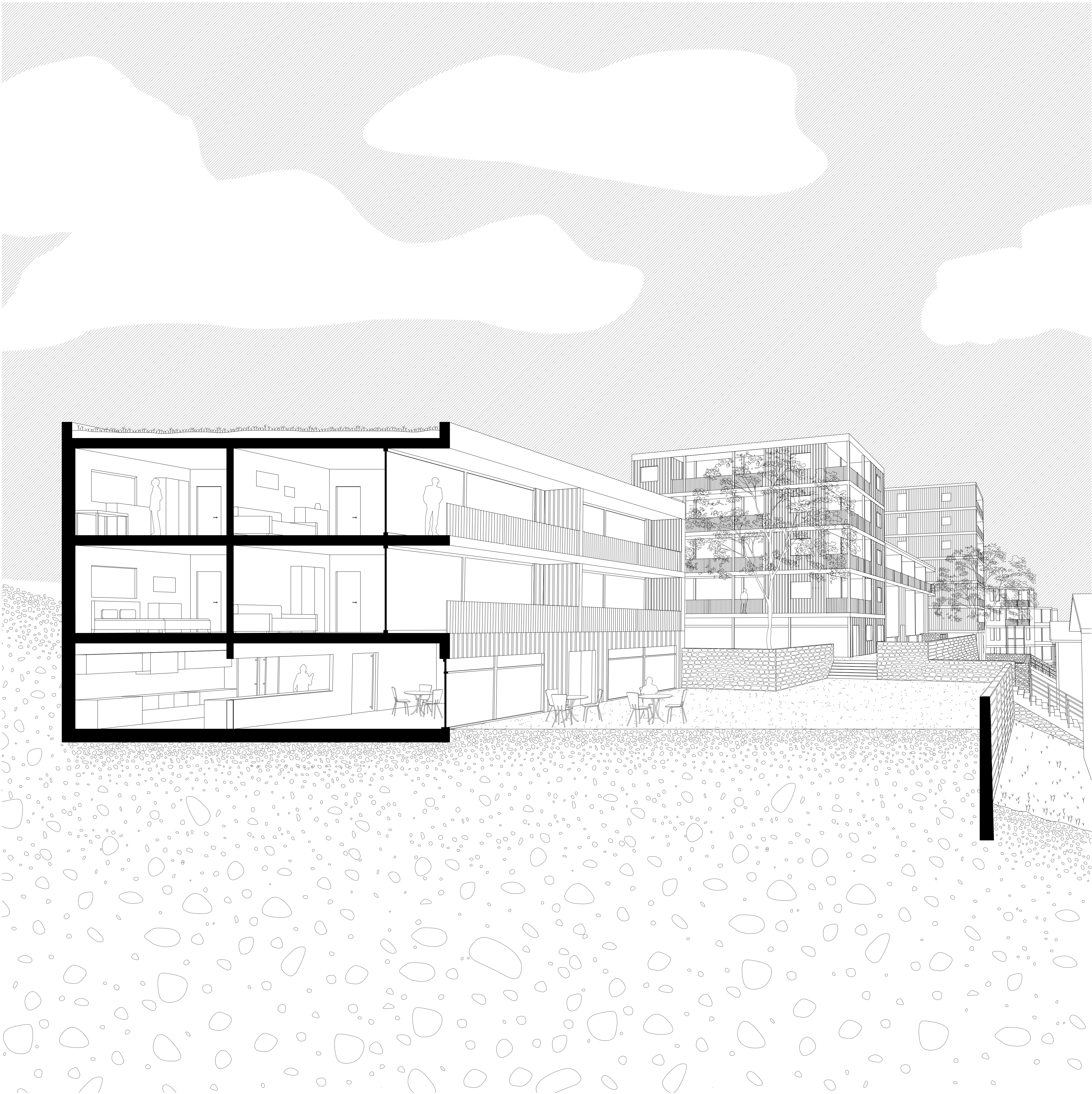
Coupe perspective, partie haute du site
