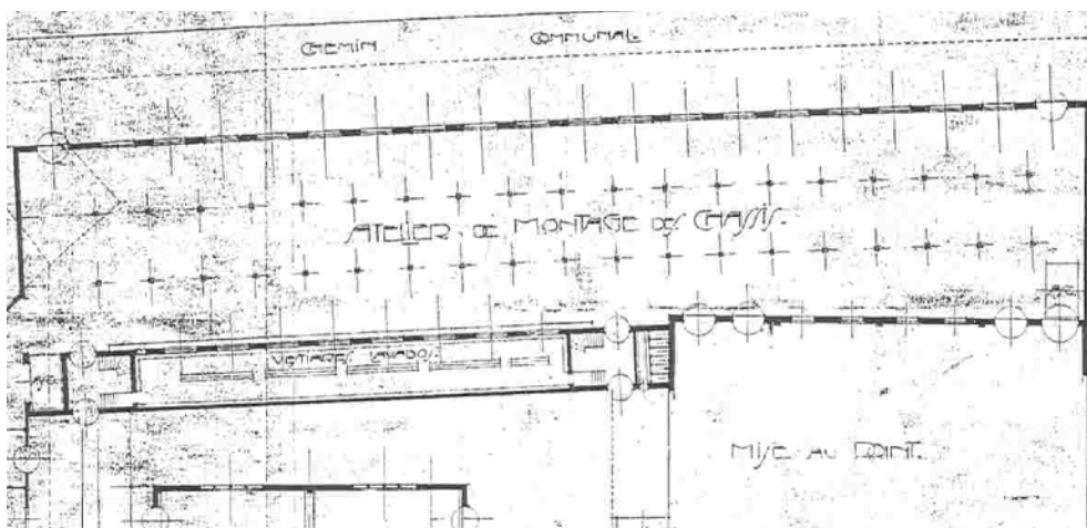
Plan du rez-de-chaussée d'origine de l'usine Pic-Pic, avec son vaste atelier de montage et ses 20 travées structurelles, 1917 © Bénédicte Frommel et Tanari Architectes
