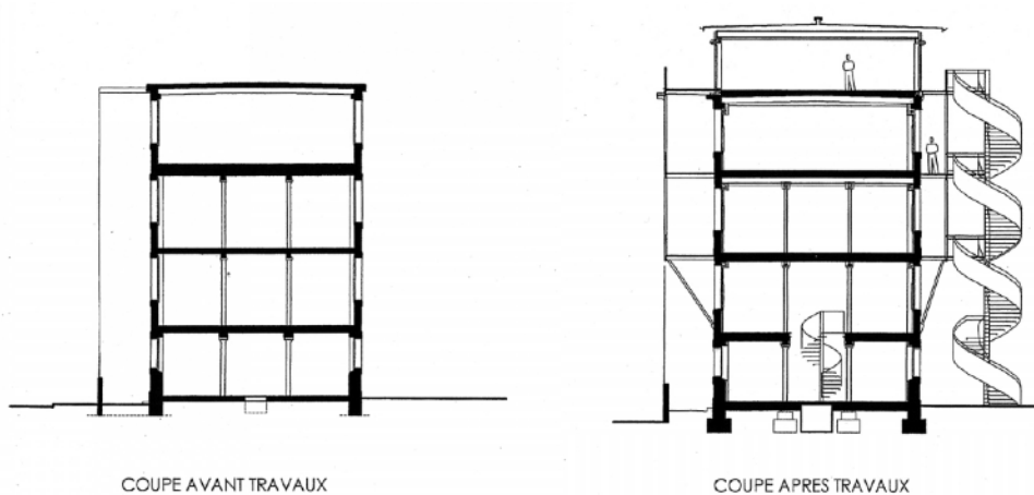
Immeuble Cinégram, coupe transversale (Est-Ouest) avant et après rénovation © BLSA Architectes
