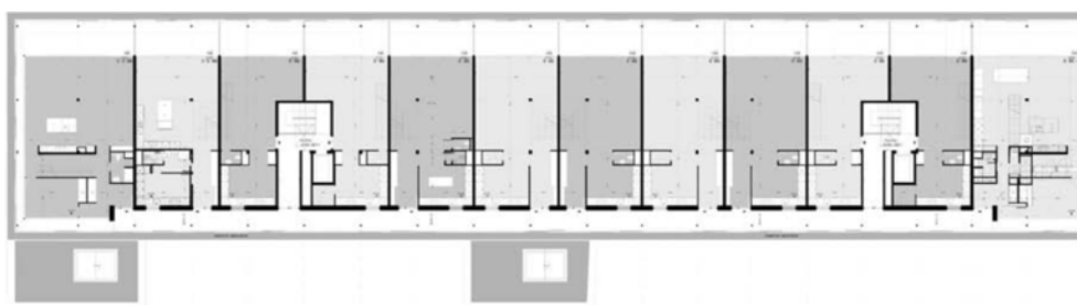
Plan de l'étage 3 (surélévation)
