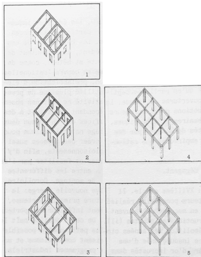
Les cinq systèmes constructifs de l'architecture industrielle à Genève par J.-M. Lamunière et B. Gachet, 1987
