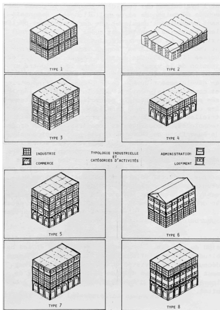
Les huit typologies d'architecture industrielle à Genève par J.-M. Lamunière et B. Gachet, 1987
