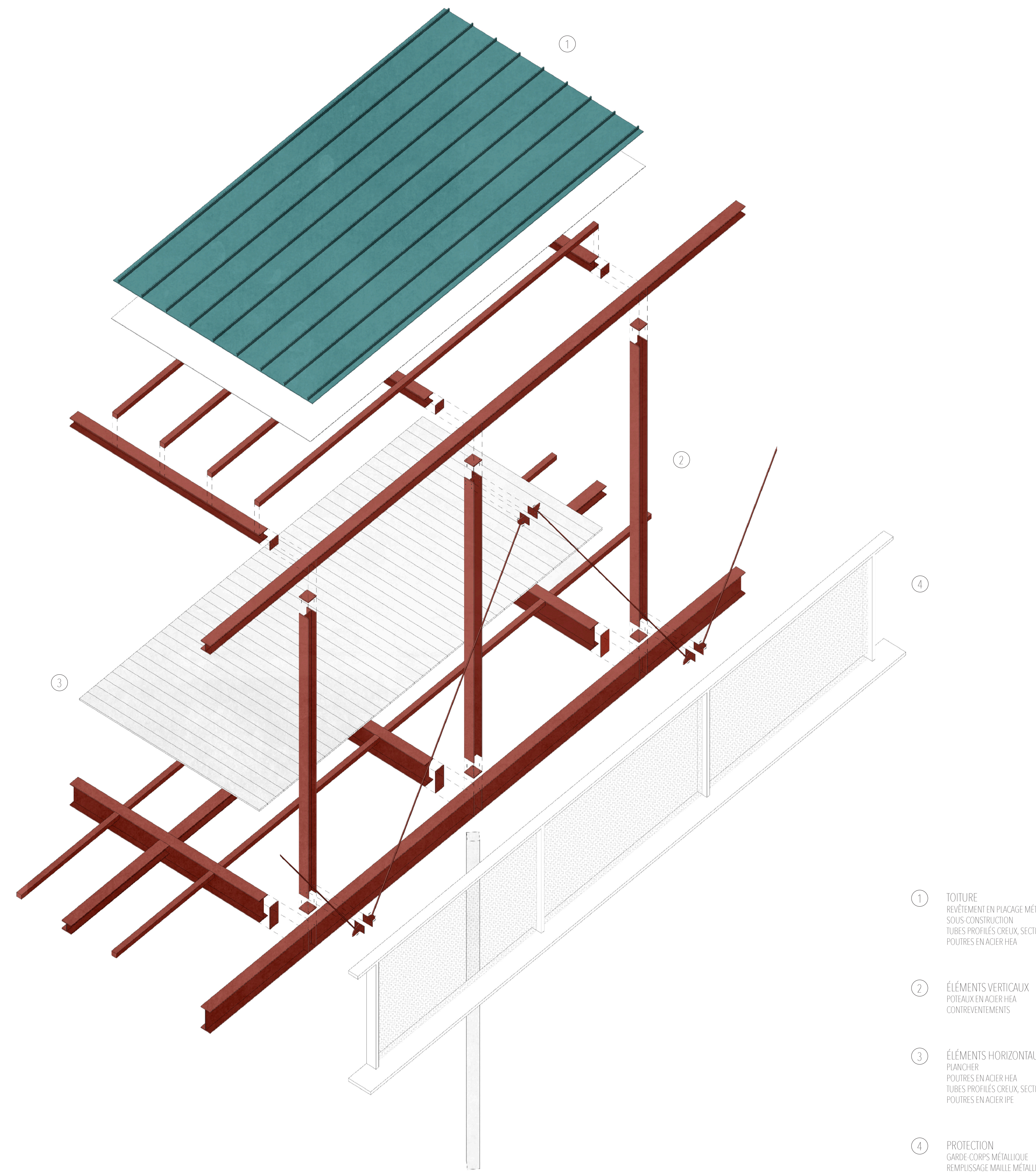
AXONOMÉTRIE STRUCTURELLE ÉCLATÉE 1:20
