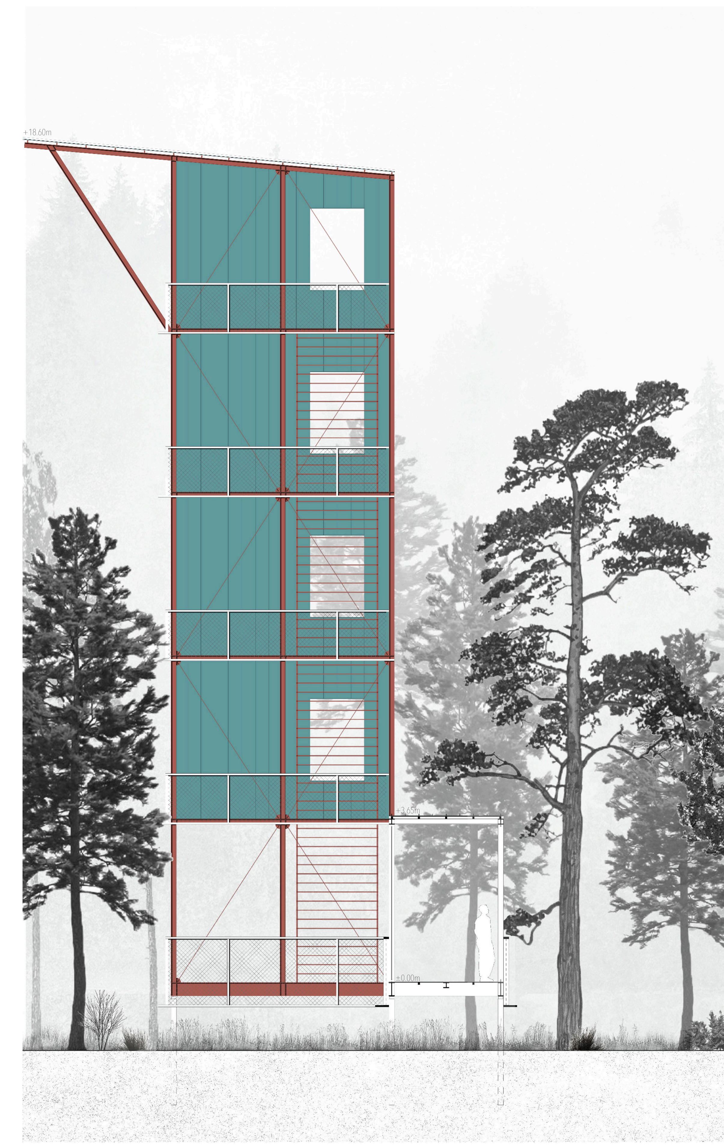
COUPE TRANSVERSALE 5 - POINT FINAL, LA TOUR 1:50
