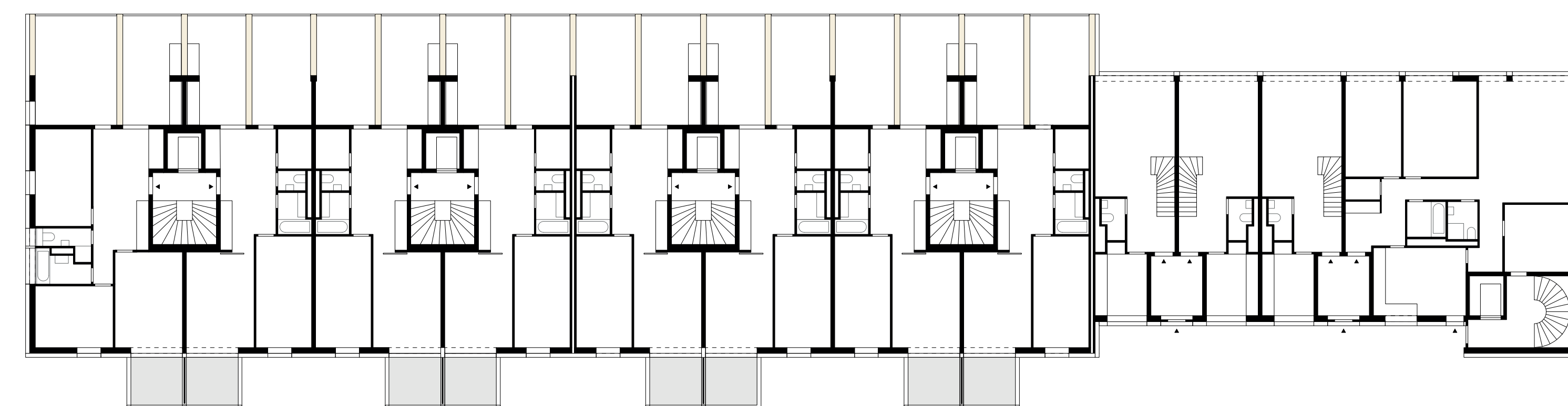
PLAN BAT. A_REZ INFERIEUR 1:200
