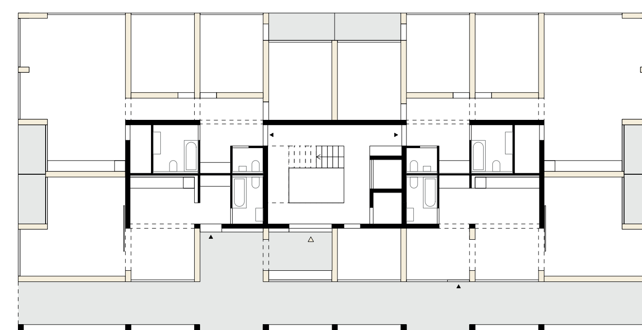
PLAN BAT. B_REZ-DE-CHAUSSEE 1:200
