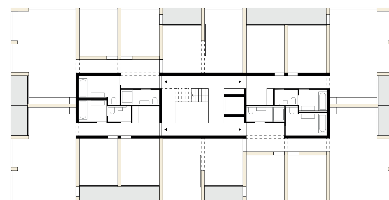
PLAN BAT. B_ETAGE TYPE 1:200
