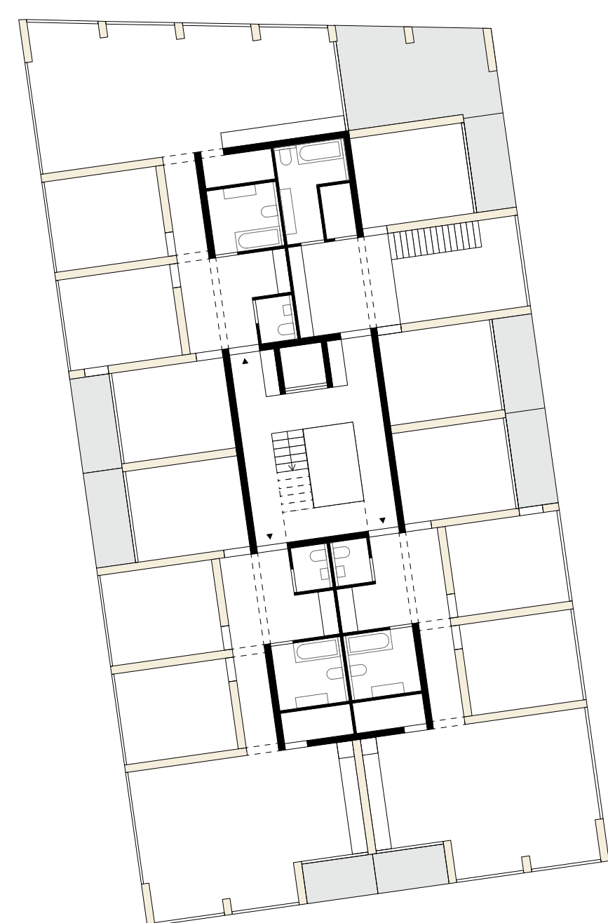
PLAN BAT. C_ETAGE TYPE DUPLEX 1:200
