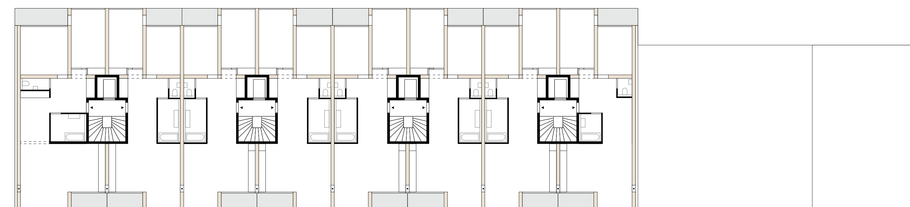
PLAN BAT. A_ETAGE TYPE 1:200
