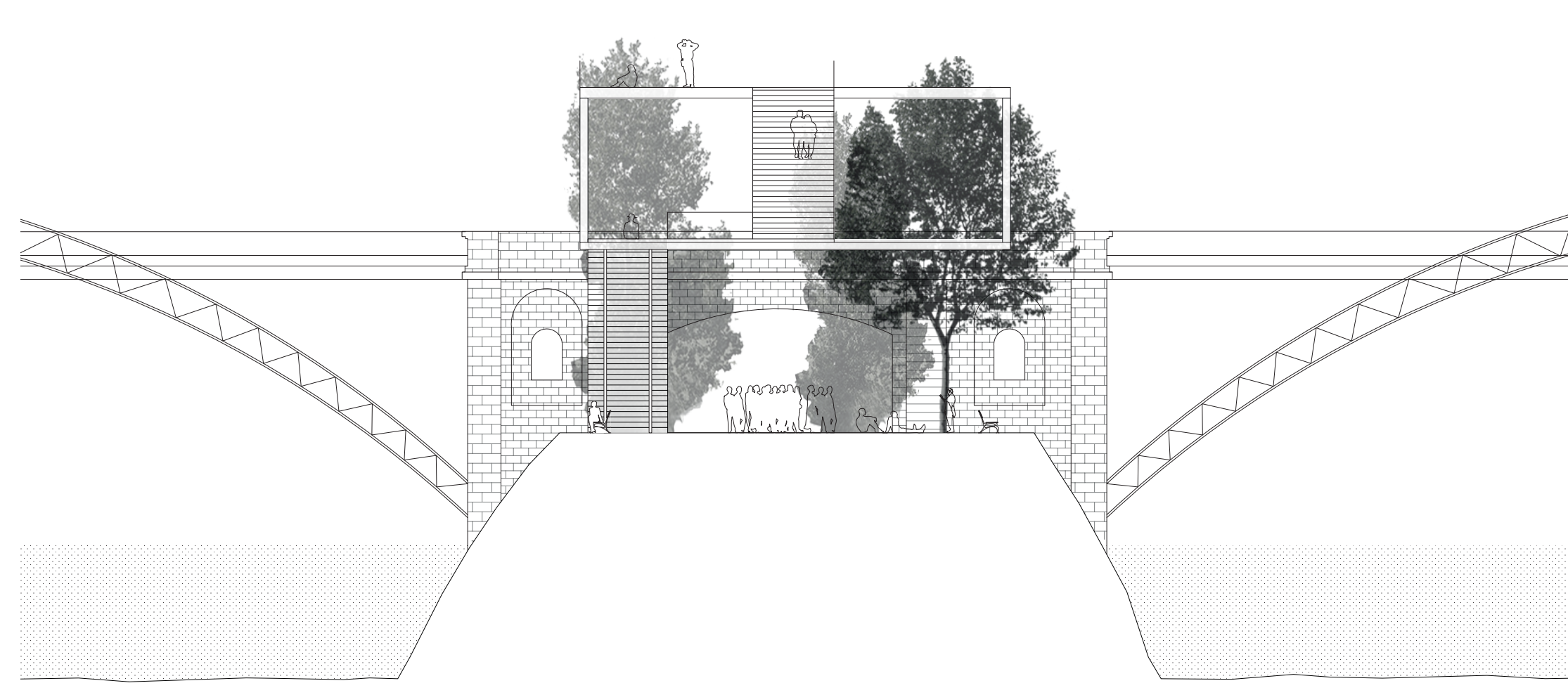
Section BB 1:200
