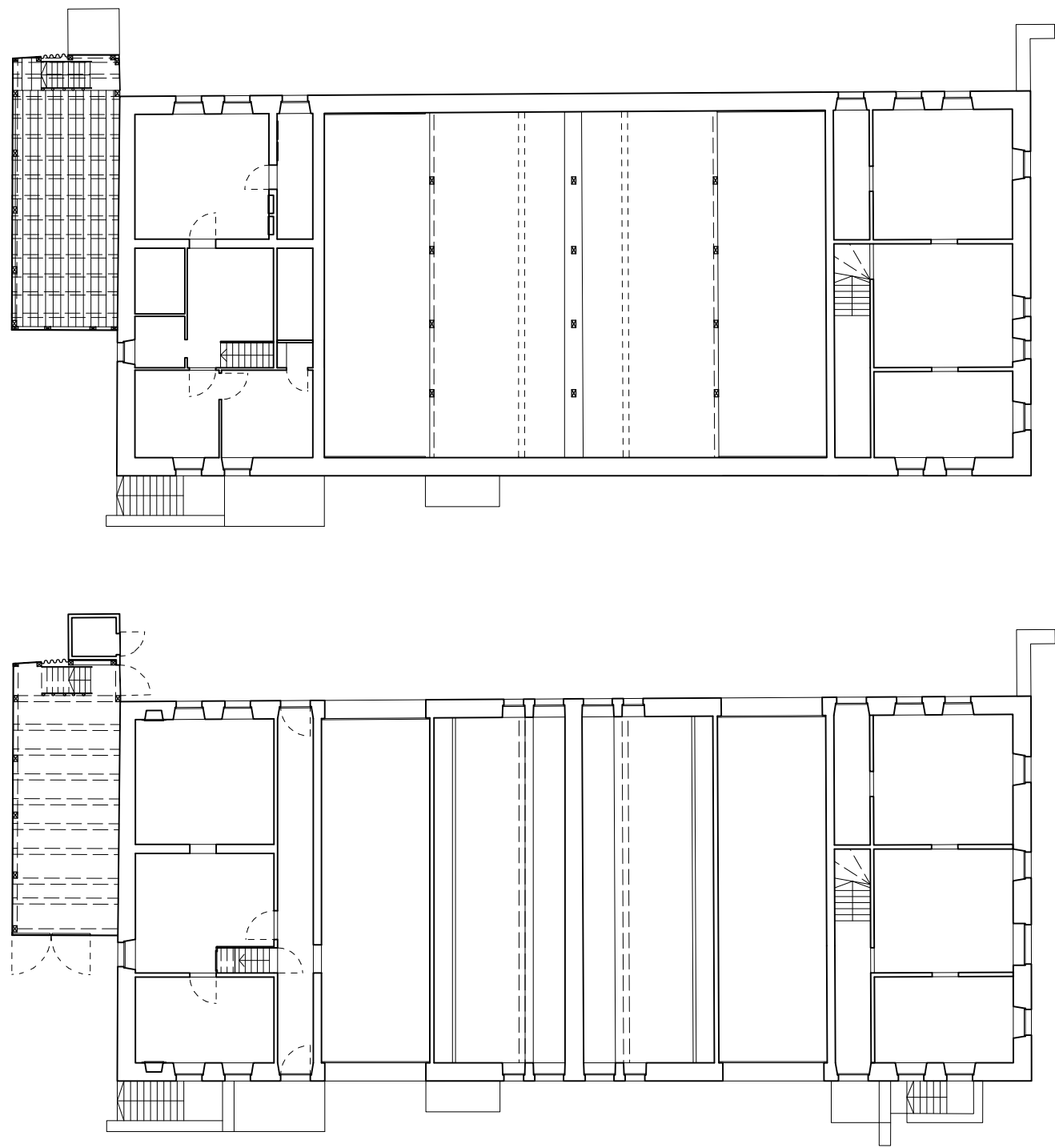
Plans des du rez et de l'étage, coupe transversale du logement et élévation du pignon nord
