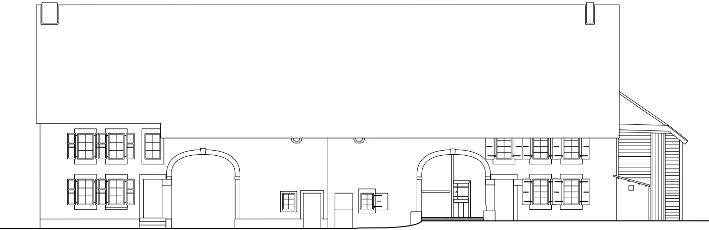
Coupe transversale, élévations des façade avant et arrière, coupe transversale dans la grange et élévation du pignon nord
