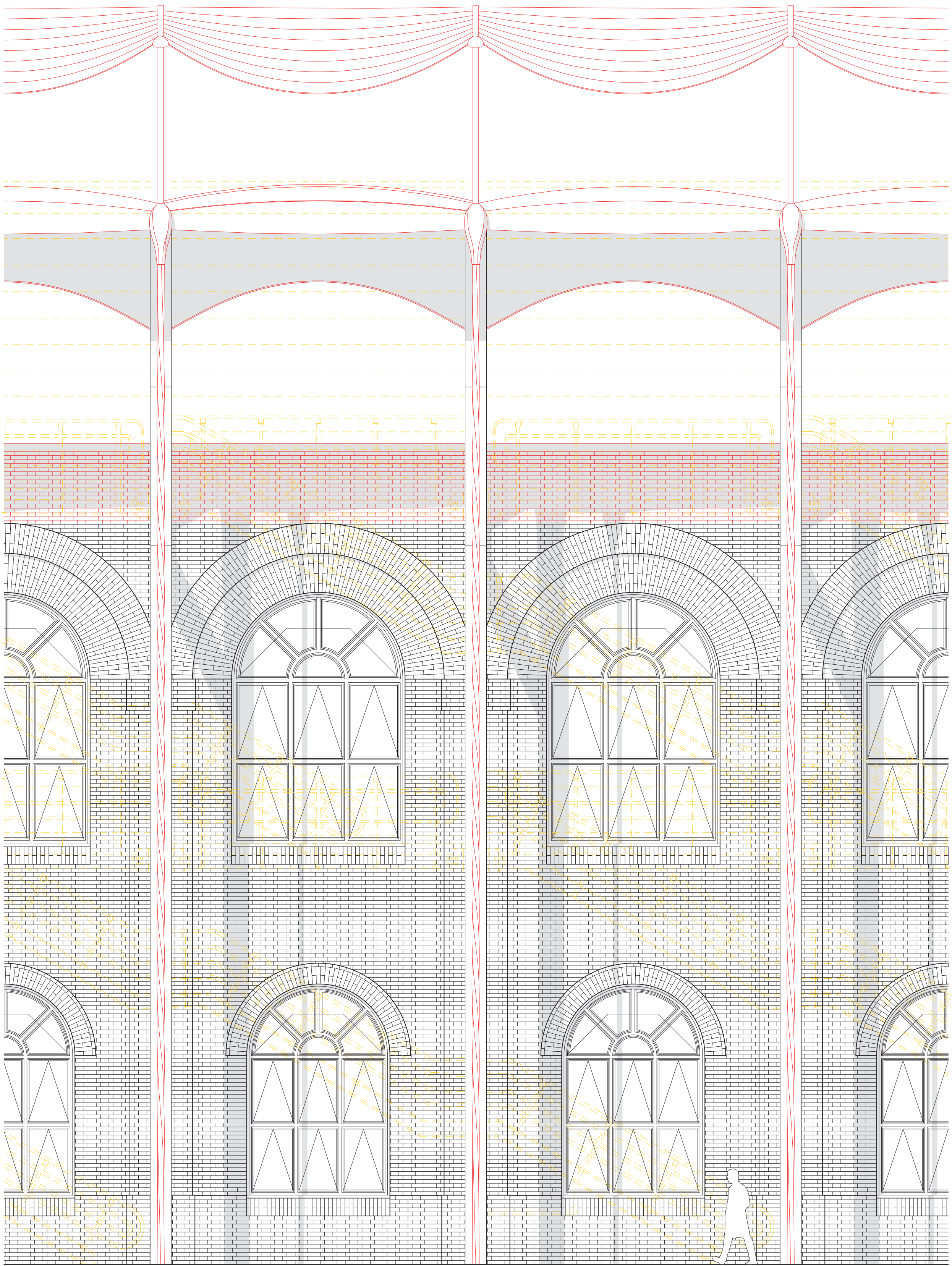
Élévation 1:50
