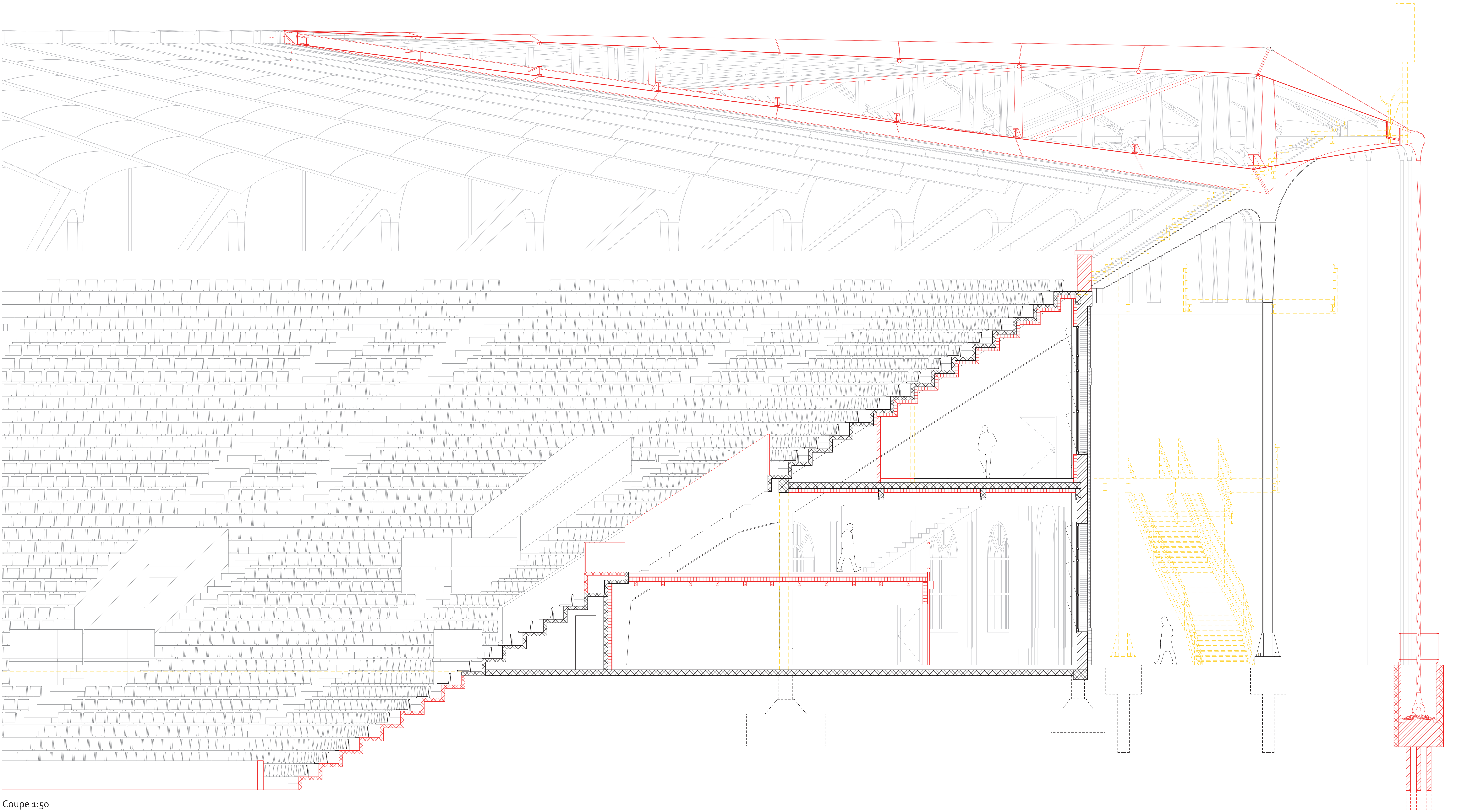
Coupe 1:50
