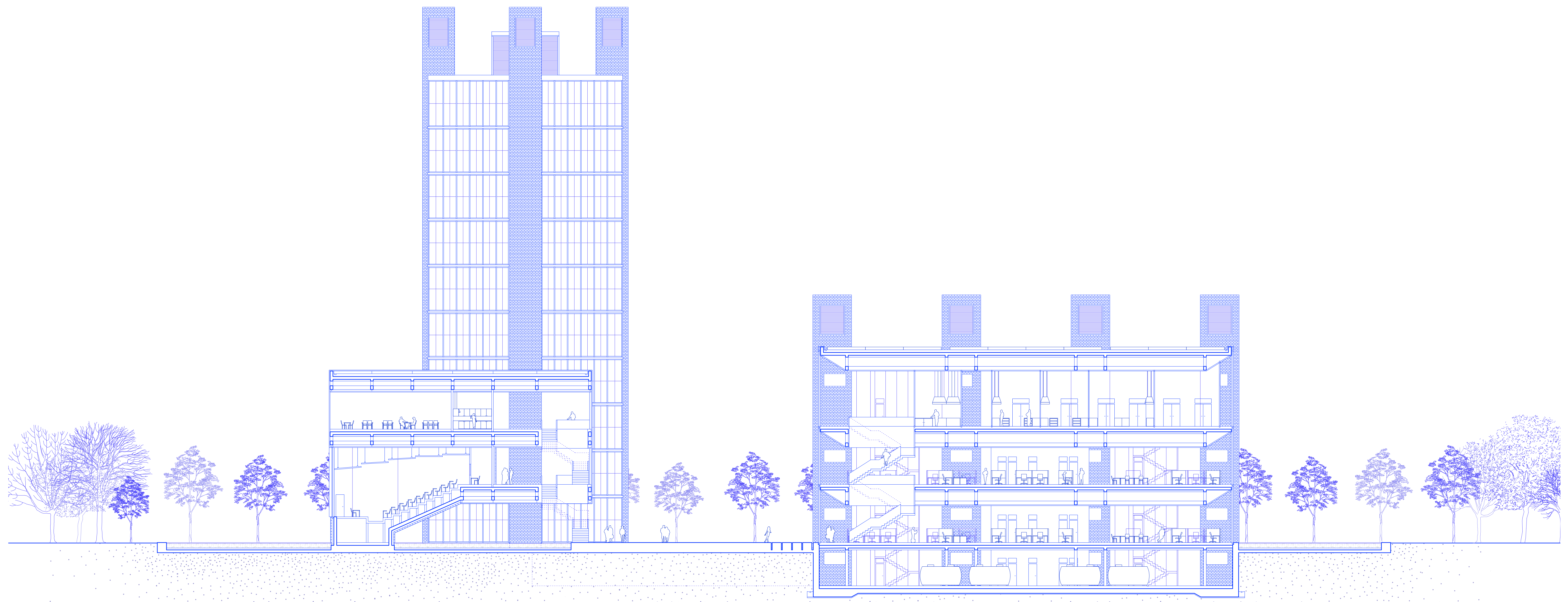
Coupe AA | 1:200
