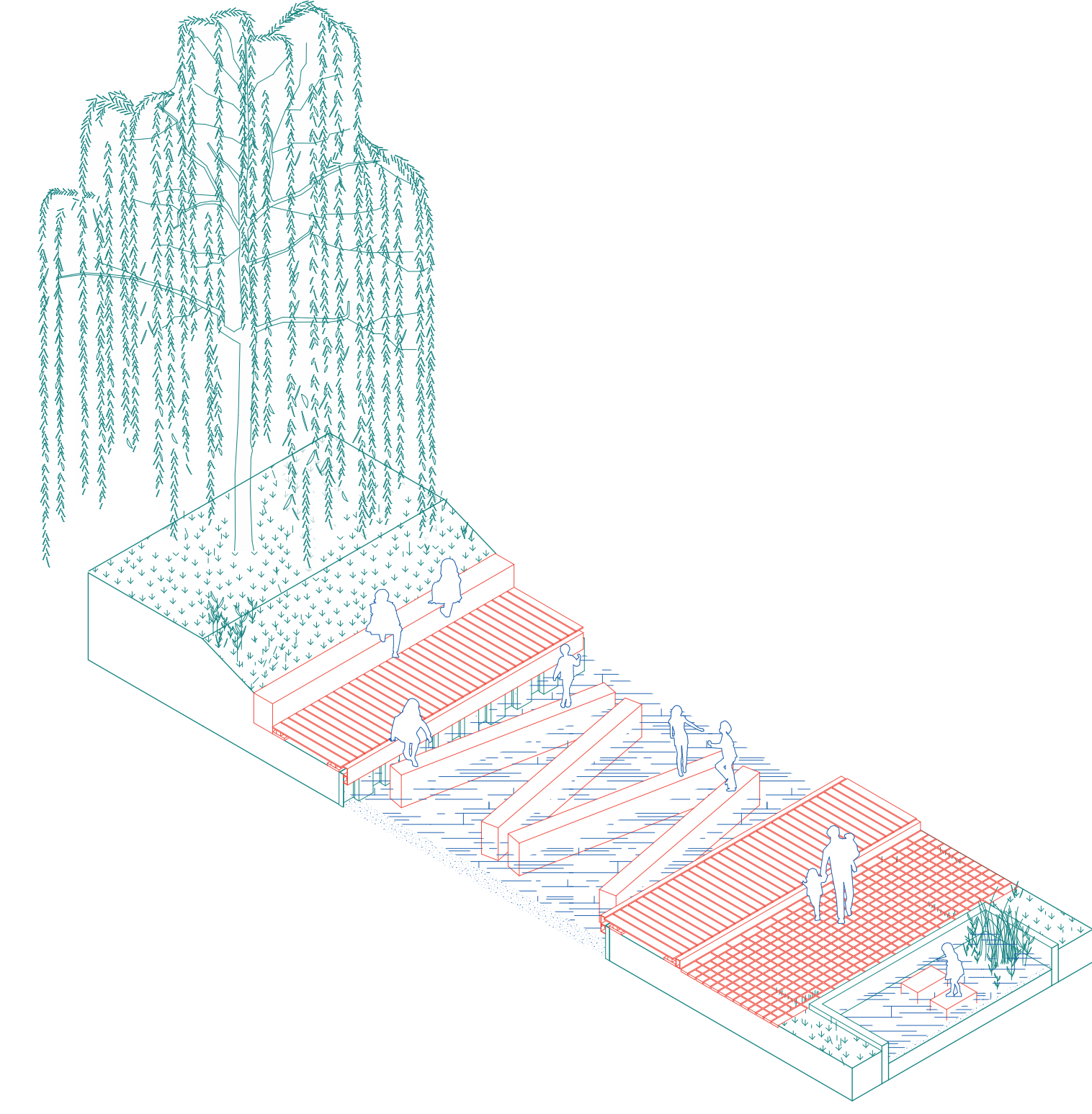
PASSAGE DES CASTORS 1:100
