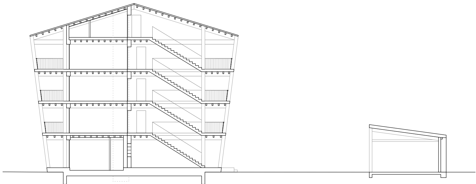
Coupe aa'
