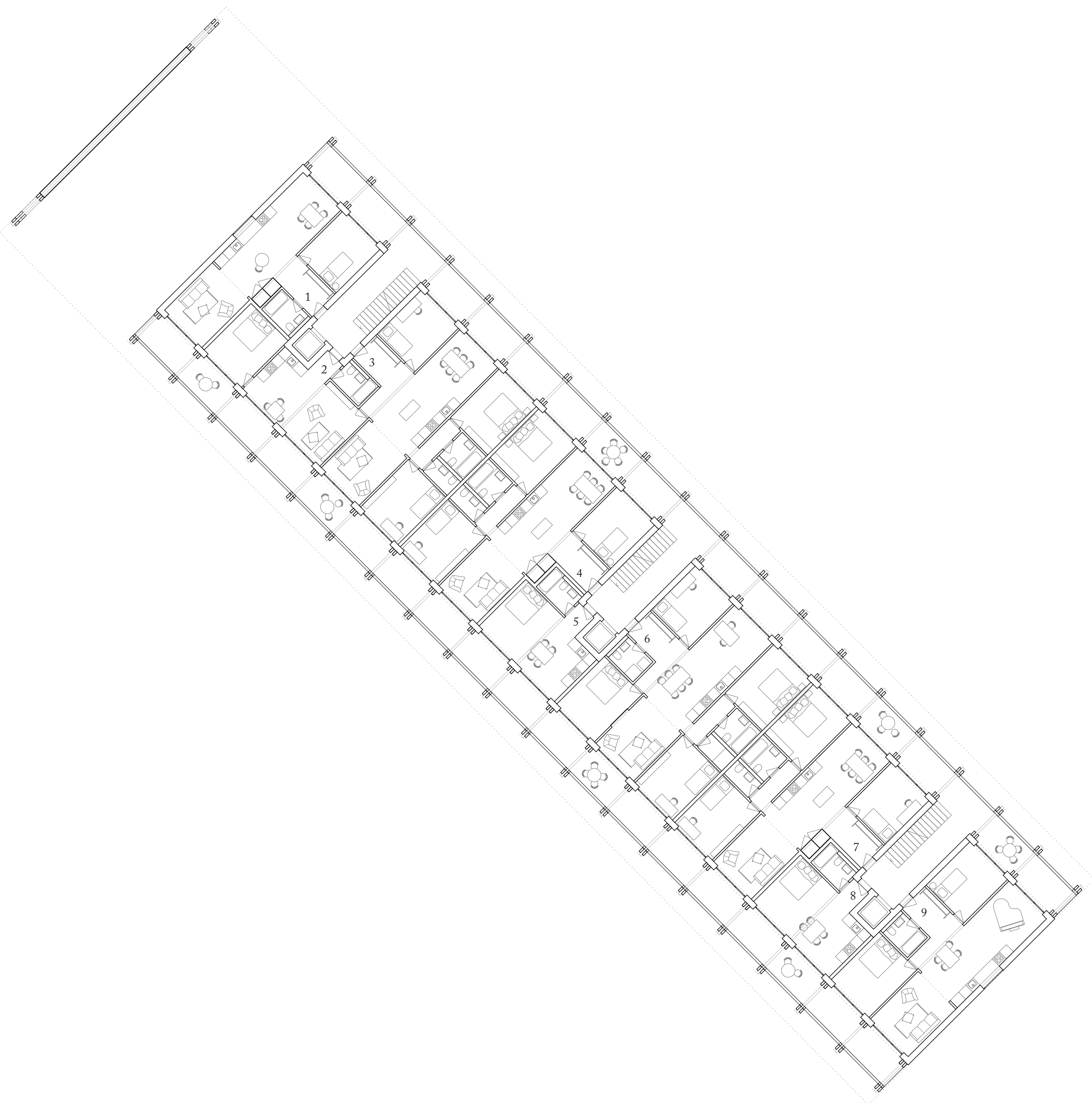
Plan du premier étage
