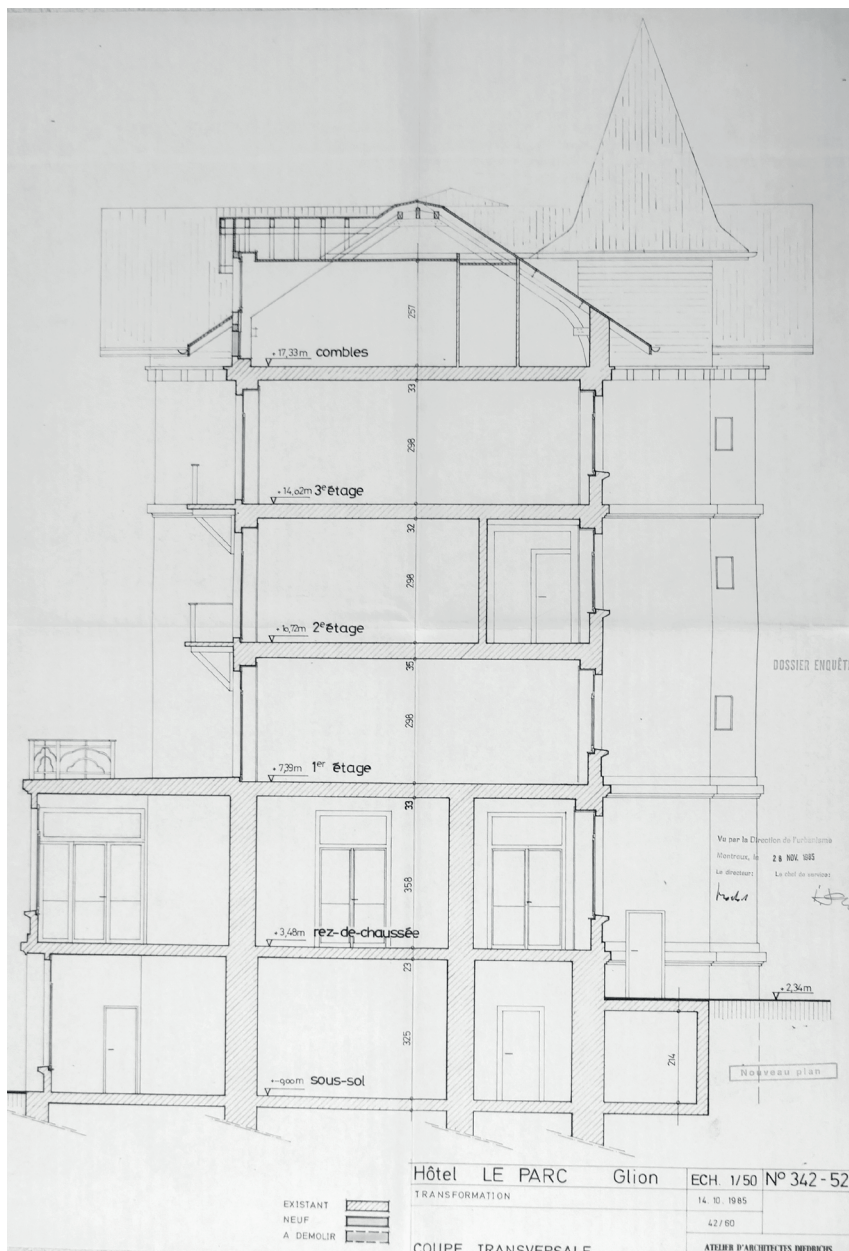
Hôtel du Parc, Glion - Coupe signée par l'atelier d'architectes Diedrichs, octobre 1985
