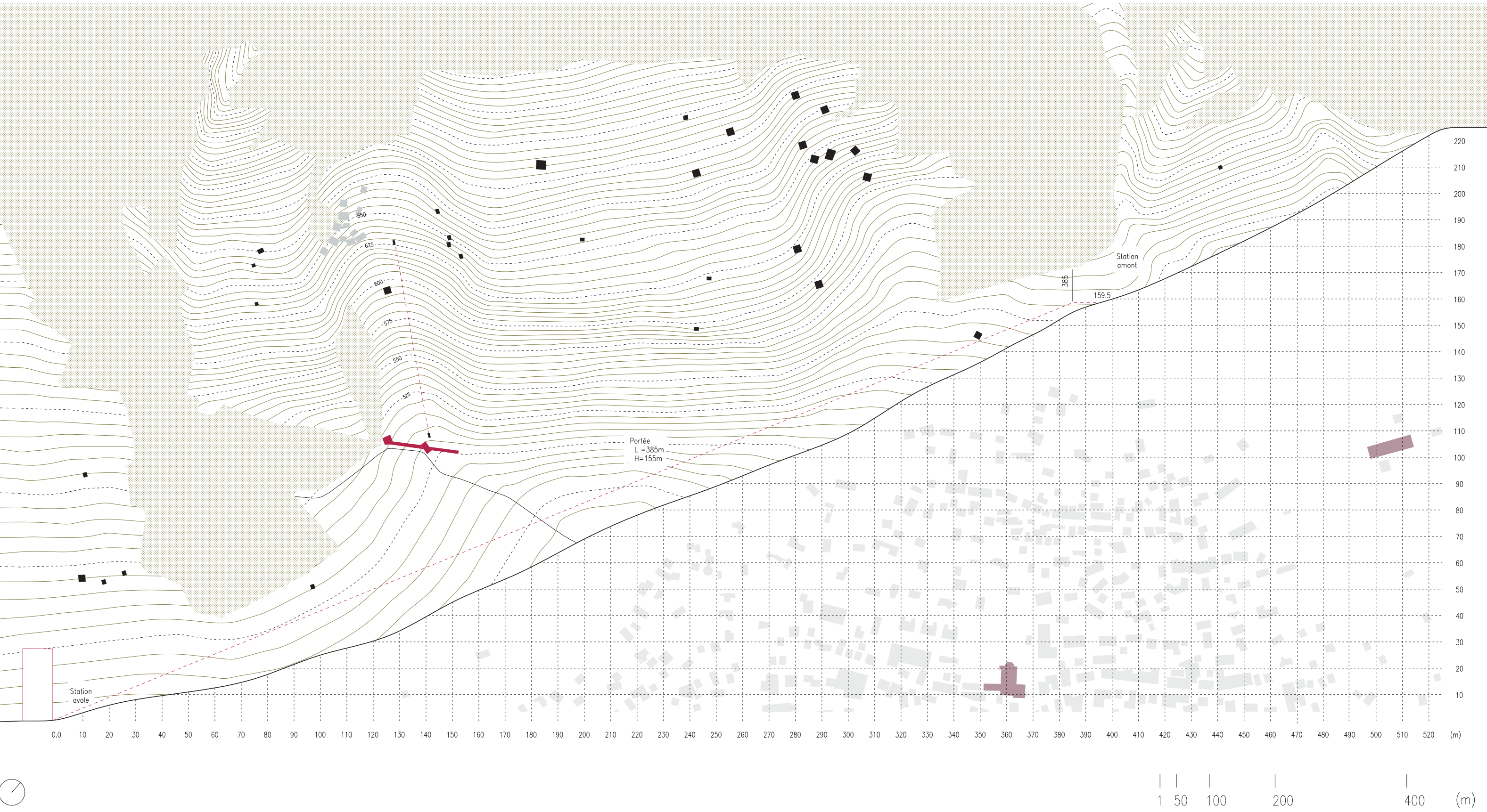
CARTE ET COUPE DE LA TOPOGRAPHIE DE LA 'COMBE D'ENFER'
