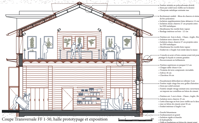
Coupe Transversale FF 1-50, halle prototypage et exposition
