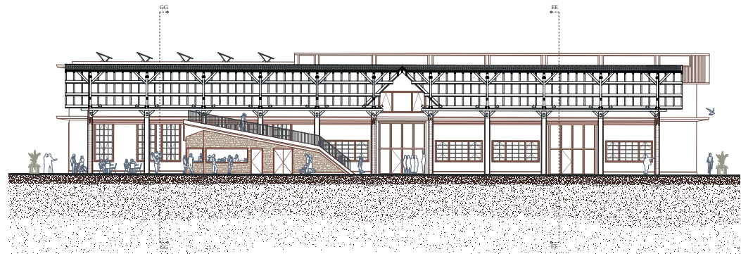
Coupe Longitudinale DD 1-100, Couvert et Pavillon
