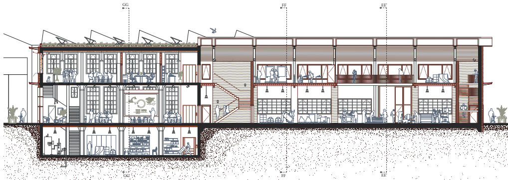
Coupe Longitudinale CC 1-100 - Centre de formation, Bureau d'étude, Halle de prototypage et Espace d'exposition
