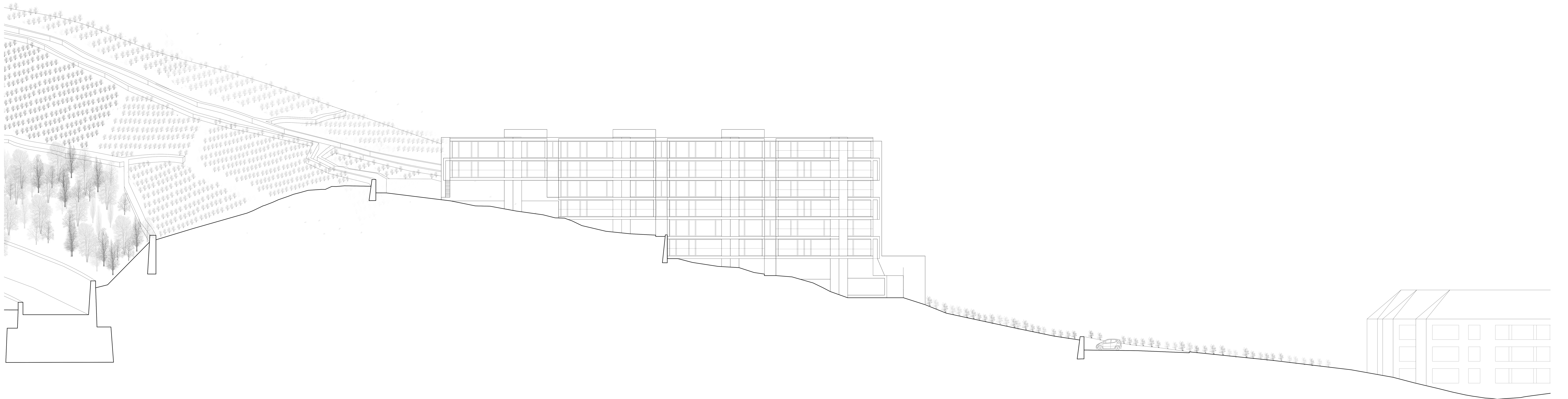
Facade sud 1:200
