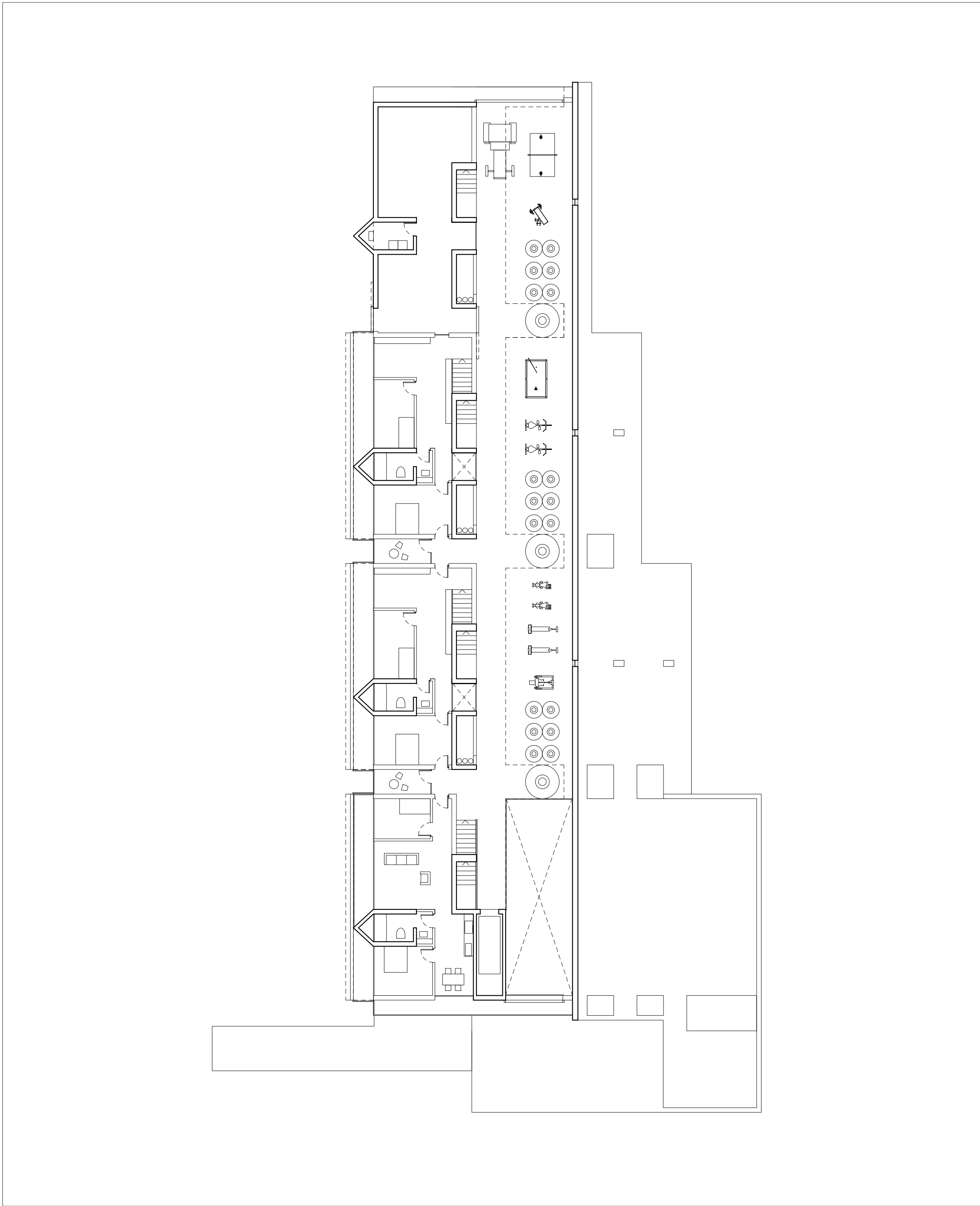
Plan improductif ± 0.00m 1:200
