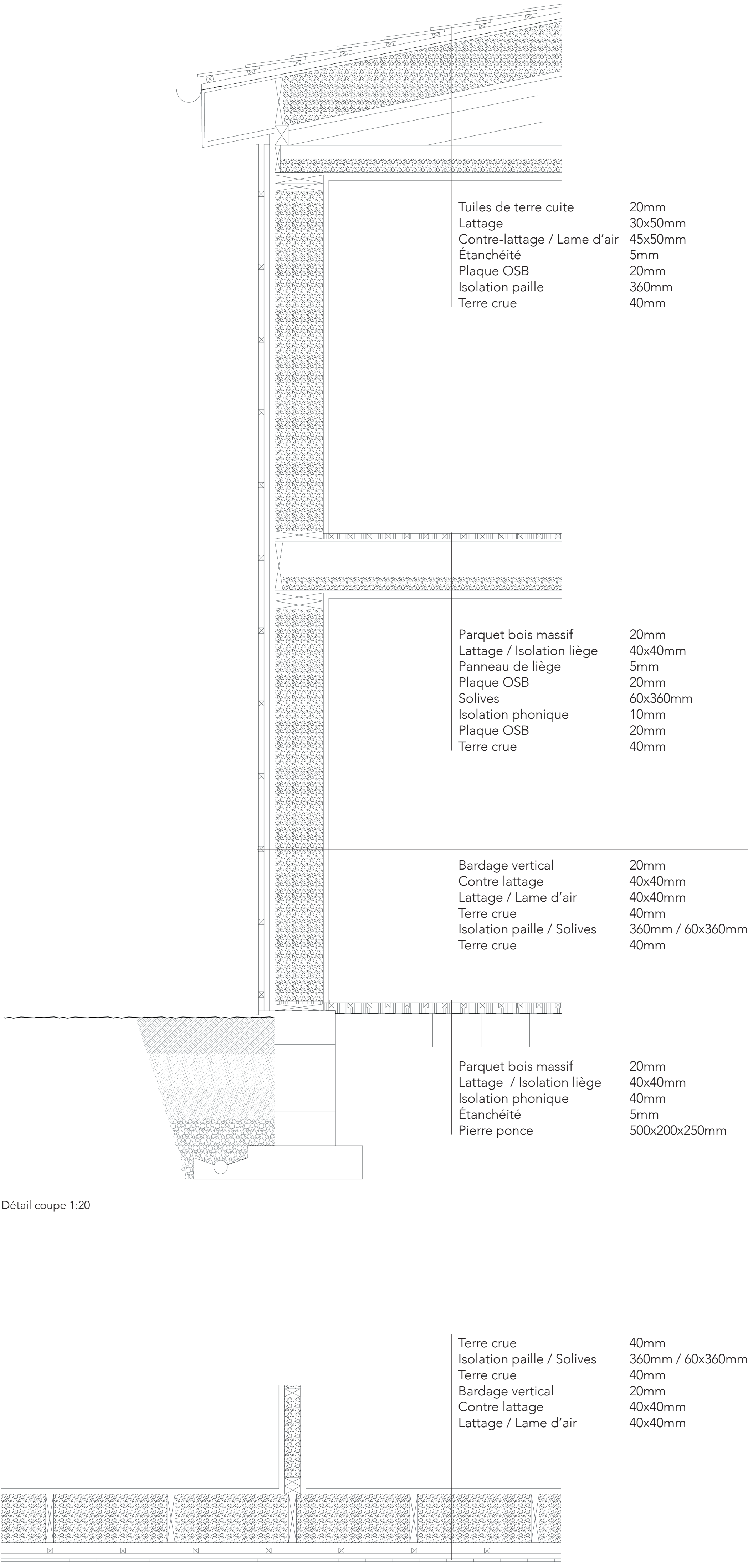
Détail plan 1:20
