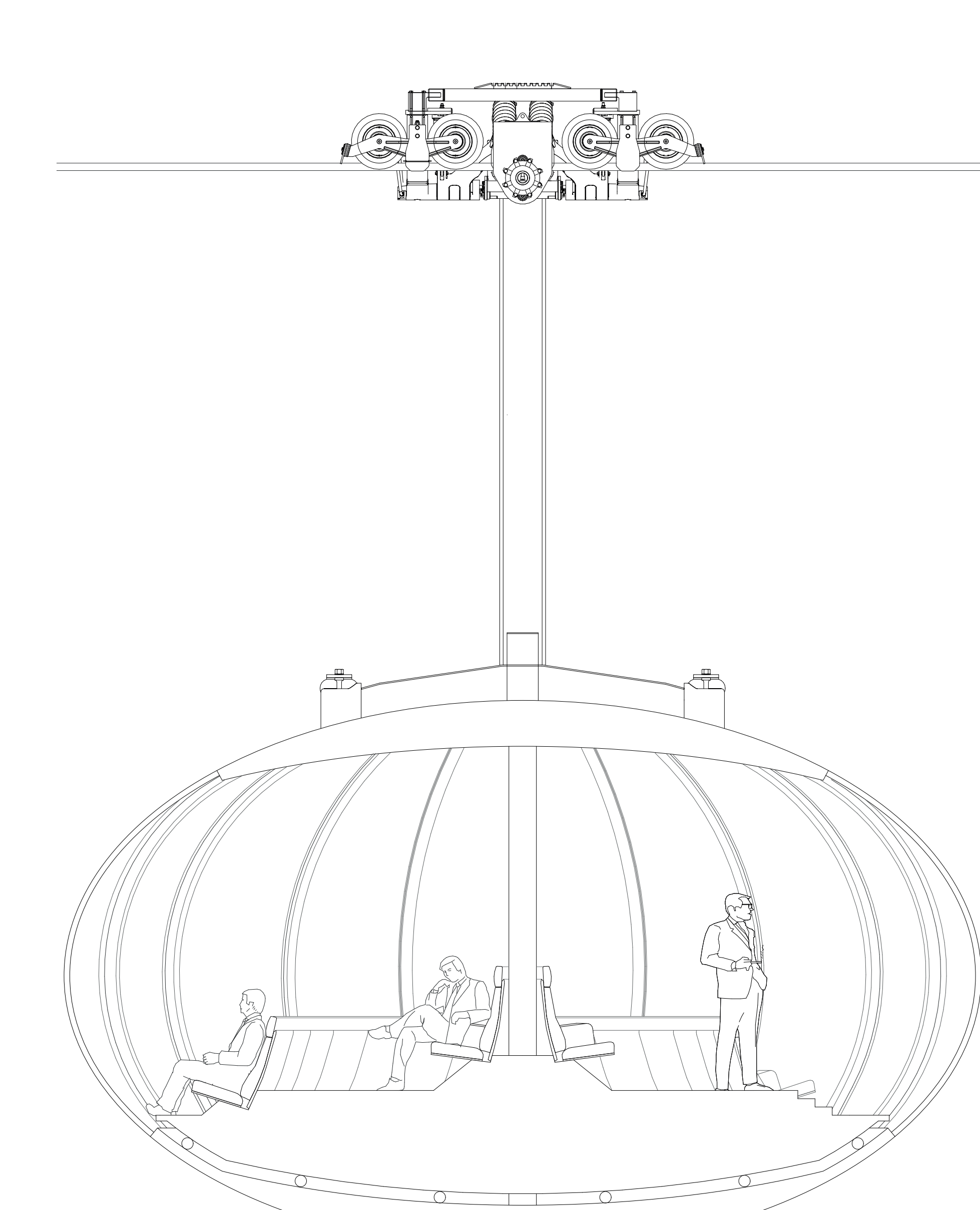
COUPE D'UNE CABINE DE L'EXPÉDITION 209 1: 33
