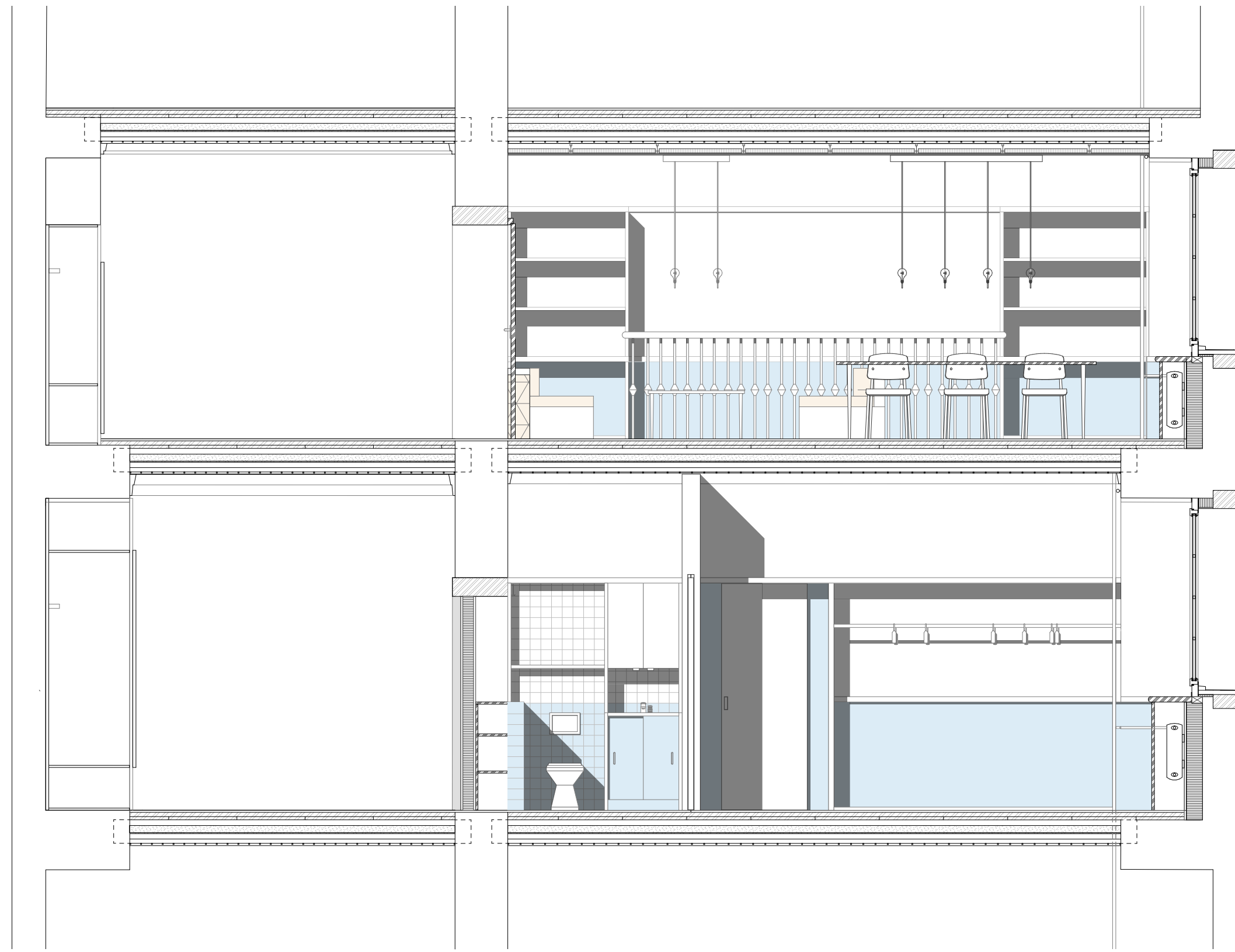
Coupe J'-J
