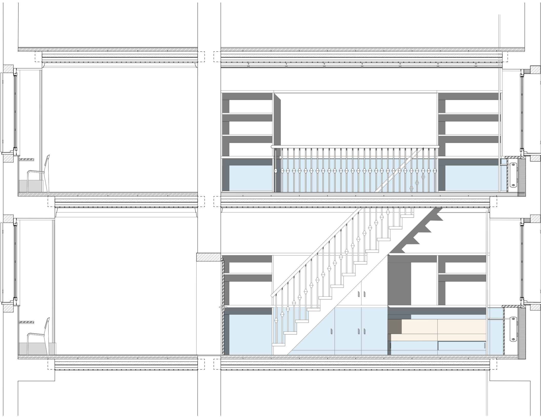
Coupe I'-I
