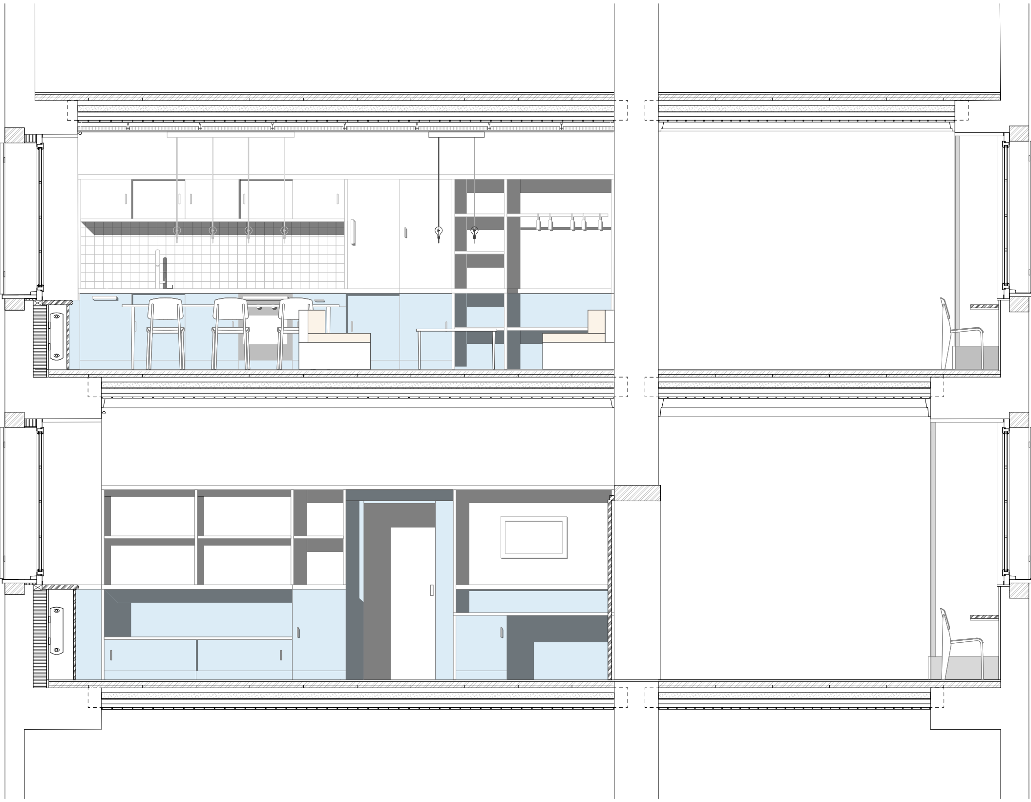
Coupe I-I'
