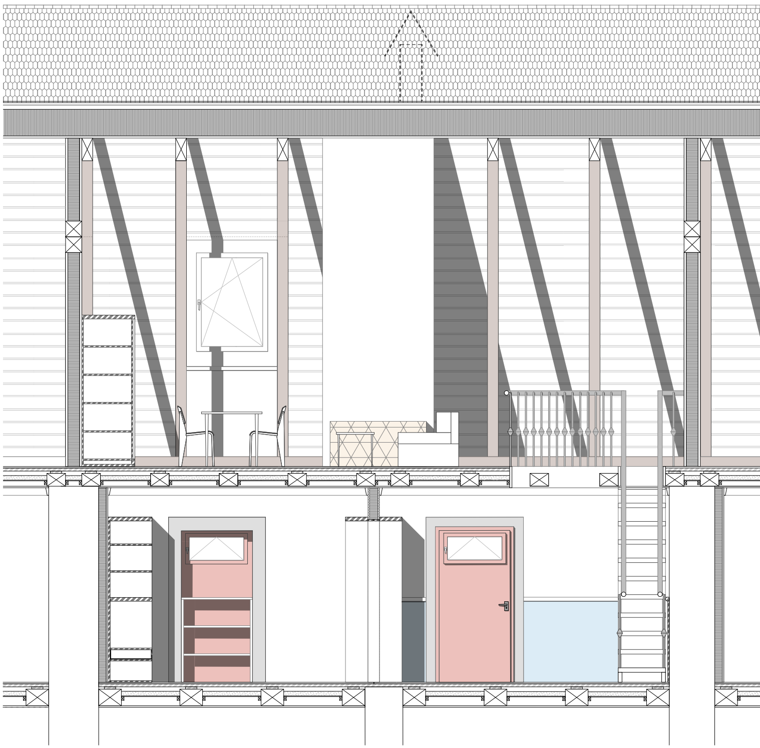
Coupe H-H'
