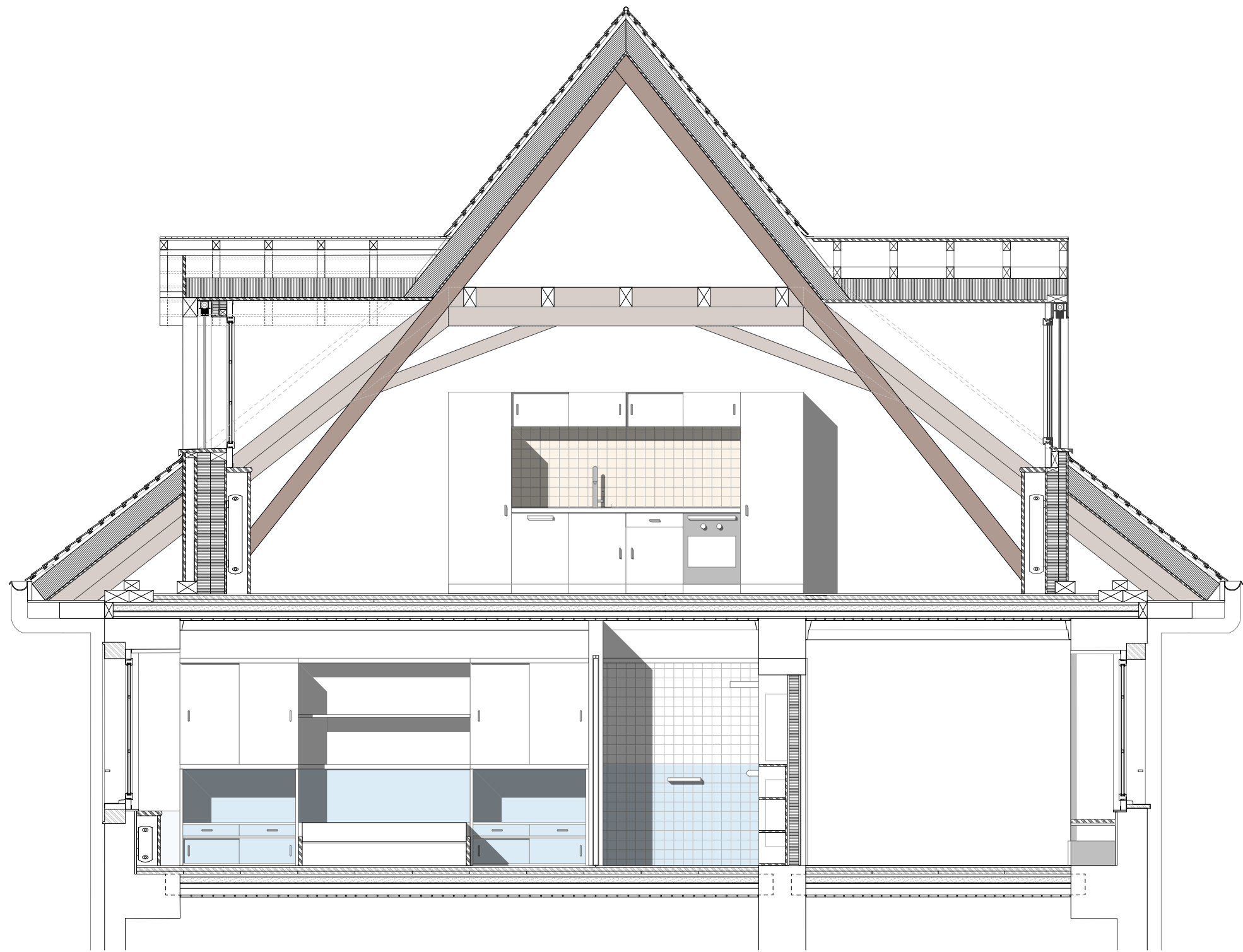
Coupe G-G'
