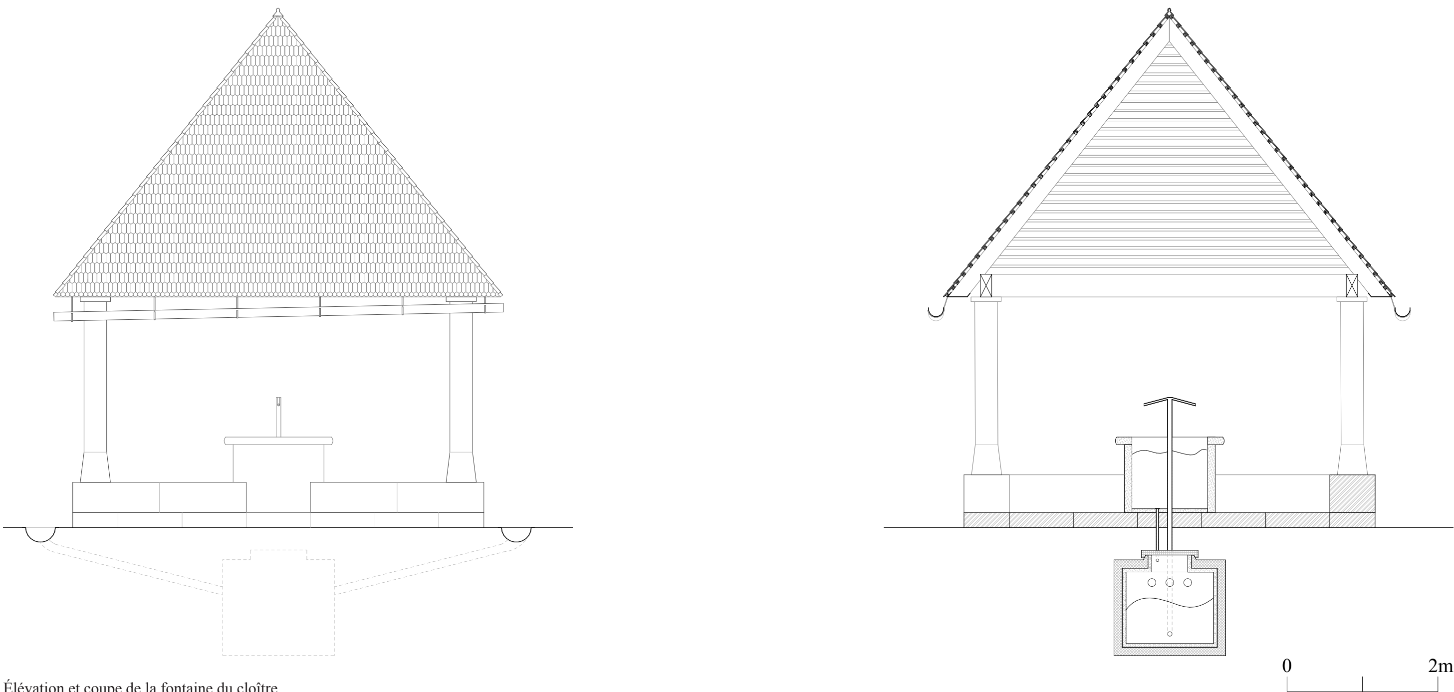
Élévation et coupe de la fontaine du cloître
