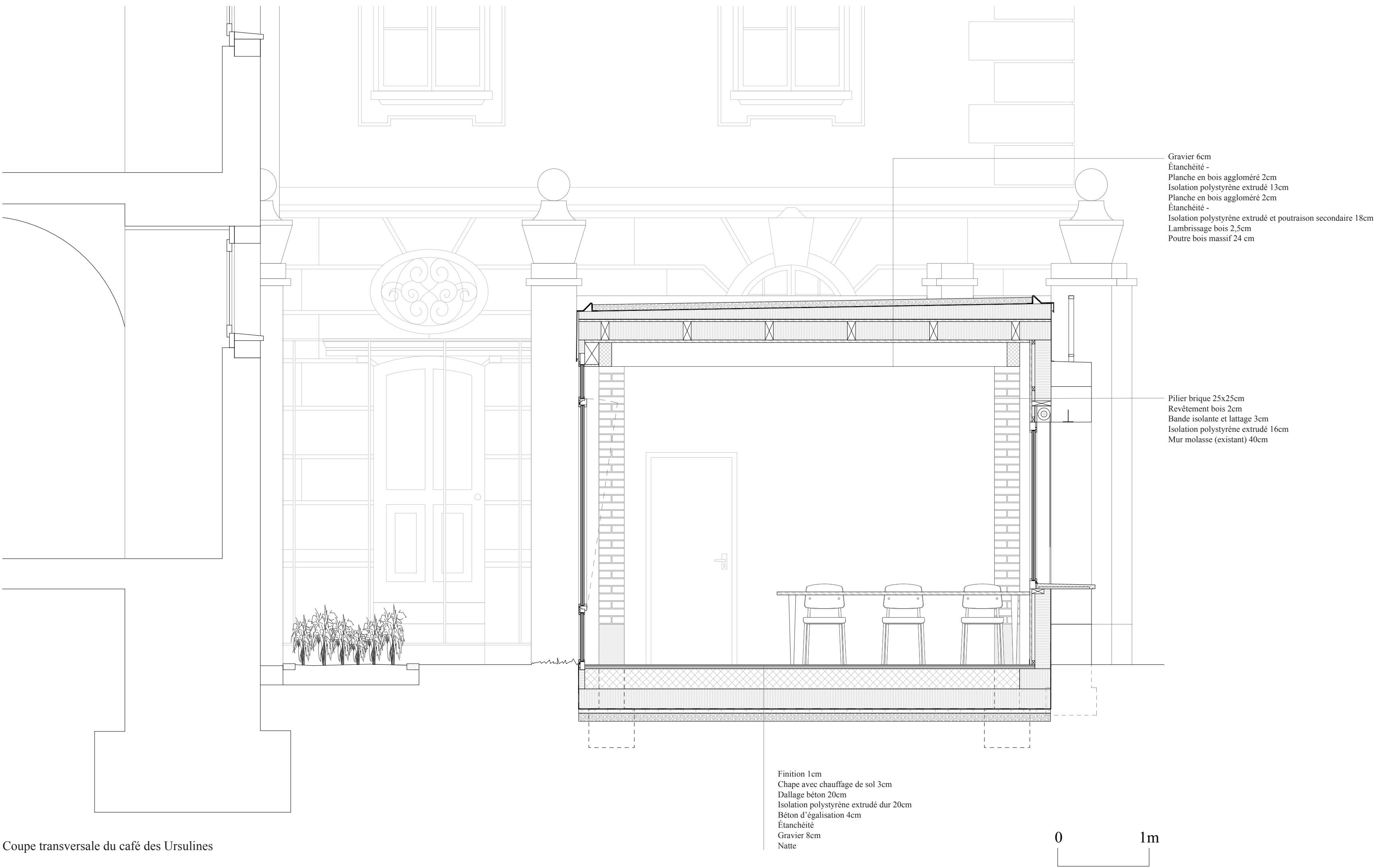
Coupe transversale du café des Ursulines
