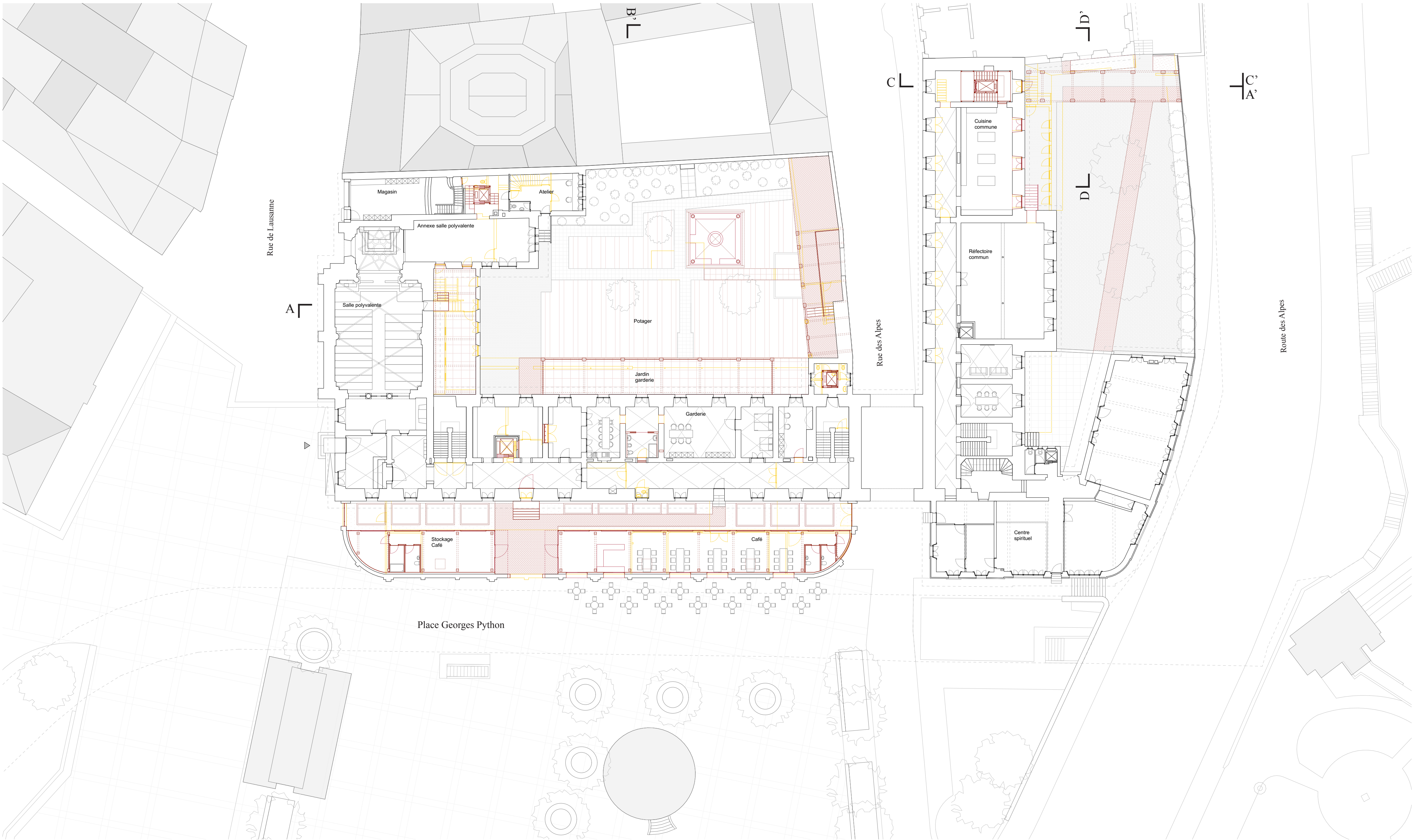
Plan du rez-de-chaussée
