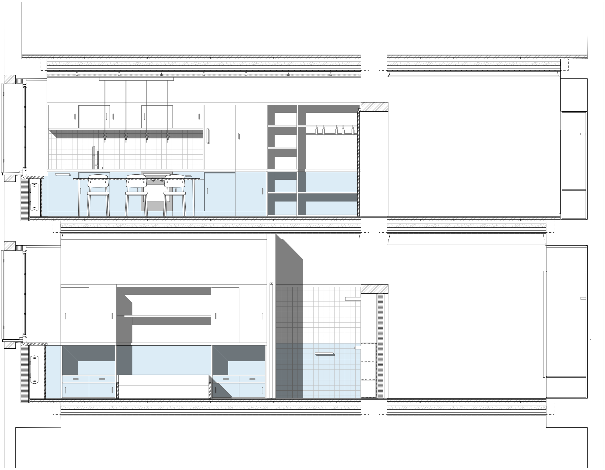
Coupe J-J'
