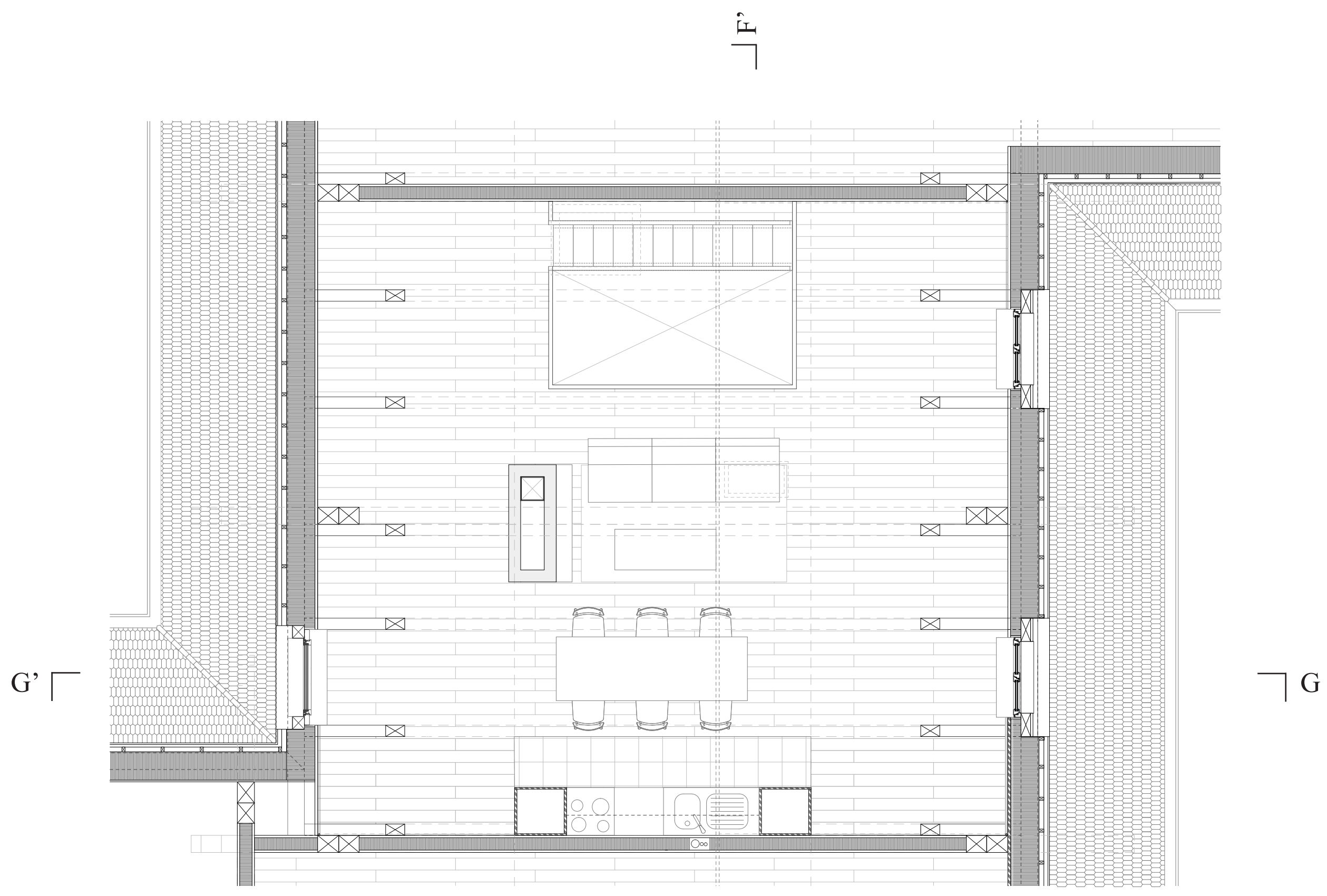
Plan d'un duplex type «combles»
