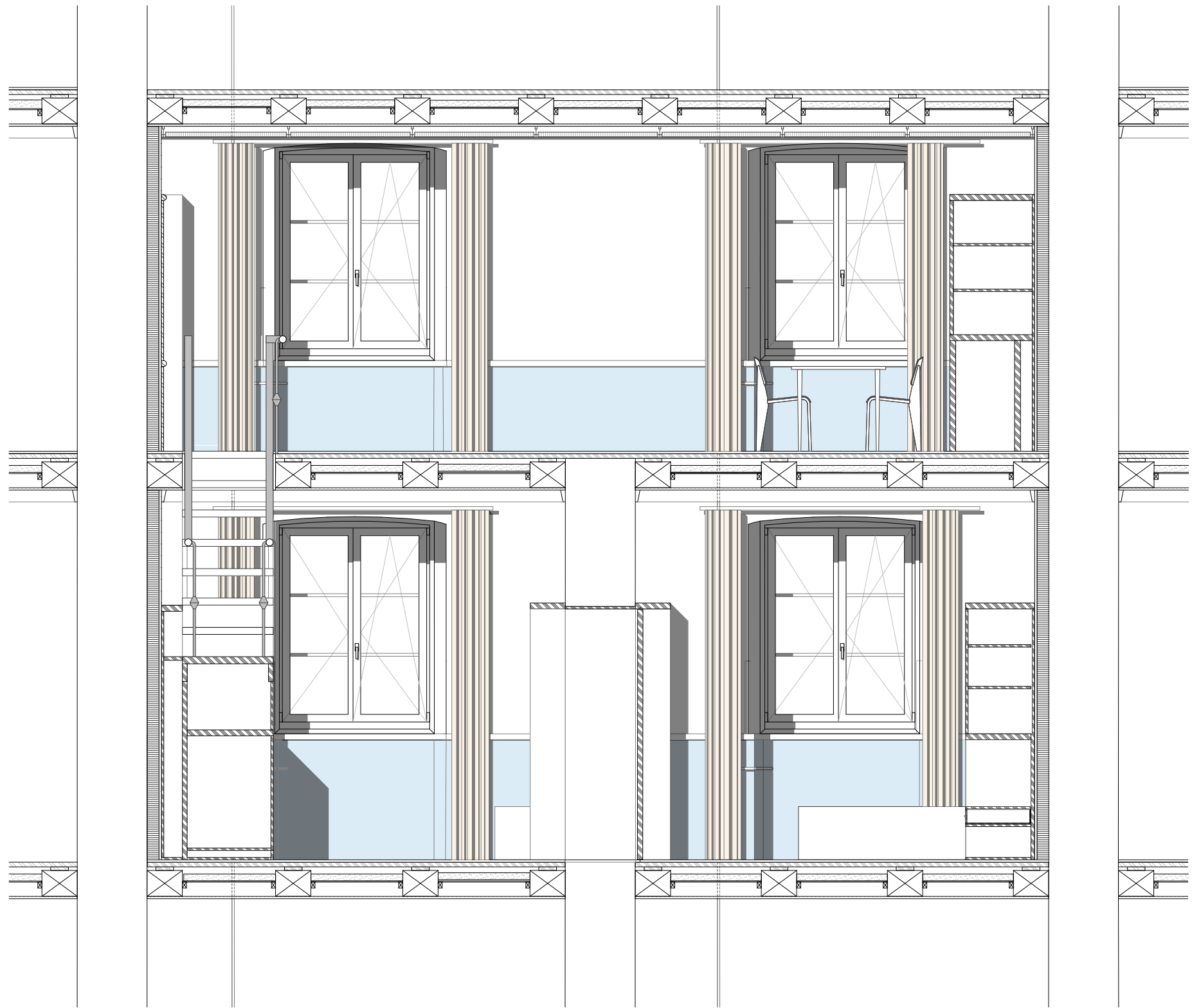
Coupe K-K'
