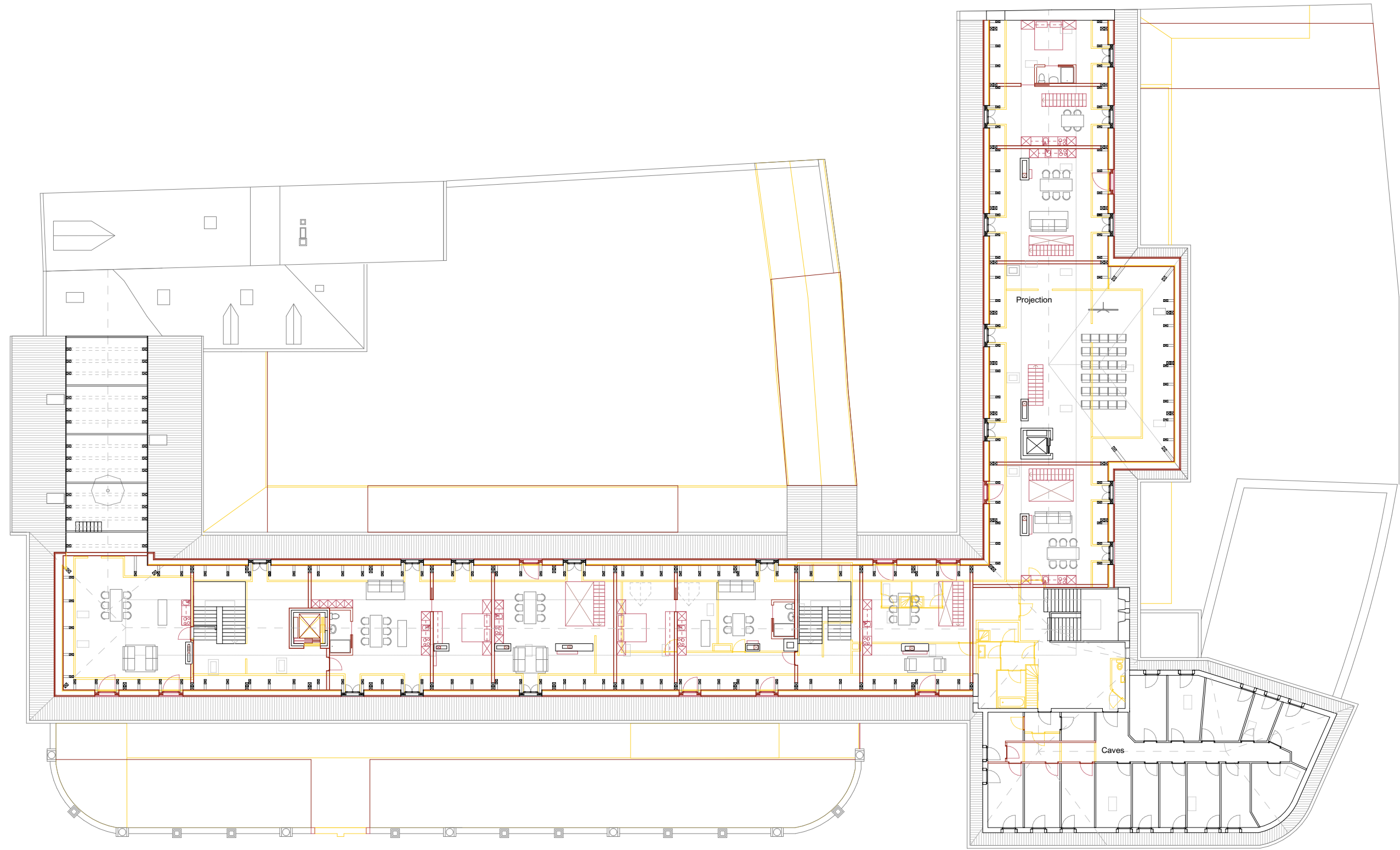
Plan des combles
