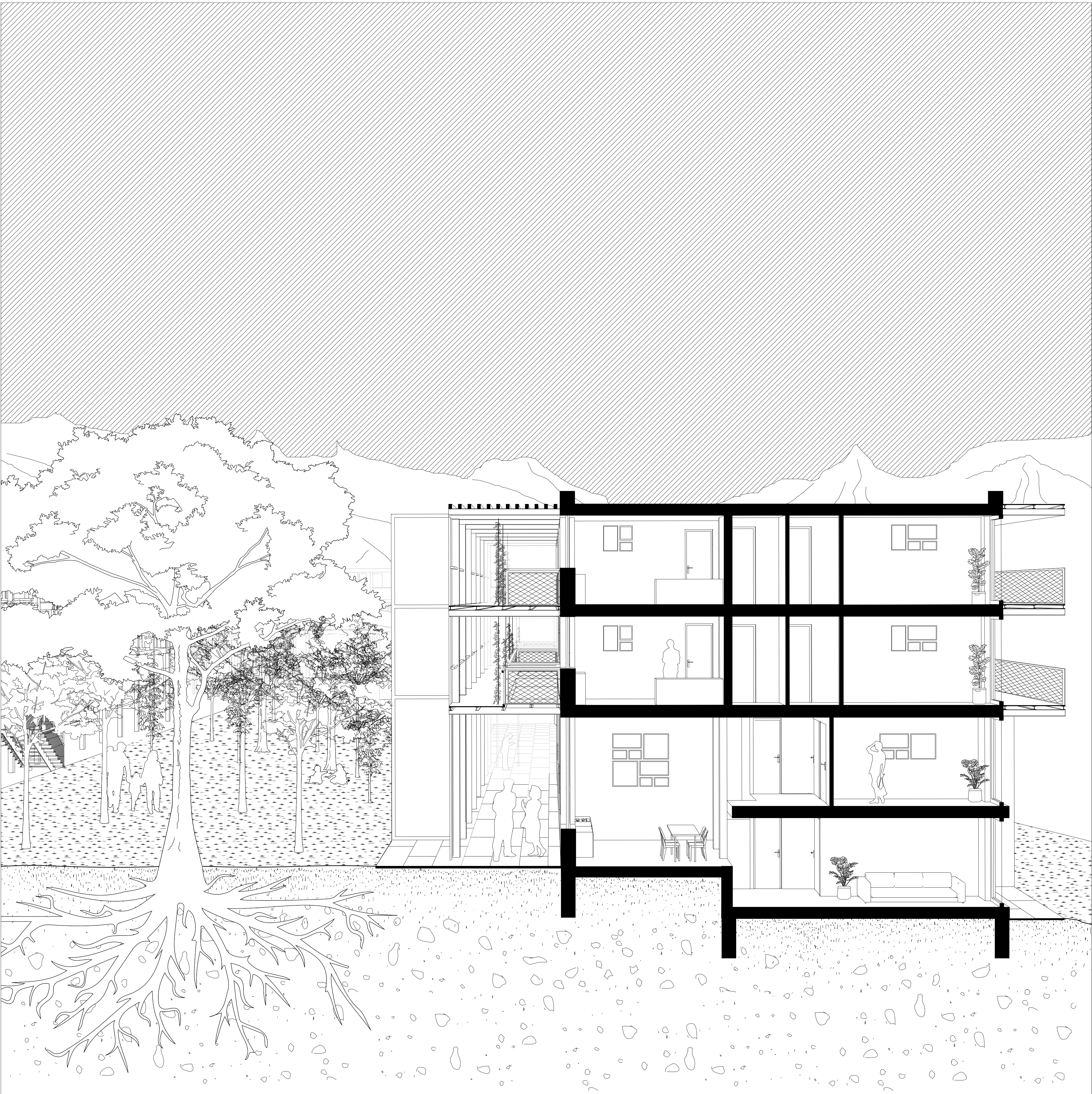
Coupe perspective
