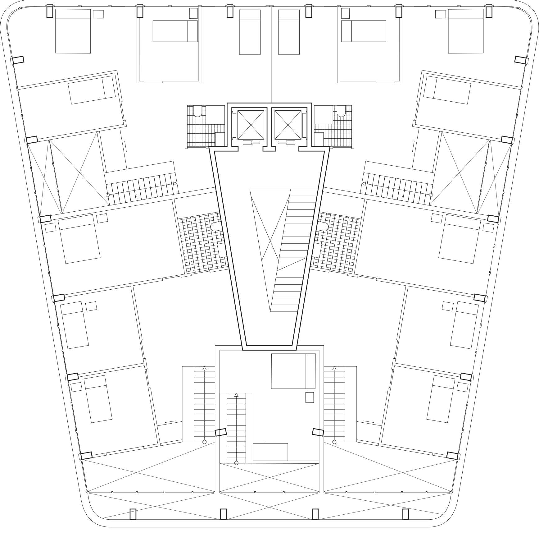
plan typologie duplexe 1:100
