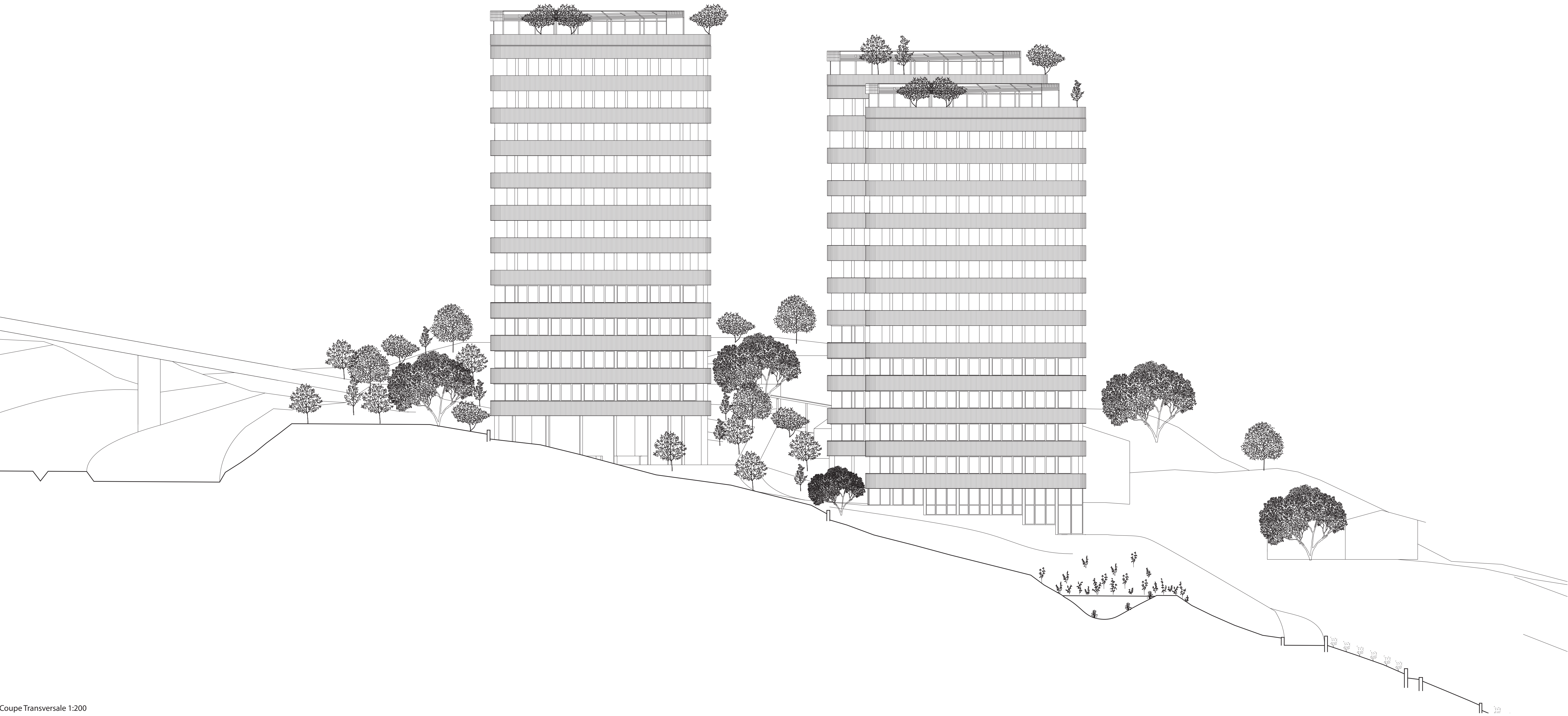
Coupe Transversale 1:200
