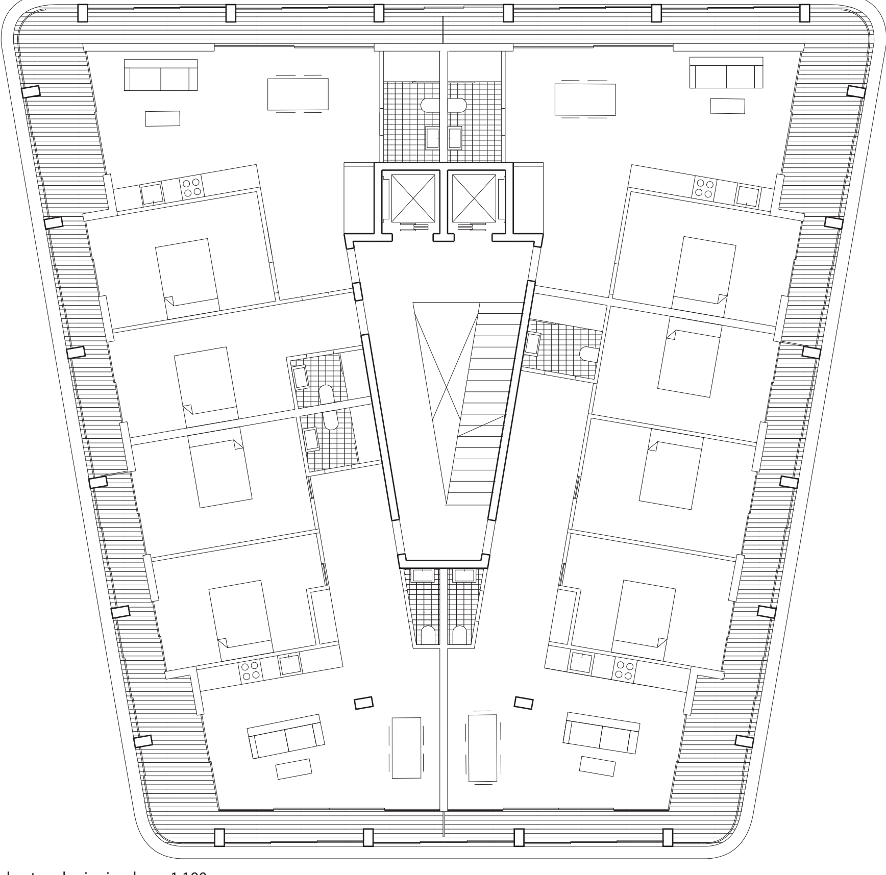
plan typologie simplex 1:100
