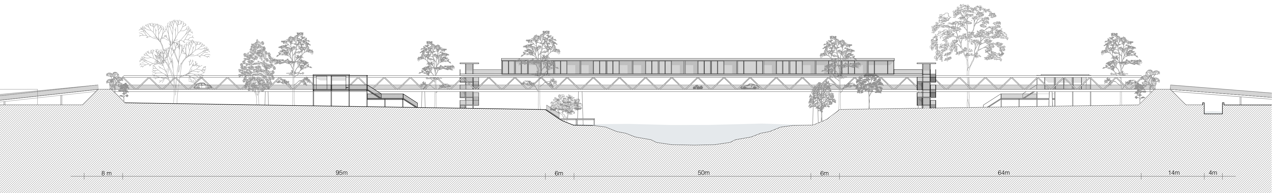
Élévation longitudinale 1:500
