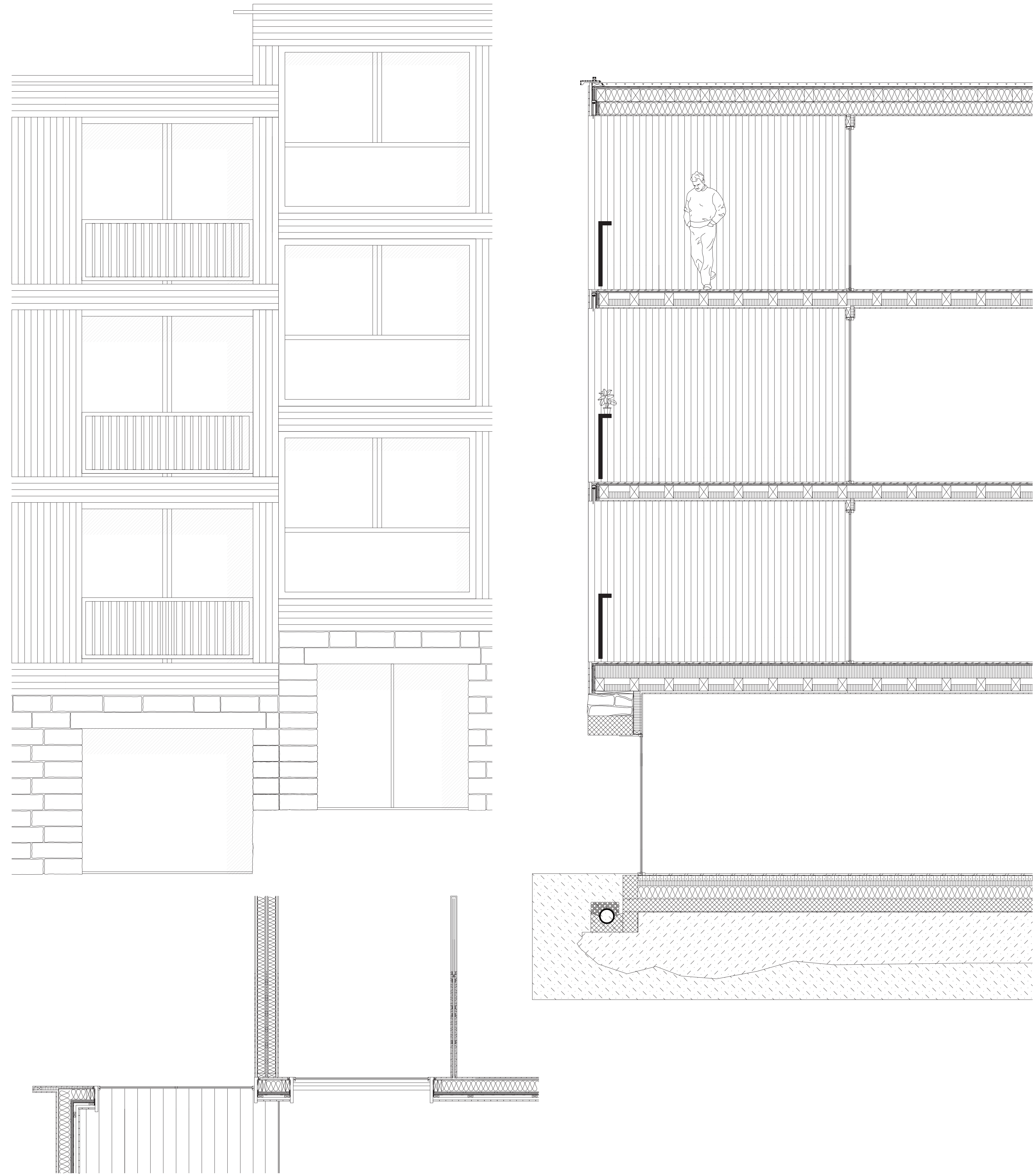
Détail constructif 1:33
