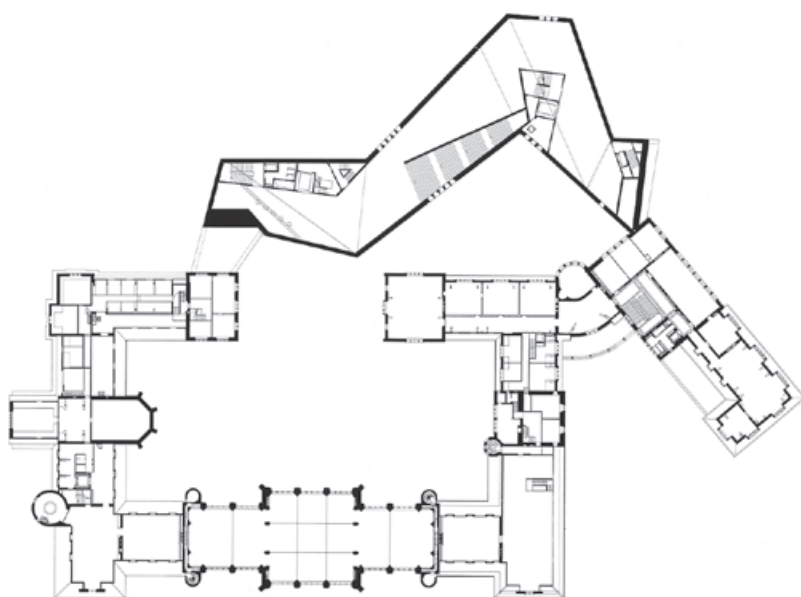
Extension du Kunstmuseum , Zürich, Suisse, 2016 Christ & Gantenbein Emmanuel Christ & Christophe Gantenbein Plan
