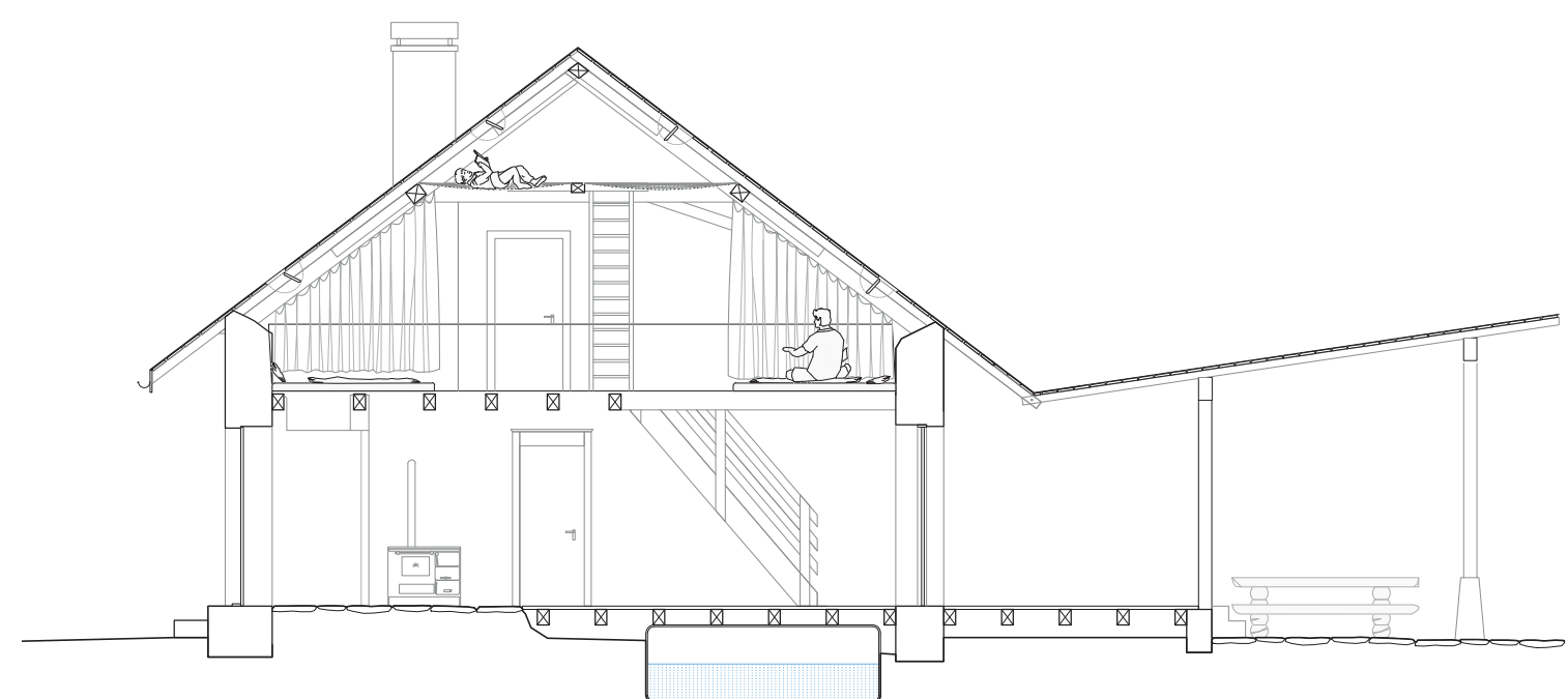
Coupe nord-sud, 1:100
