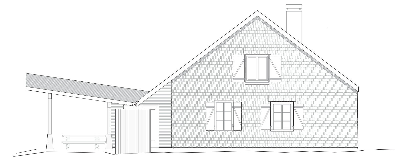
Façade ouest, 1:100
