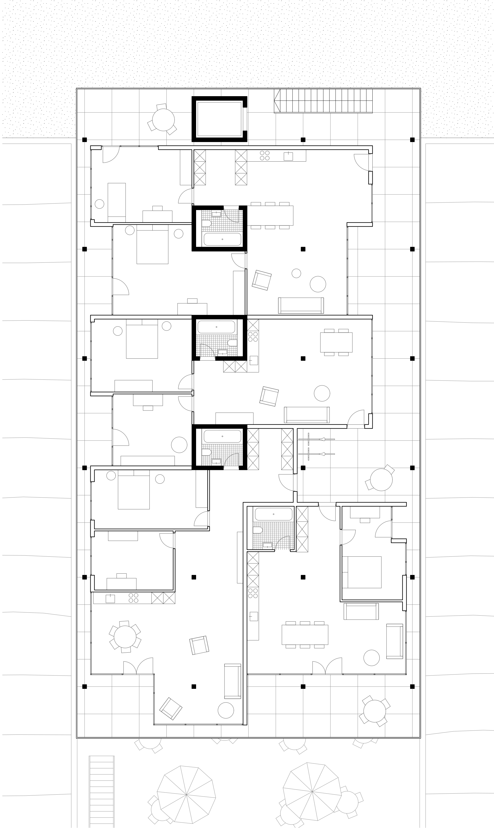
Plan étage 2 1:100
