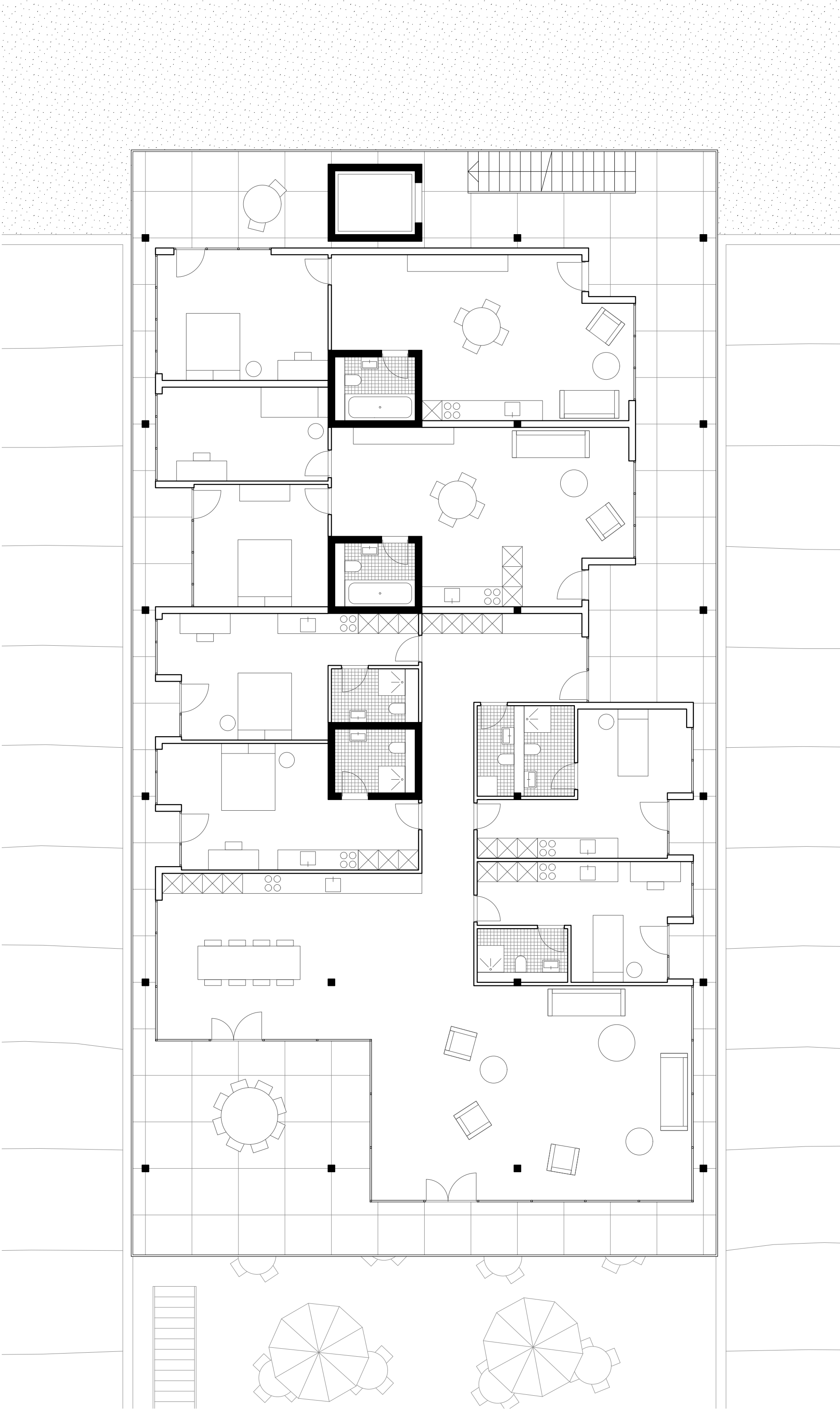
Plan étage 1 1:100
