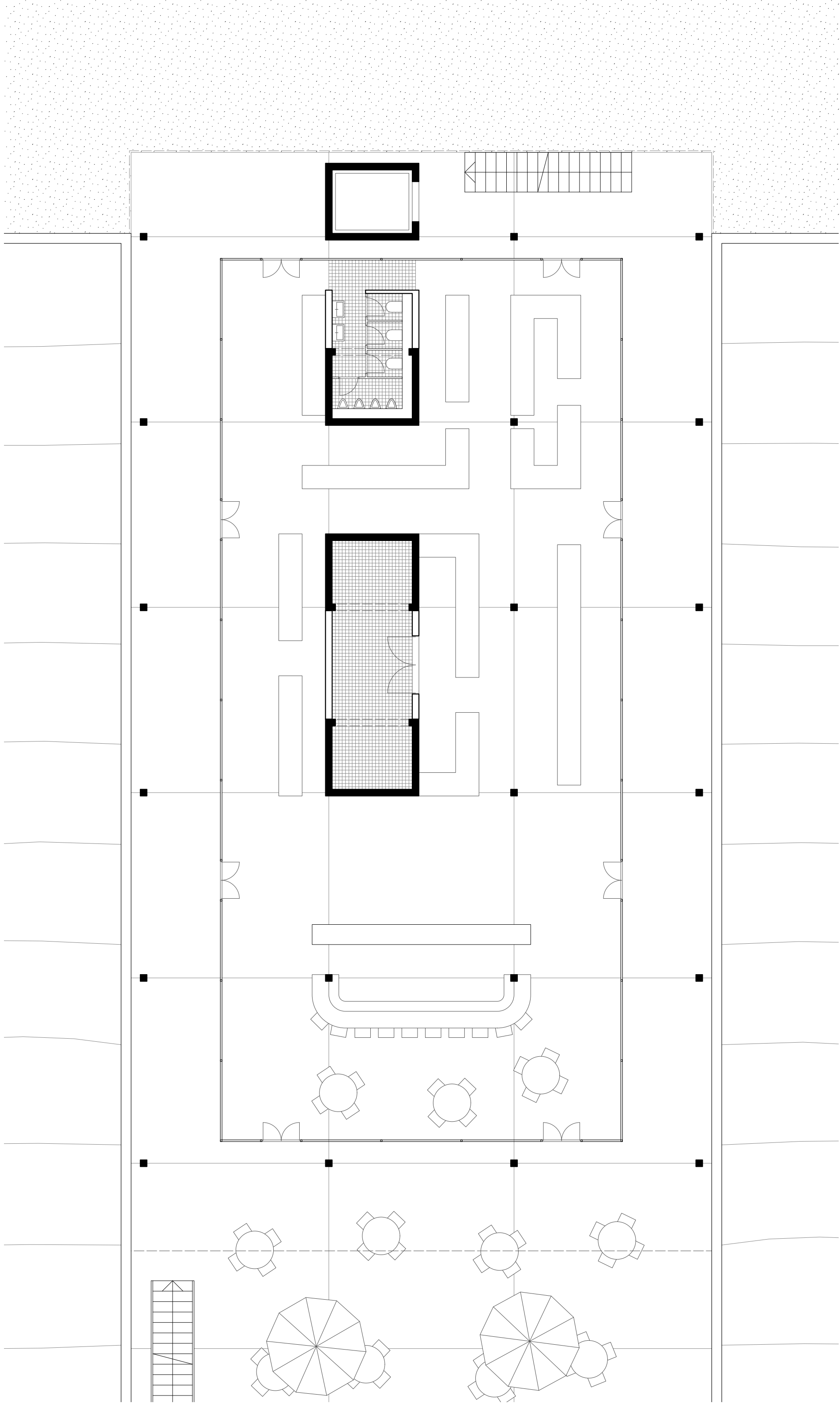
Plan rez 1:100
