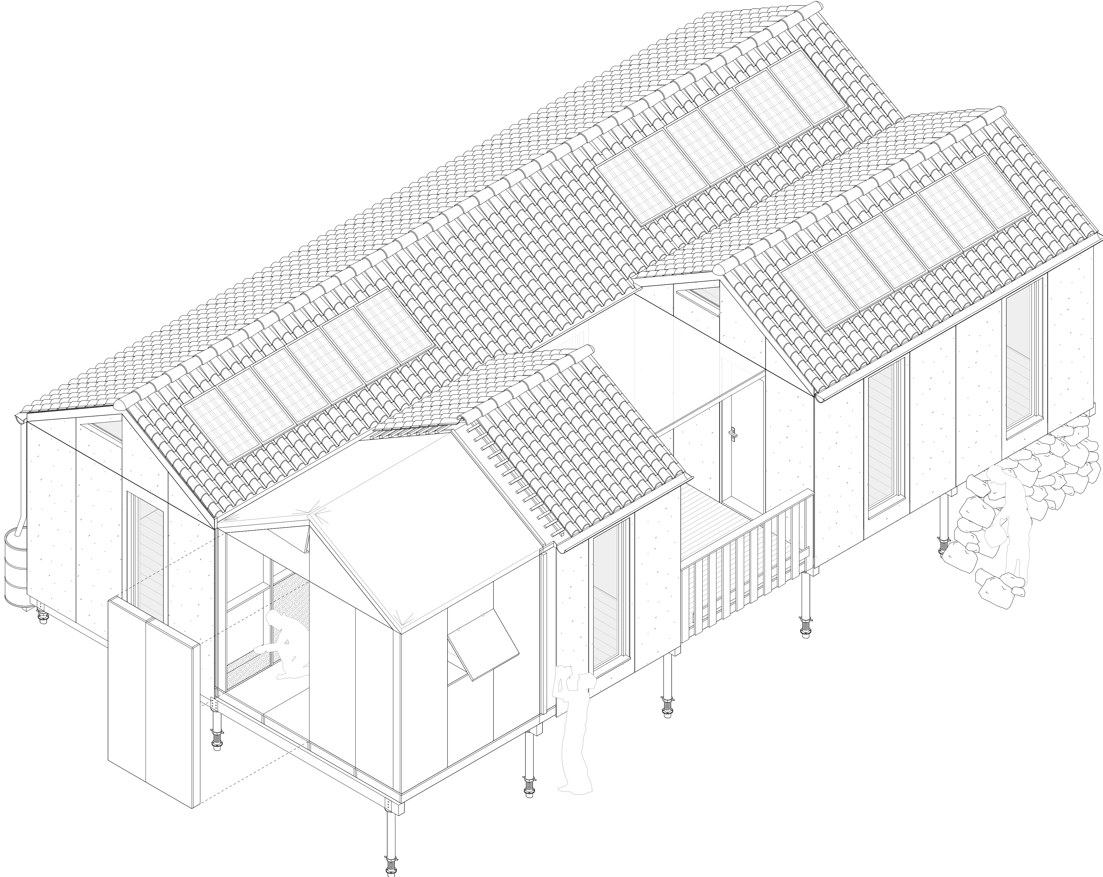
Axonométrie isométrique _Permanent 1:33
