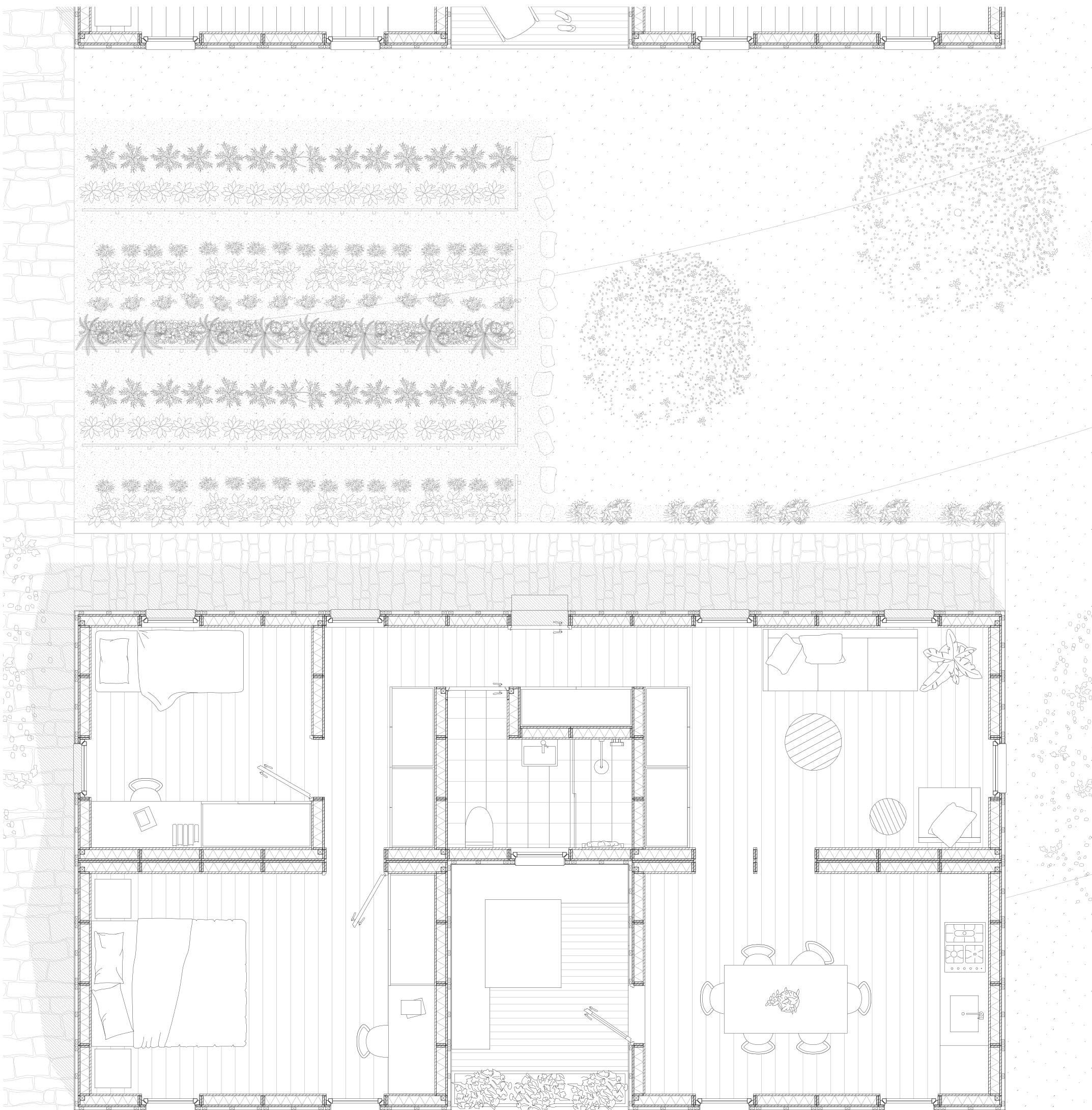
Plan faible pente _Permanent 1:33
