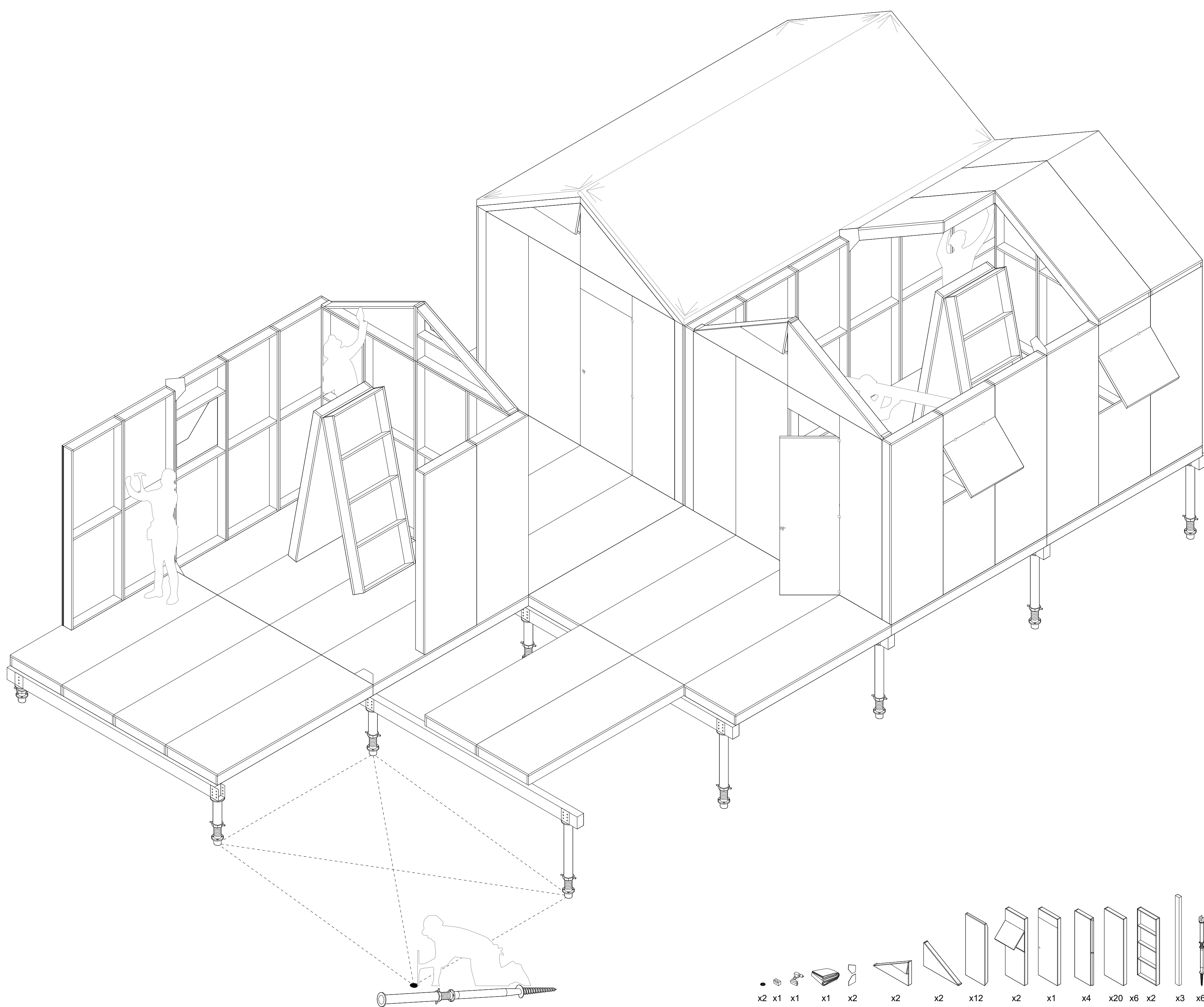
Axonométrie isométrique _Urgence 1:33
