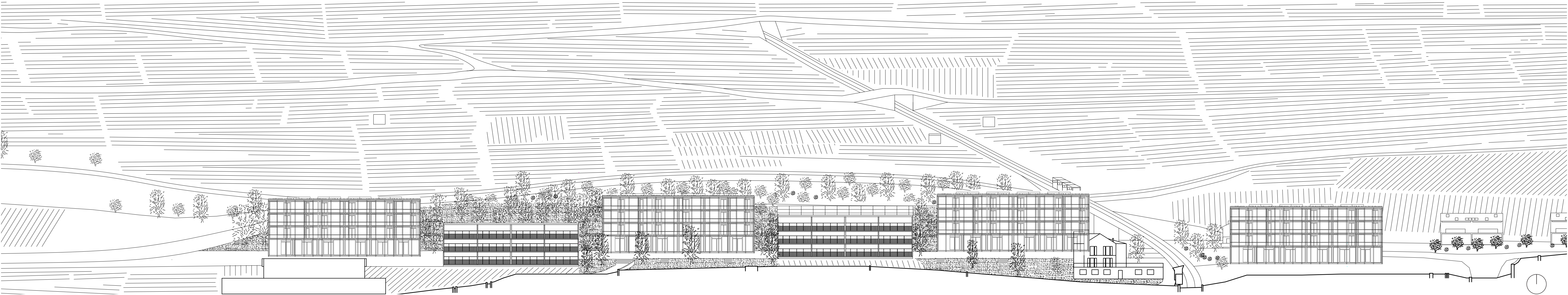
Coupes longitudinale Nord 1:500
