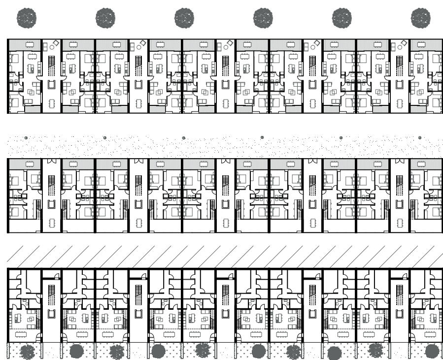
PLAN APPARTEMENTS BATIMENT COTE RHONE 1:200, DE BAS EN HAUT: REZ INFERIEUR, REZ SUPERIEUR, ETAGE TYPE
