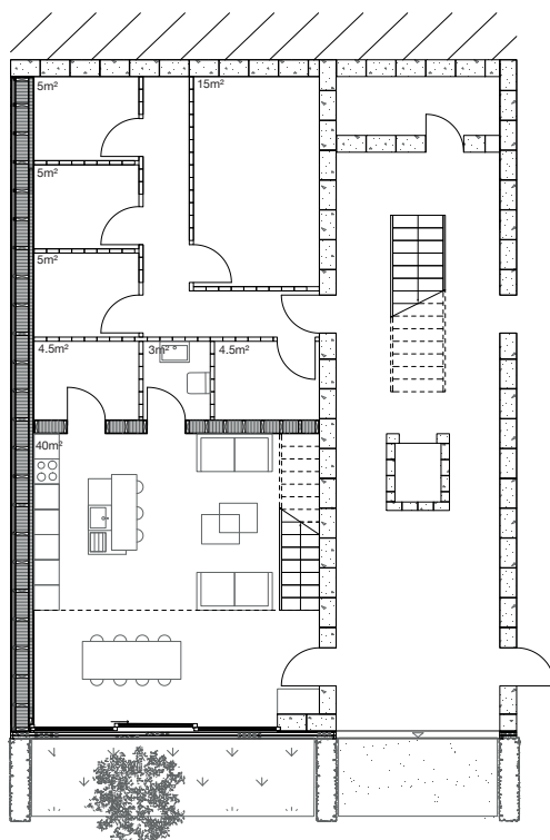
PLAN APPARTEMENTS BATIMENT CTE RHONE 1:50, HAUT: ETAGE TYPE, BAS GAUCHE: REZ INFERIEUR, BAS DROITE: REZ SUPERIEUR
