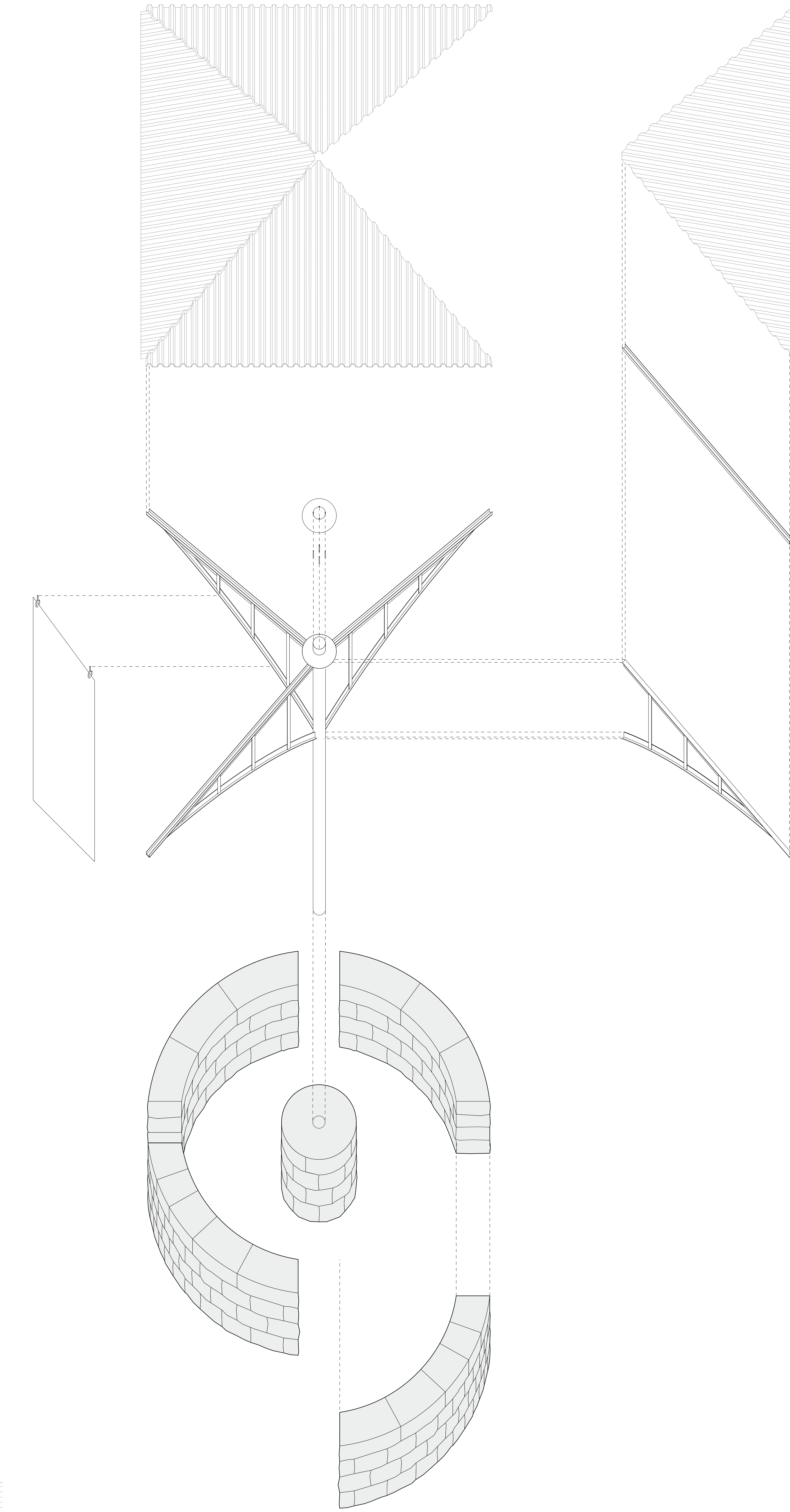
Axonométrie de principe
