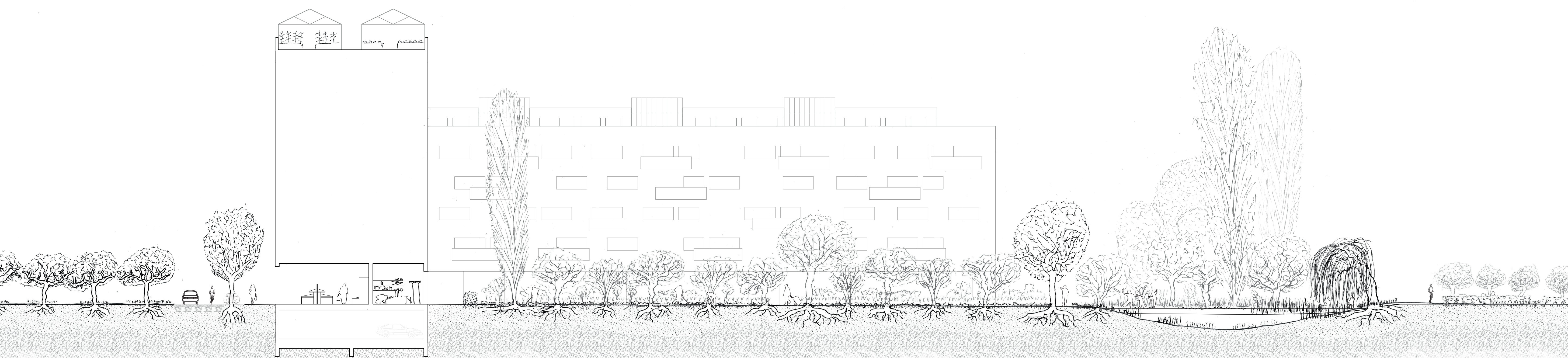
Cours agricoles - Coupe longitudinale - 1:200
