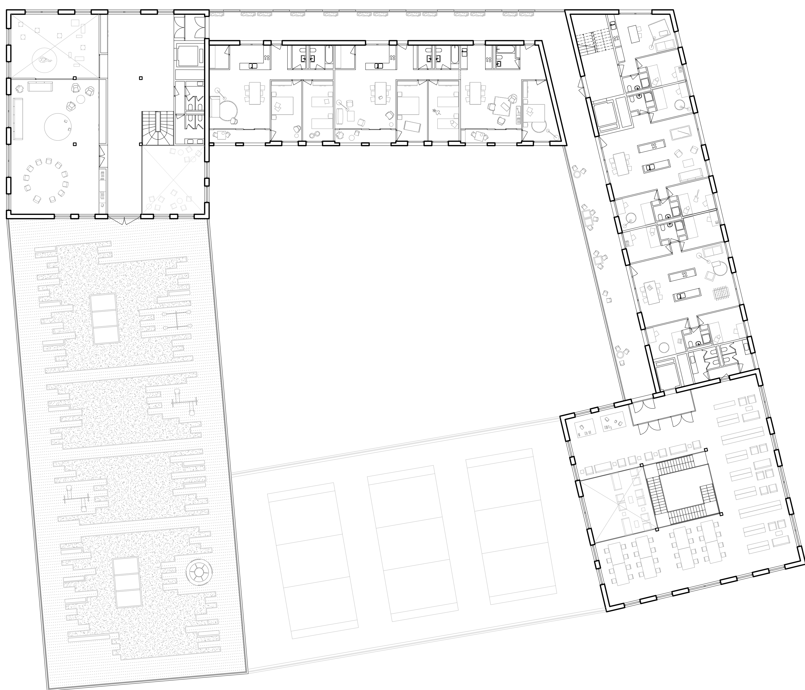
- PLAN ETAGE 3 | 1:200 -
