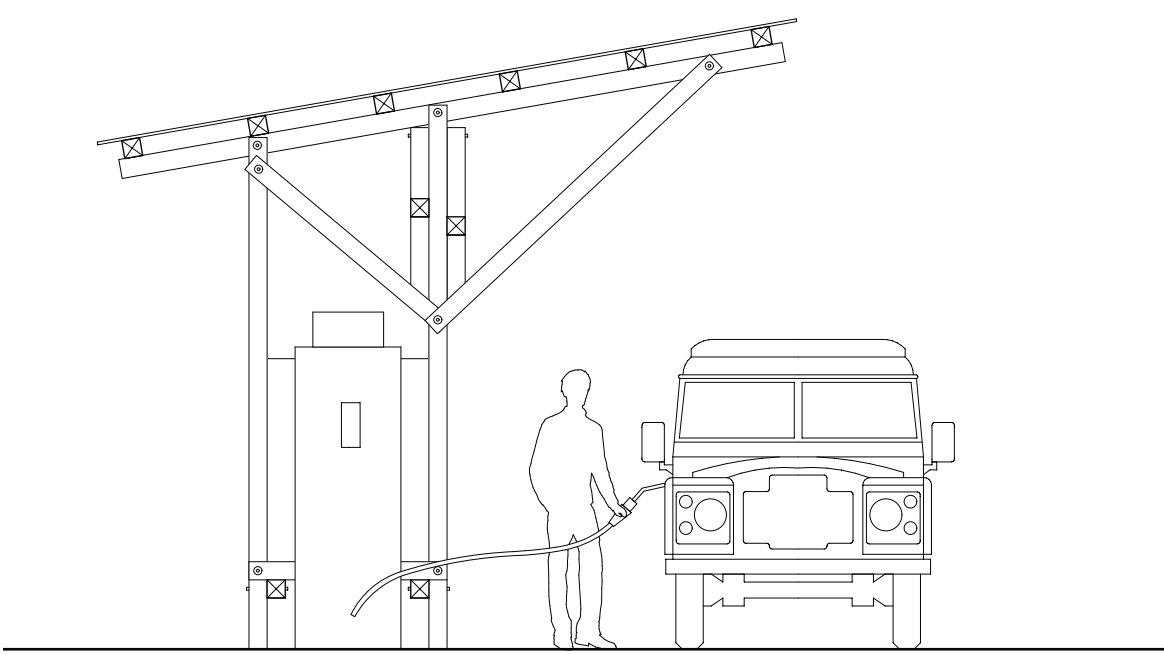
Coupe BB 1:50
