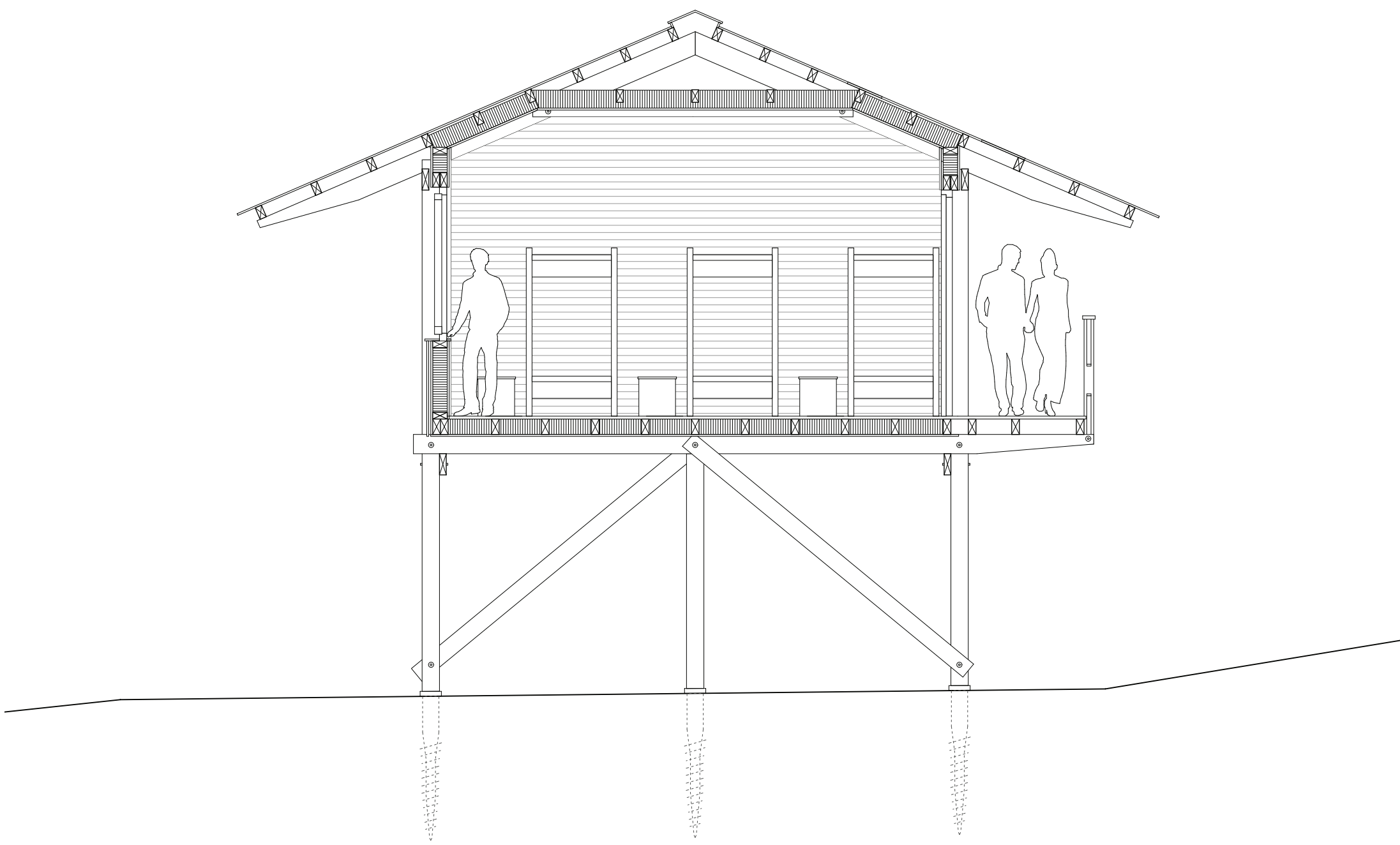
Coupe DD 1:50
