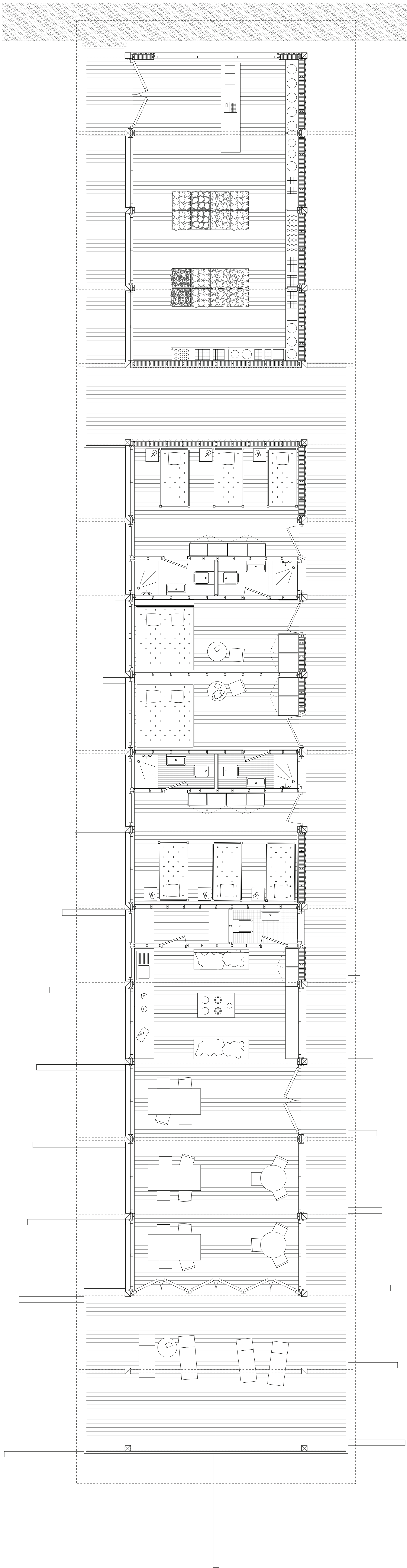
Plan Auberge - Echoppe 1:50
