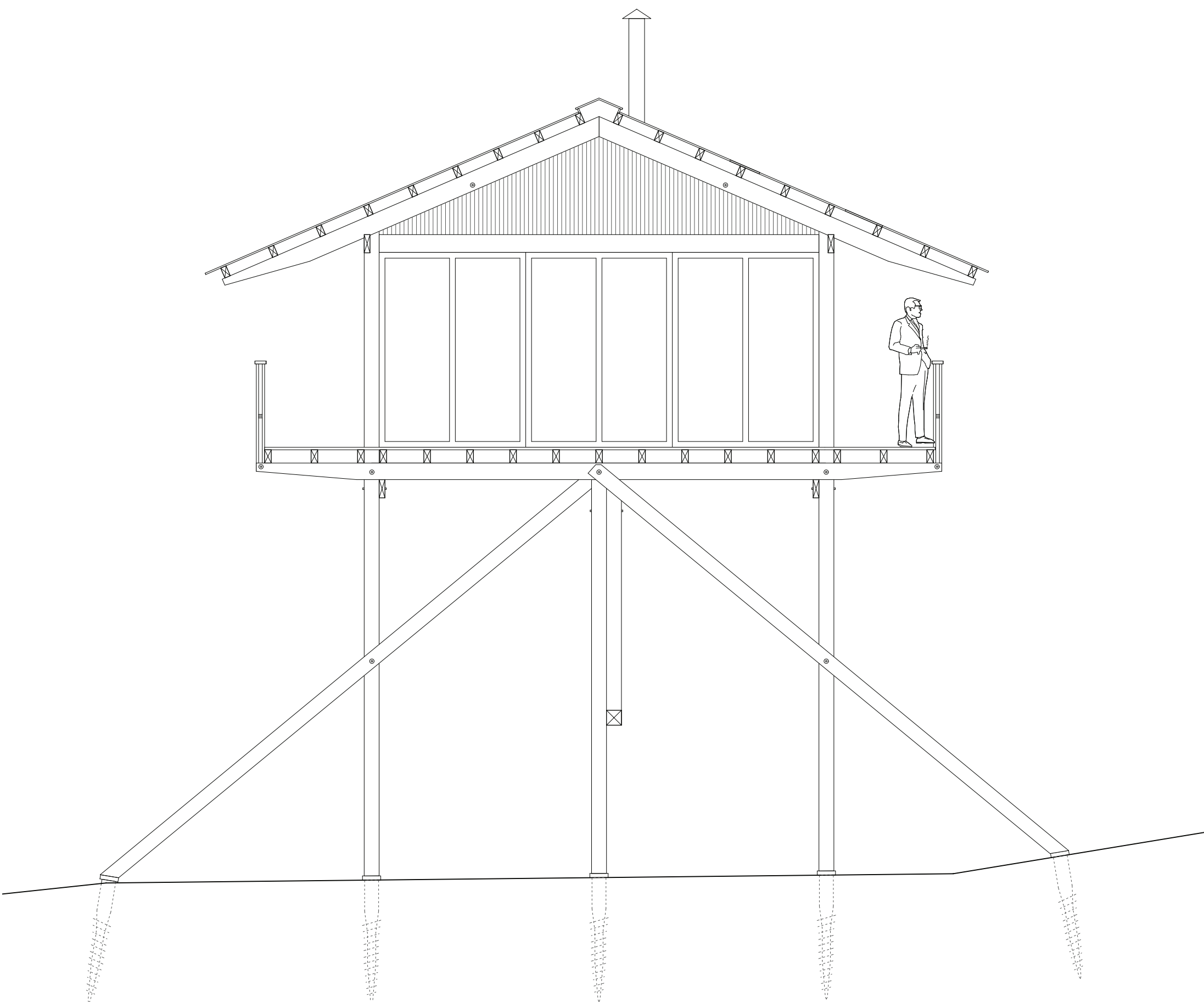
Coupe EE 1:50
