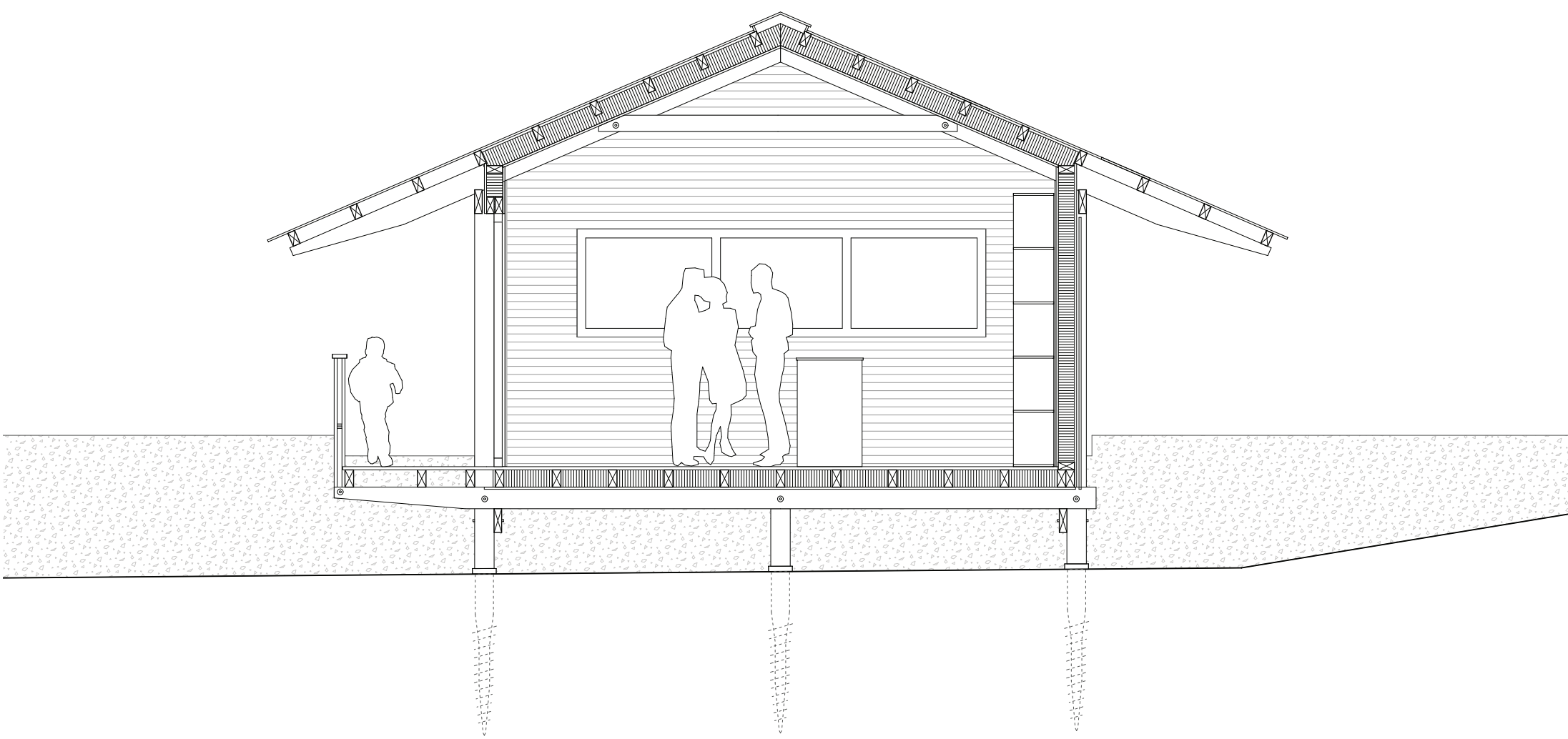
Coupe CC 1:50
