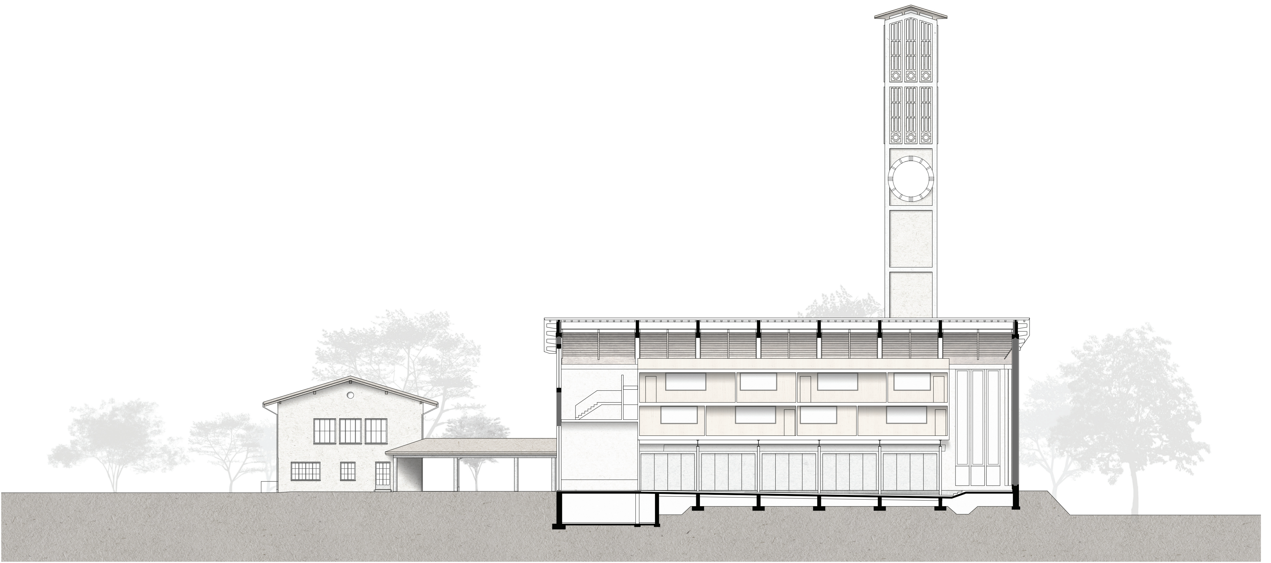
Coupe BB' 1:200
