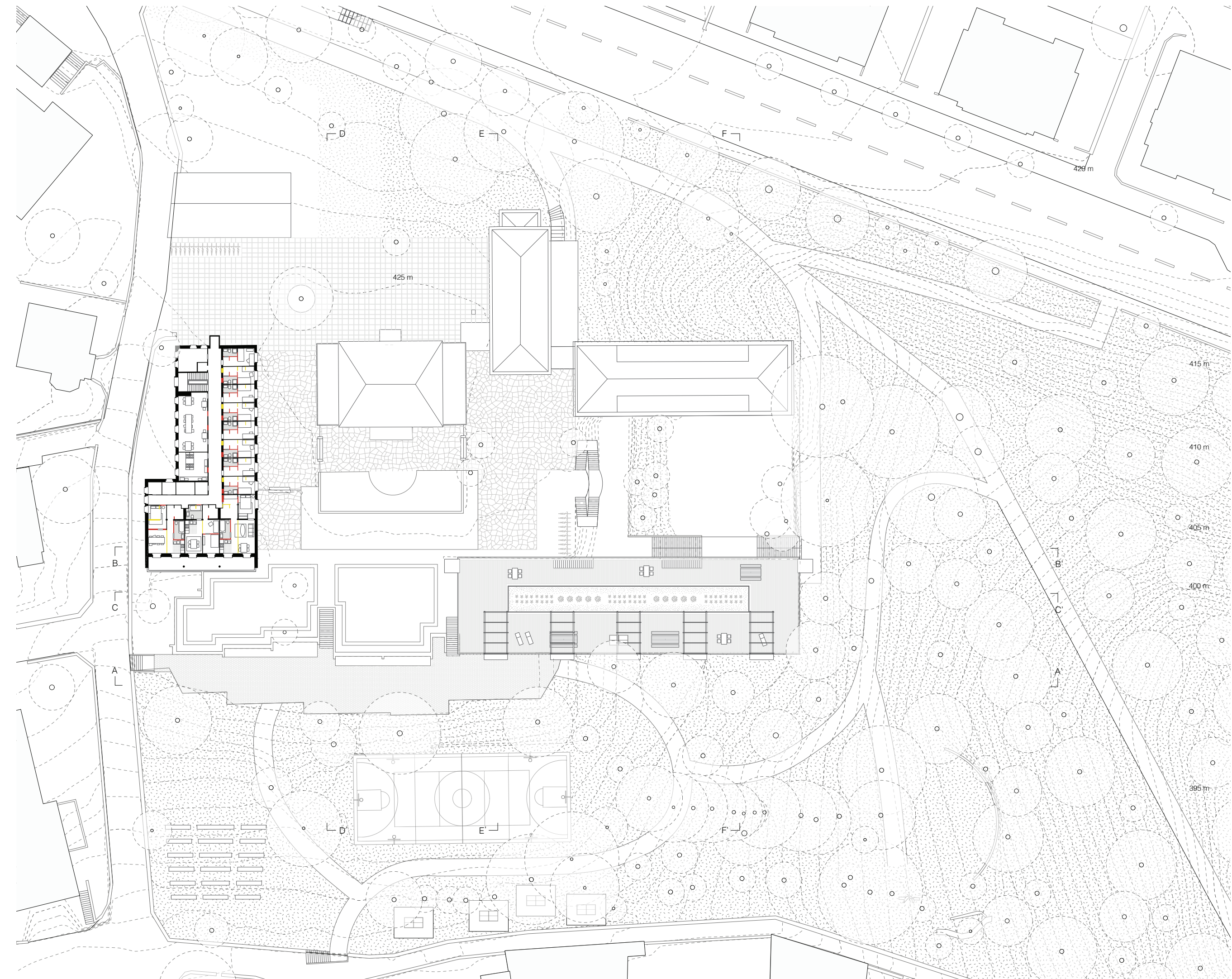
Plan site - Niveau 3
