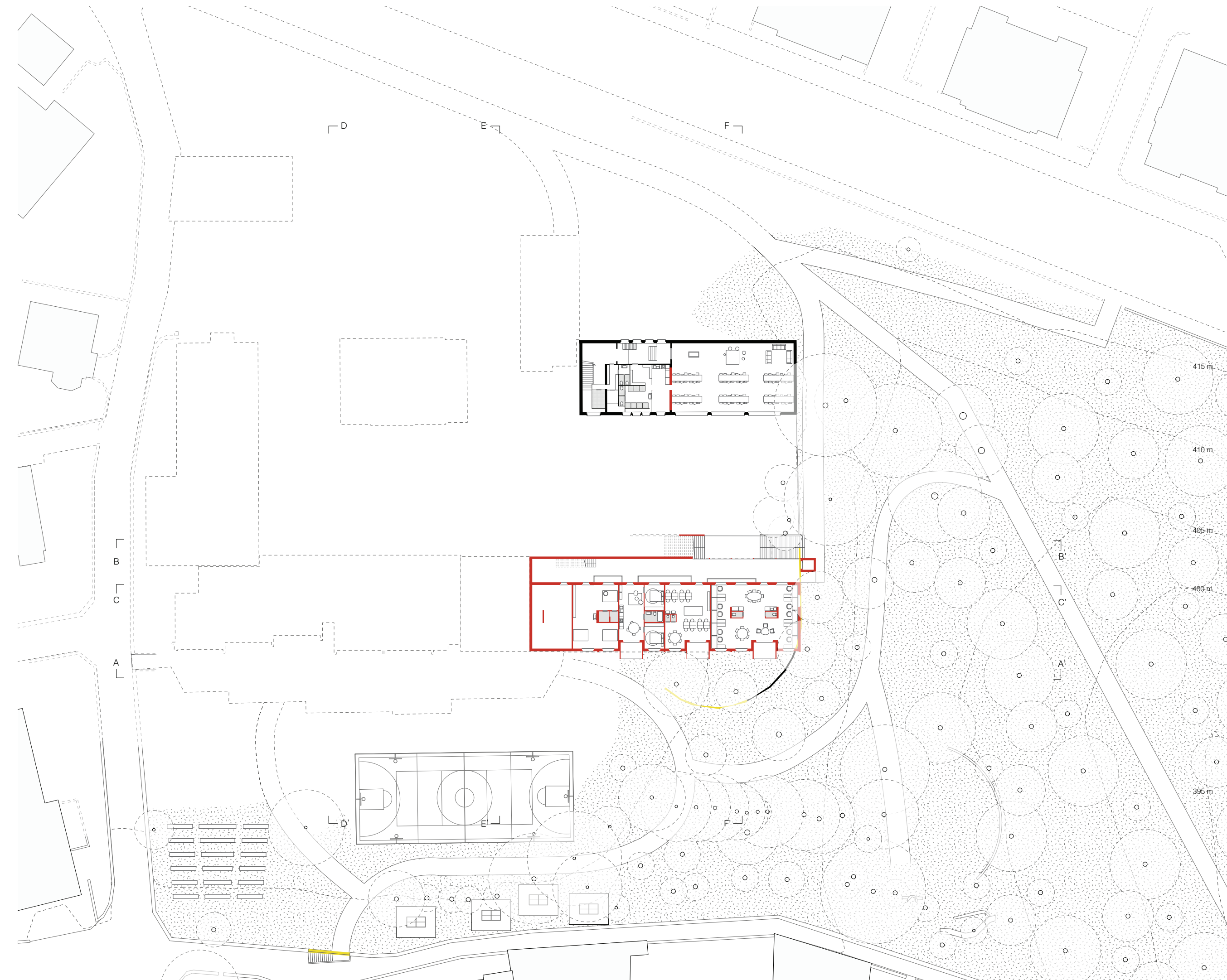
Plan site - Niveau -2
