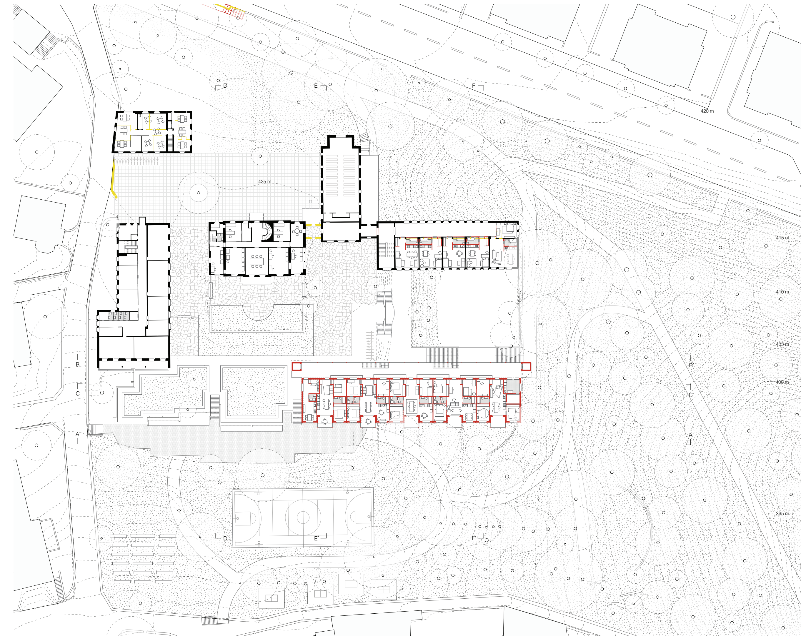
Plan site - Niveau 1
