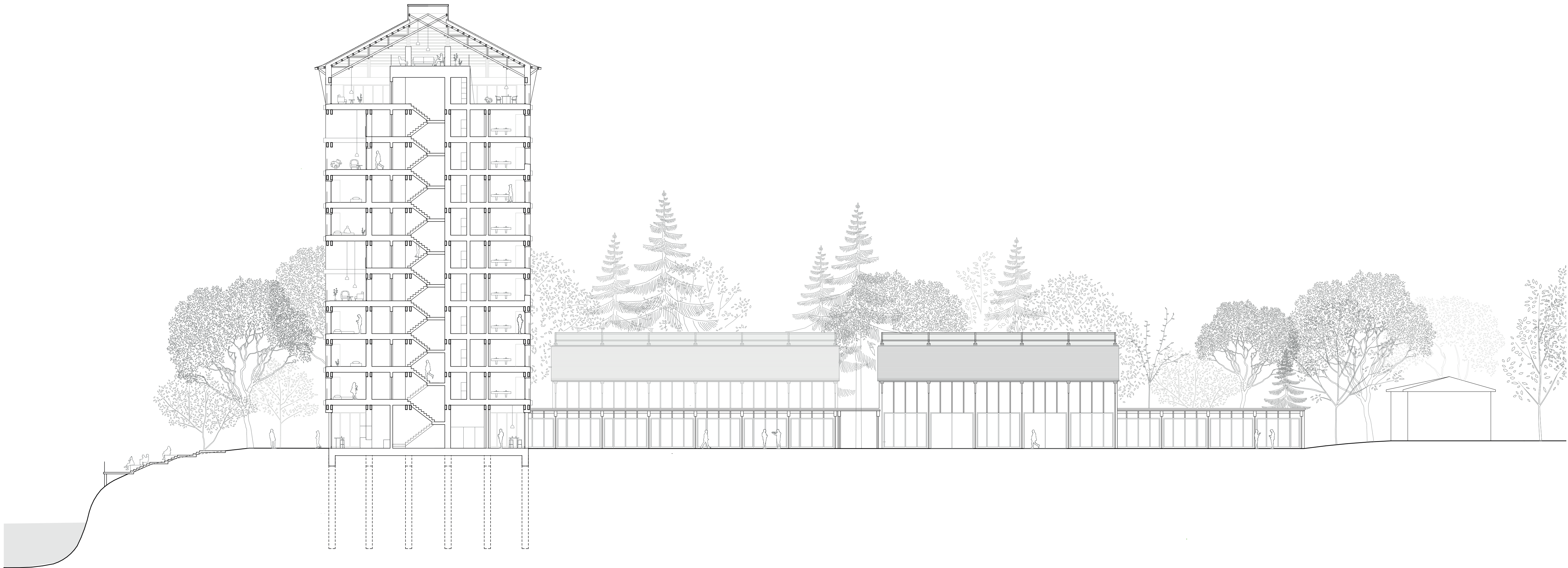
LONGITUDINAL SECTION BB'
