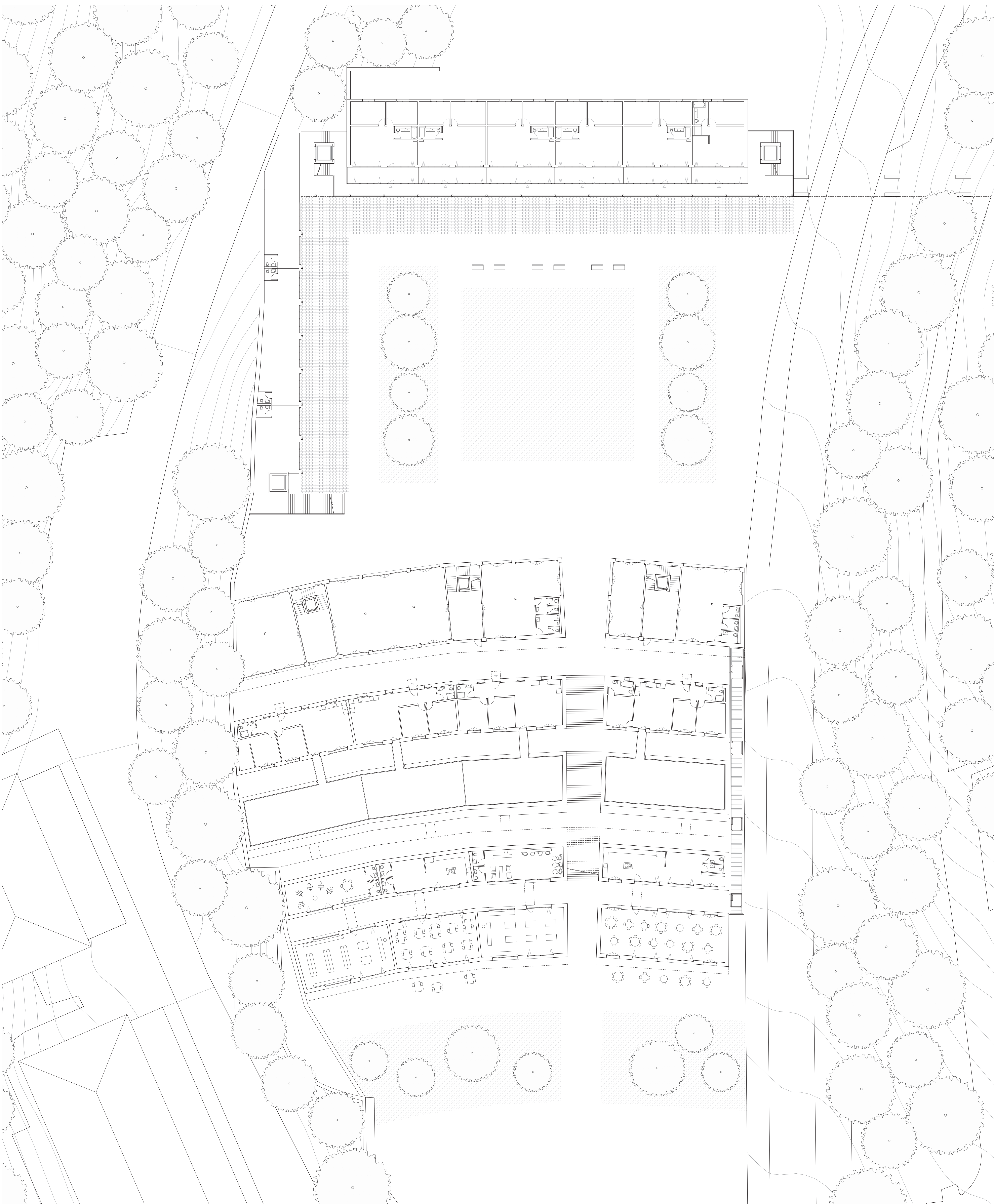
Plan du rez-de-chaussée 1:200
