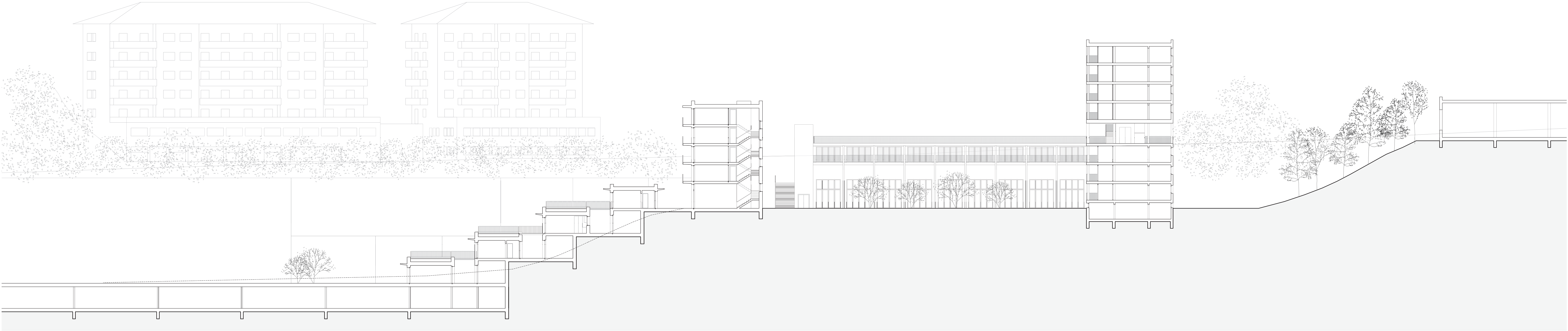
Coupe transversale 1:200
