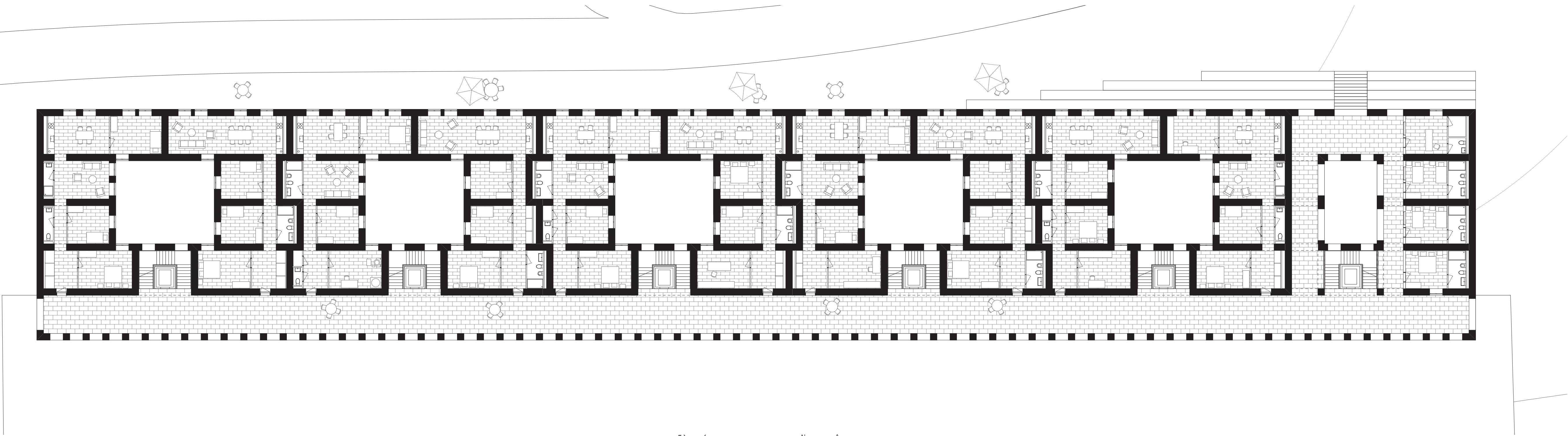
5ème étage, appartements-ateliers et gîte
