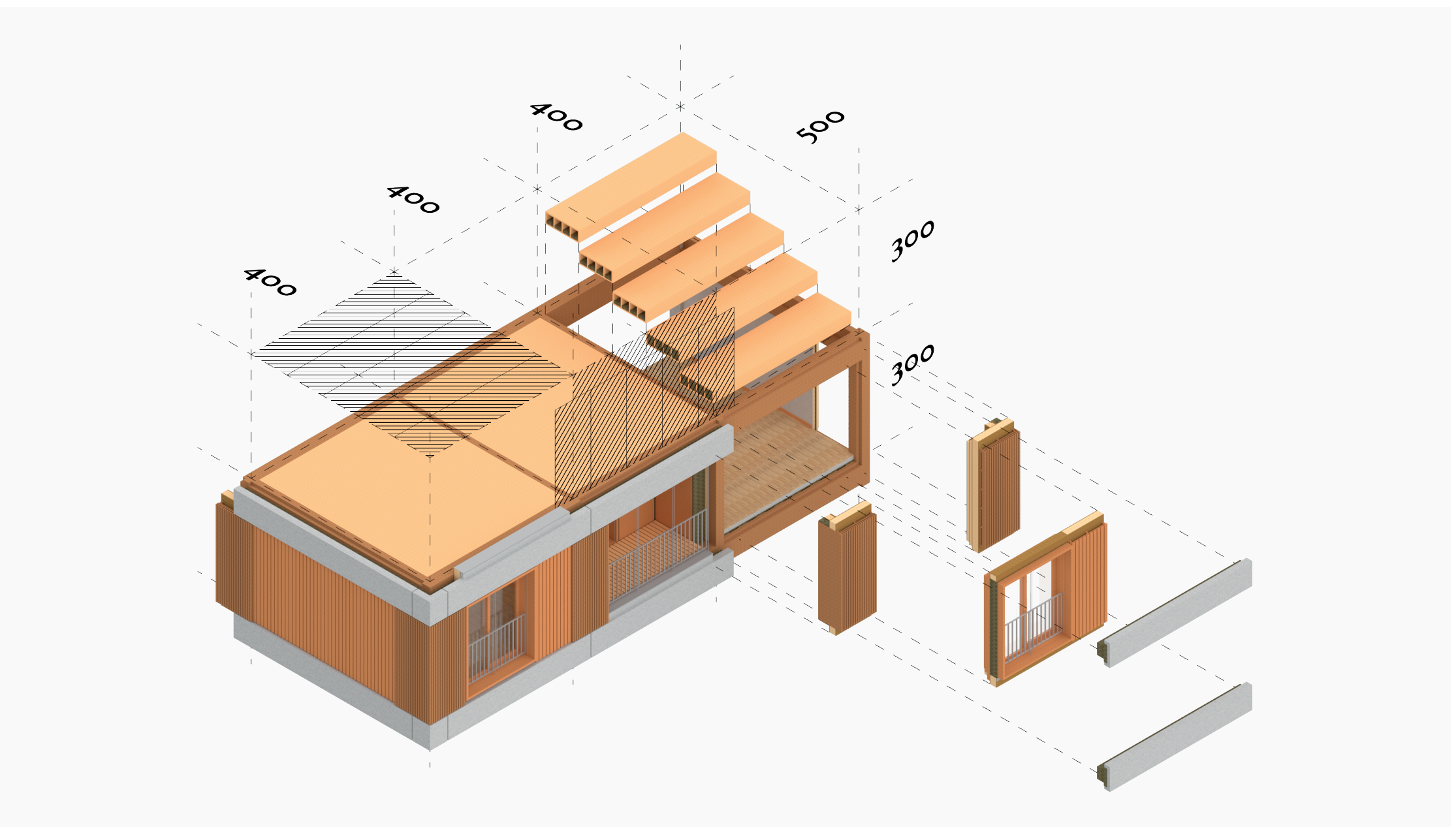
schéma 4 - modules
