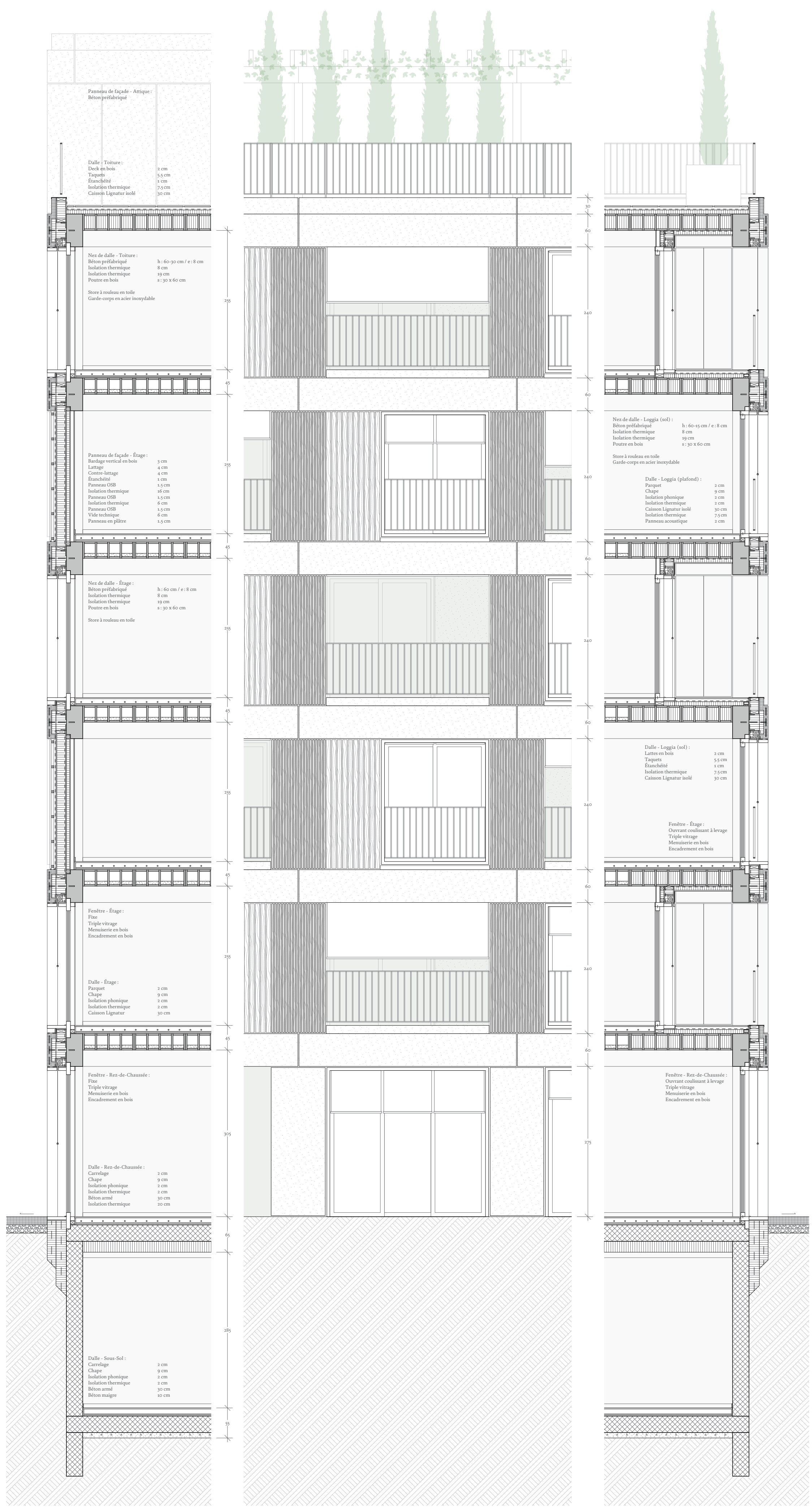
coupe constructive - façade nord-est - 1:50
