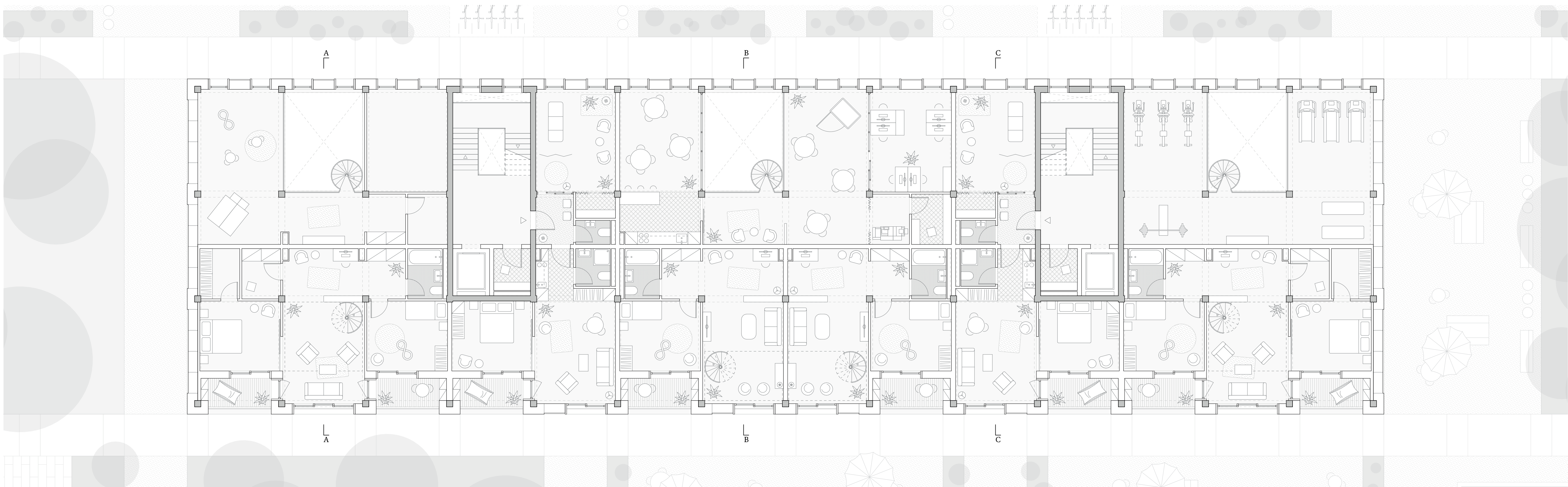
plan étage 1 - 1:100
