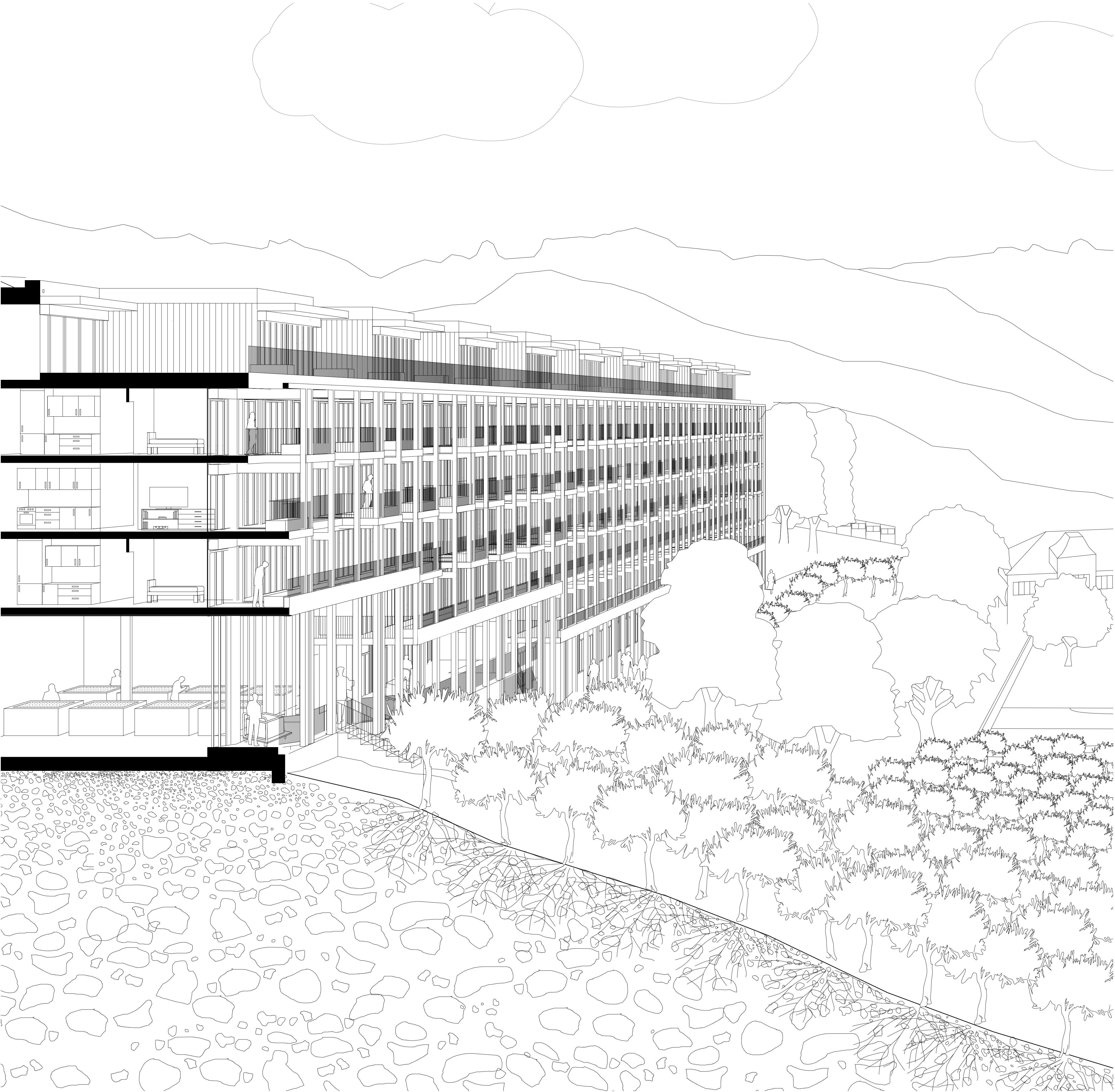
Coupe perspective
