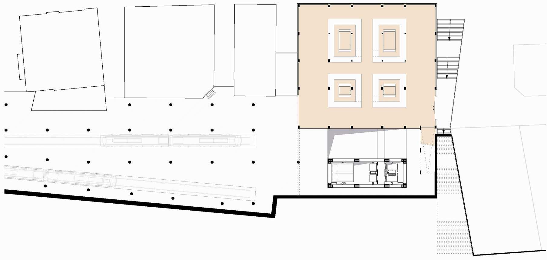
Plan Niveau -7 1 / 500
