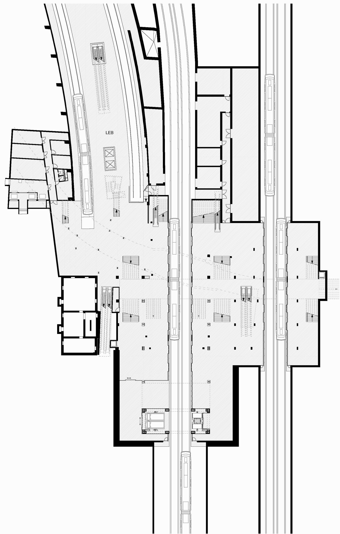
Plan Niveau Métro M2/M3/LEB 1 / 500
