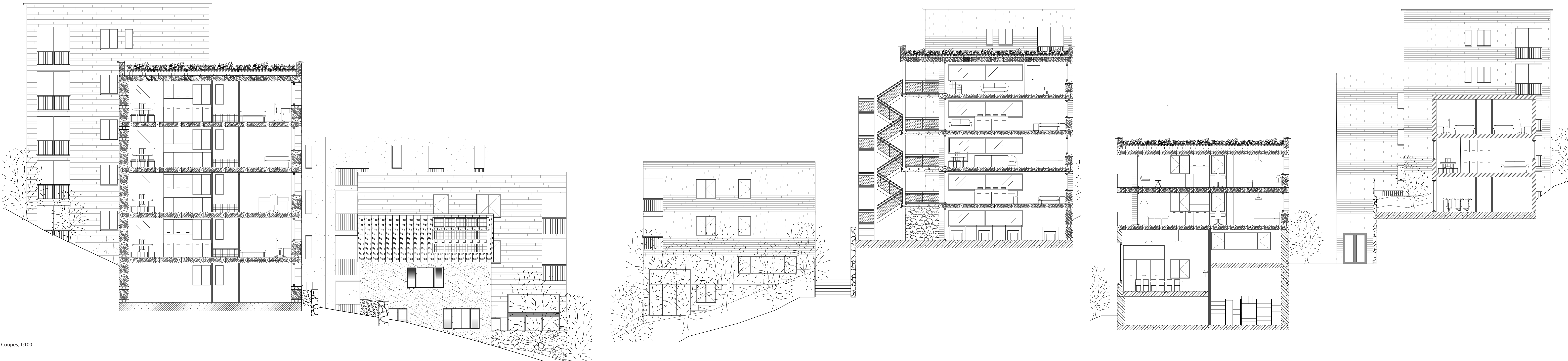
Coupe longitudinale, 1:100
